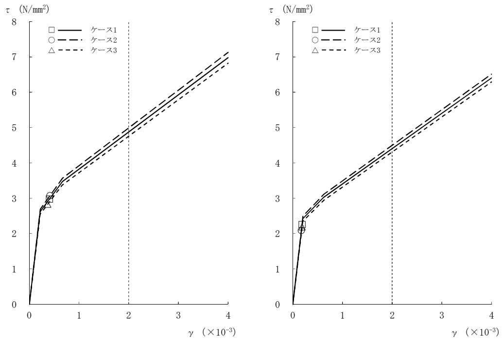
図2-18 τ - γ 関係と最大応答値 (Ss-1, NS方向, B1F) (6/8)
