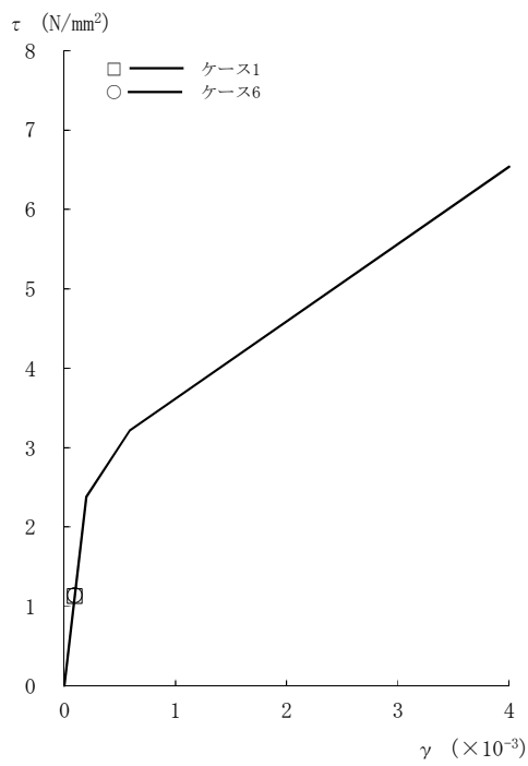
図2-116 τ - γ 関係と最大応答値 (Sd-1, NS方向, 4F) (2/8)
