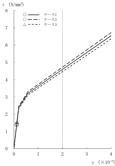
図2-20 τ - γ 関係と最大応答値 (Ss-3, NS方向, 4F) (2/8)
