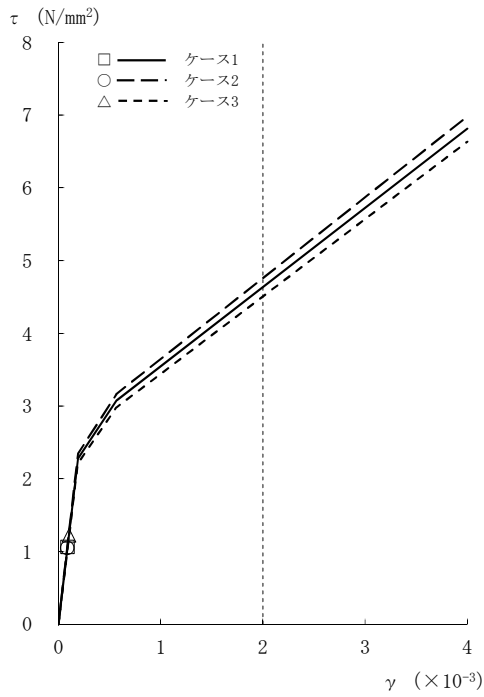
図2-20 τ - γ 関係と最大応答値 (Ss-3, NS方向, CRF) (1/8)
