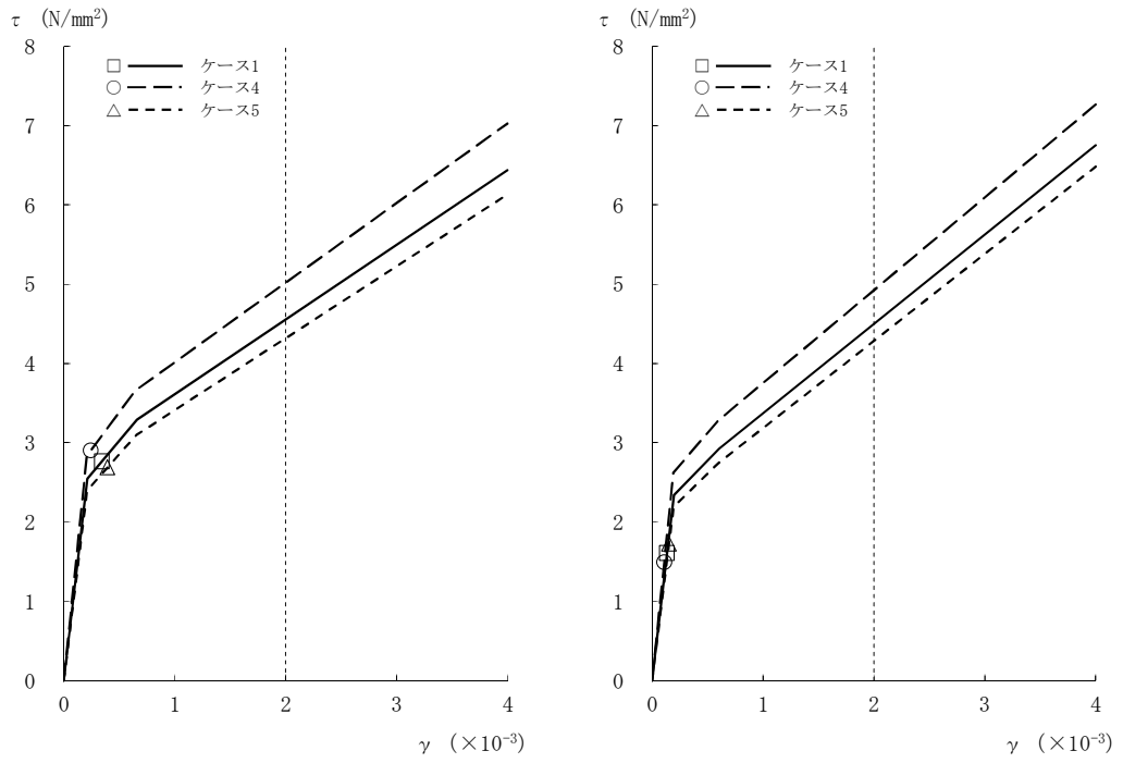
図2-62 \tau - \gamma 関係と最大応答値 (Ss-8, NS方向, 1F) (5/8)
