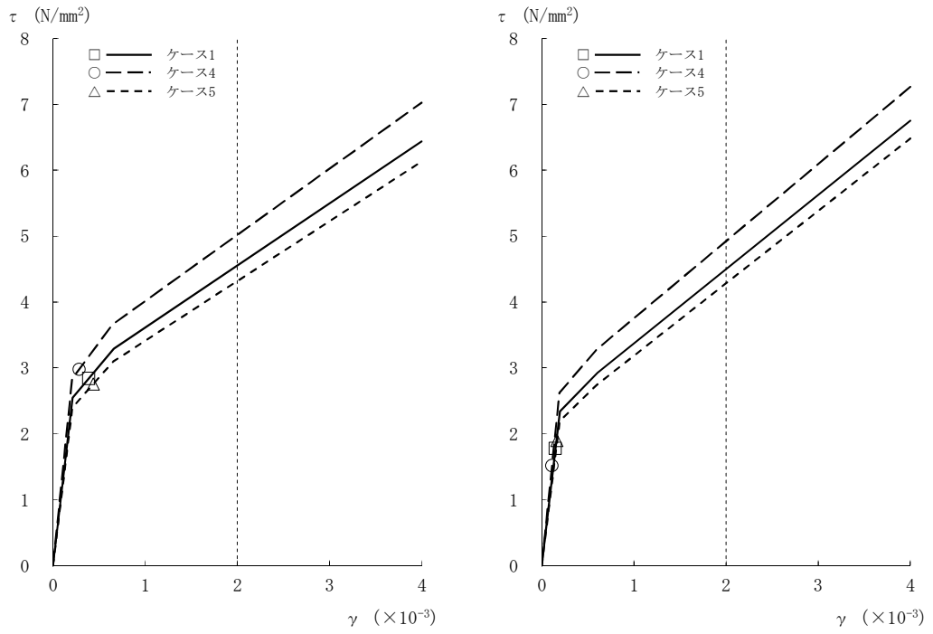
図2-59 \tau - \gamma 関係と最大応答値 (Ss-1, NS方向, 1F) (5/8)
