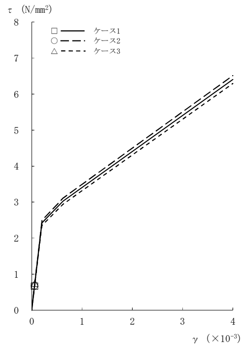
図2-38 \tau - \gamma 関係と最大応答値 (Sd-2, NS方向, B1F) (6/8)
