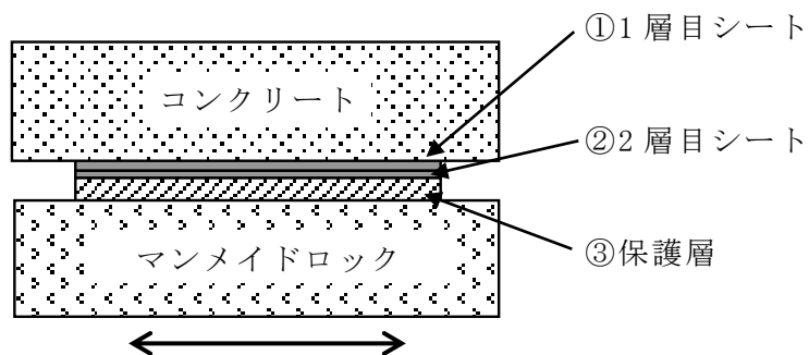
図 3-12 一方向載荷及び繰返し載荷試験供試体
