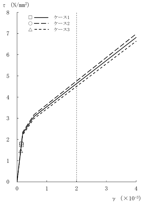
図2-18 \tau - \gamma 関係と最大応答値 (Ss-1, NS方向, CRF) (1/8)
