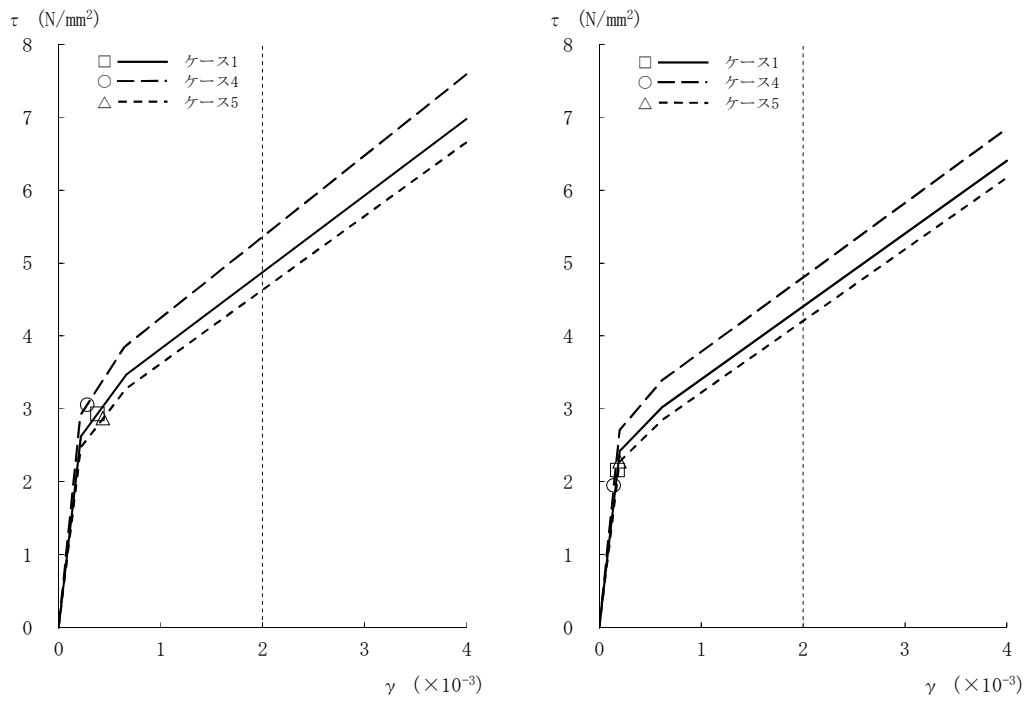
図2-62 \tau - \gamma 関係と最大応答値 (Ss-8, NS方向, B1F) (6/8)
