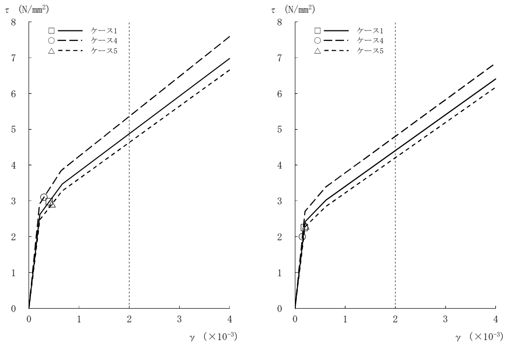
図2-59 \tau - \gamma 関係と最大応答値 (Ss-1, NS方向, B1F) (6/8)
