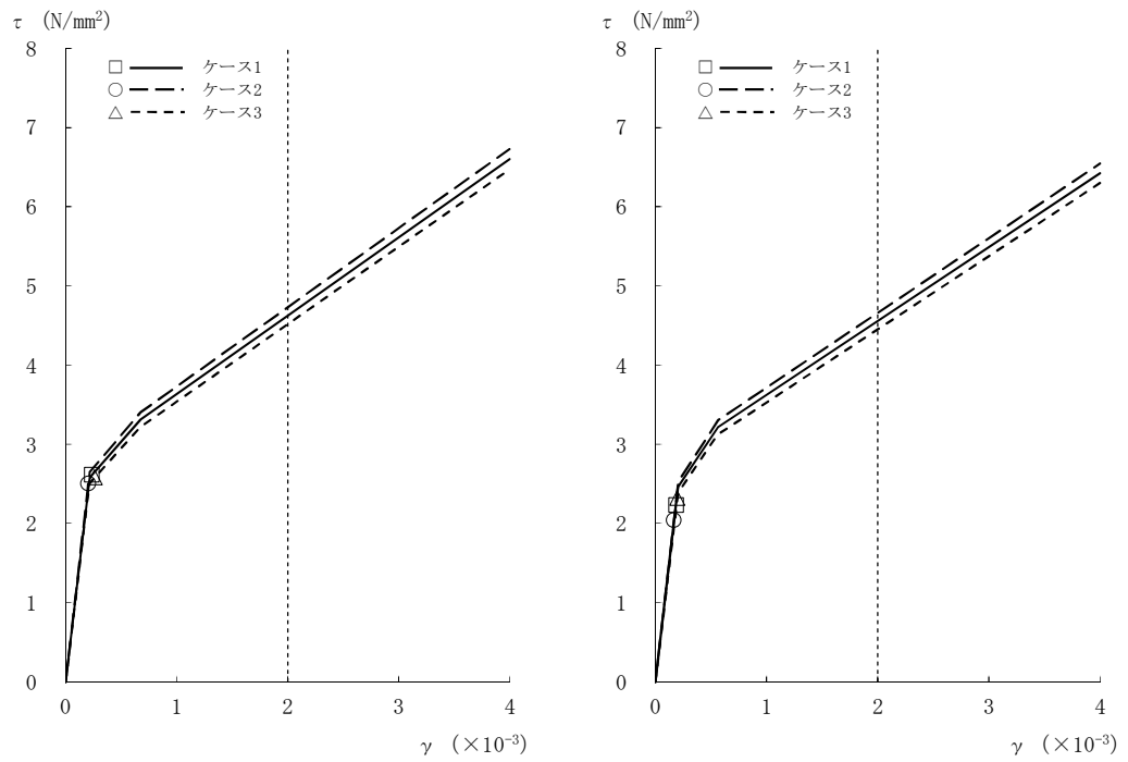
図2-25 τ - γ 関係と最大応答値 (Ss-8, EW方向, B3F) (8/8)
