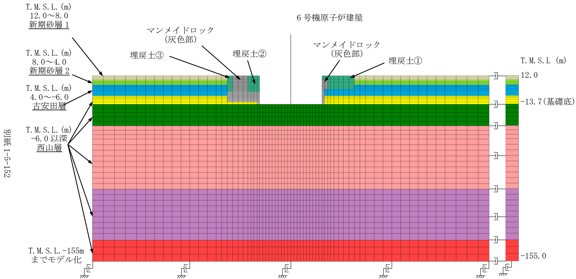
図 5-2 地盤精緻化モデルの地盤メッシュ図 (NS 方向)
