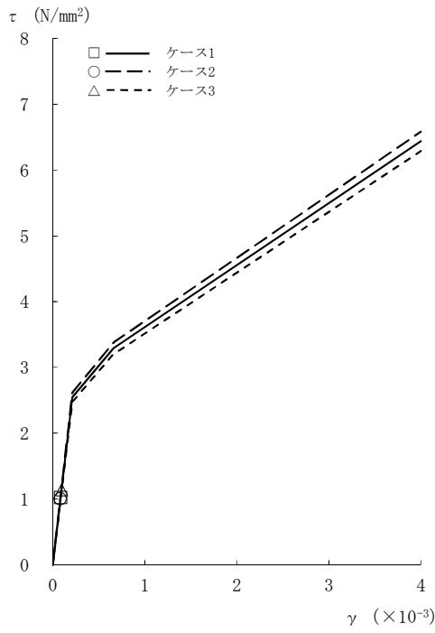
図2-38 \tau - \gamma 関係と最大応答値 (Sd-2, NS方向, 1F) (5/8)
