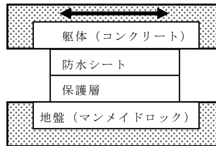
図 3-4 供試体（標準）
