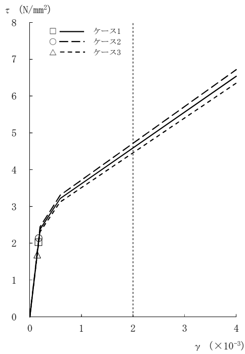
図2-18 \tau - \gamma 関係と最大応答値 (Ss-1, NS方向, 4F) (2/8)
