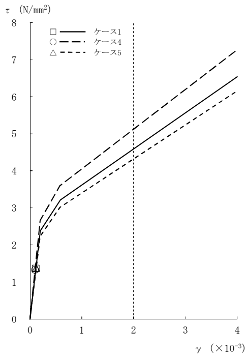
図2-60 \tau - \gamma 関係と最大応答値 (S s -2, NS方向, 4F) (2/8)
