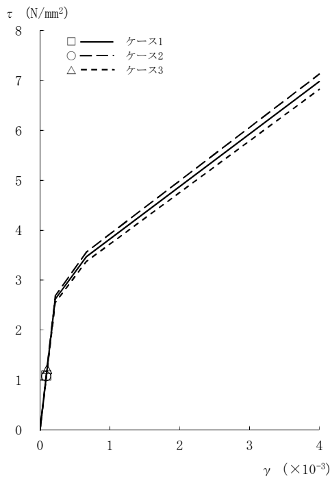
図2-38 \tau - \gamma 関係と最大応答値 (Sd-2, NS方向, B1F) (6/8)
