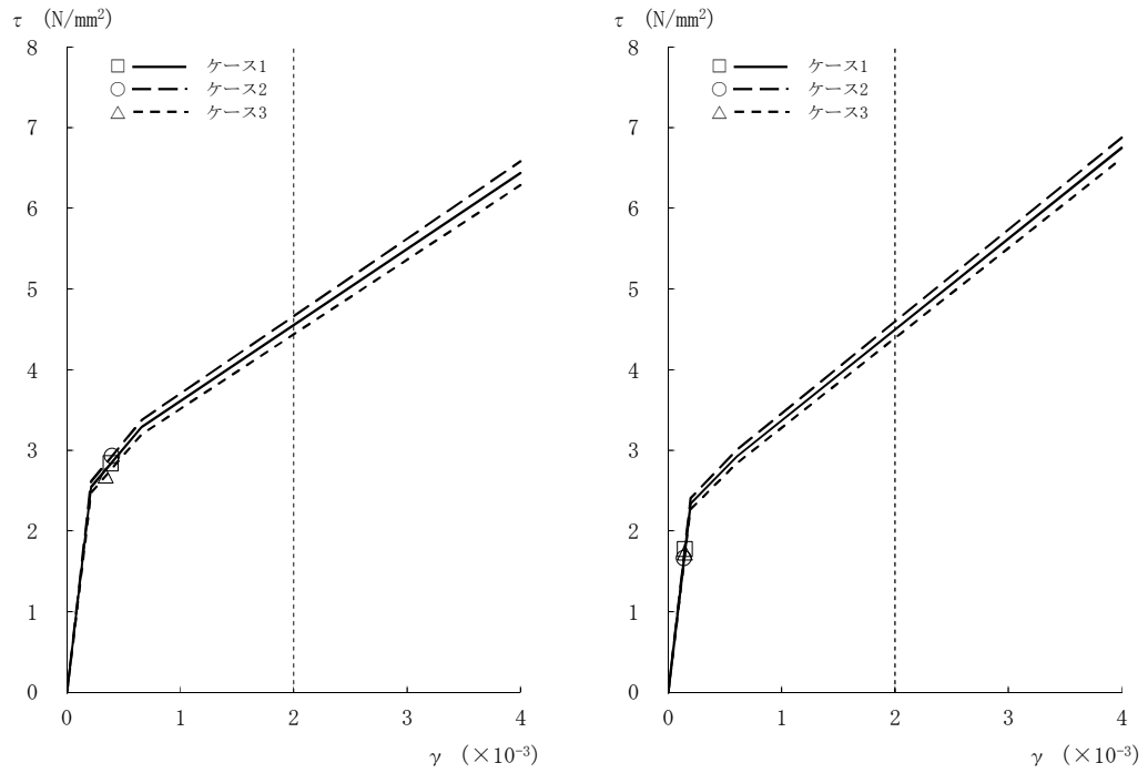
図2-18 τ - γ 関係と最大応答値 (Ss-1, NS方向, 1F) (5/8)
