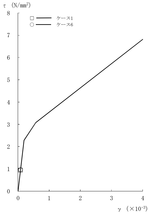
図2-116 τ - γ 関係と最大応答値 (Sd-1, NS方向, CRF) (1/8)
