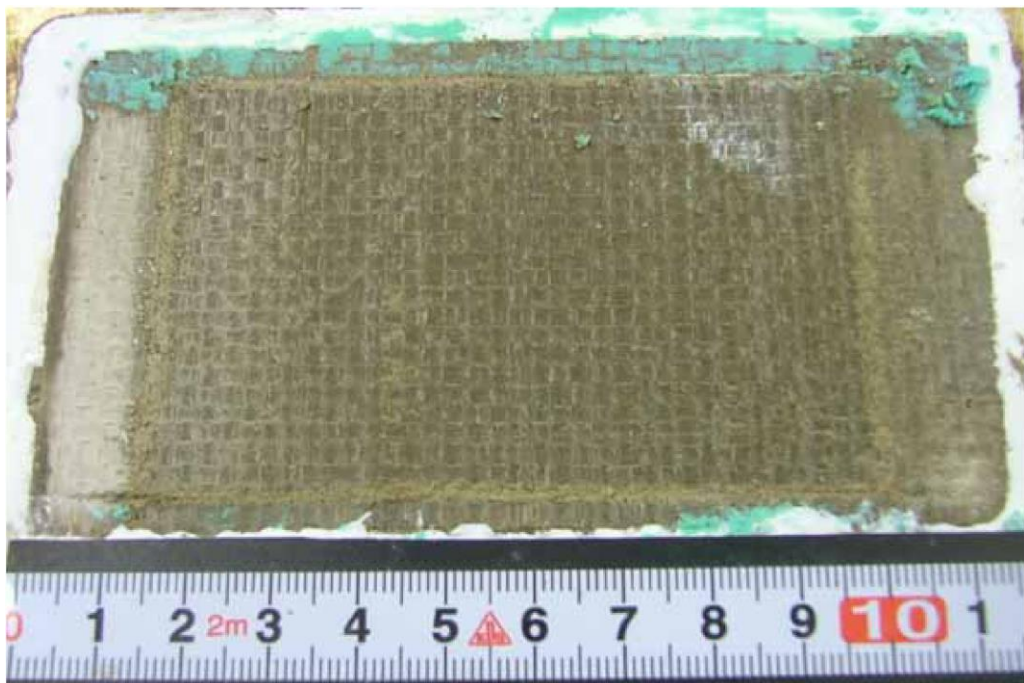
図 3-19 一方向荷重試験後の供試体状況 ケース 1-3 (マンメイドロック表面)
