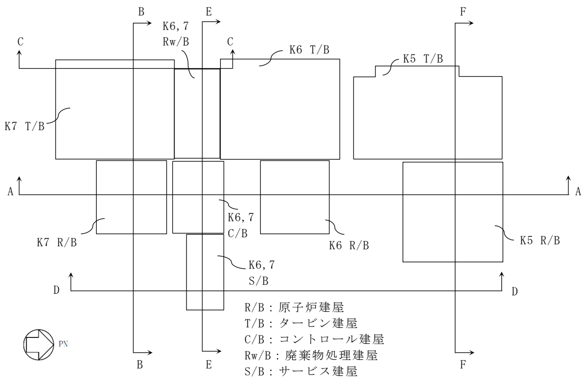
図 2-1 配置図
