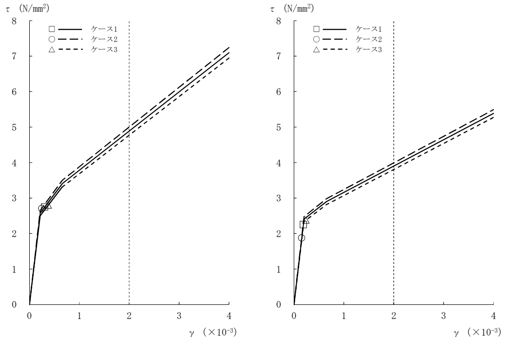
図2-25 τ - γ 関係と最大応答値 (Ss-8, EW方向, B2F) (7/8)
