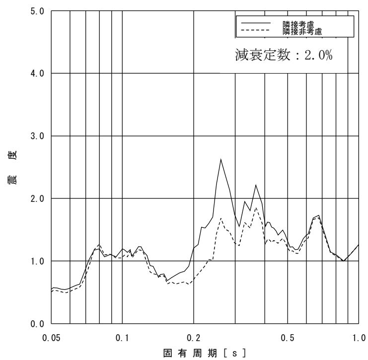
図 2-6 床応答スペクトルの比較 (原子炉遮蔽壁 T.M.S.L.15.600m, 水平方向, 減衰定数 2.0%)
