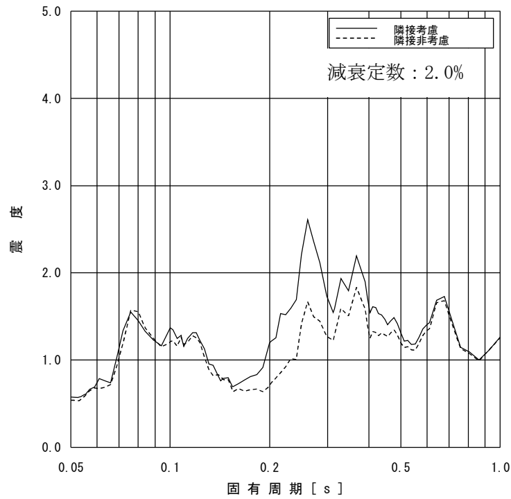
図 2-19 床応答スペクトルの比較 (原子炉压力容器 T. M. S. L. 15. 266m, 水平方向, 減衰定数 2. 0%)
