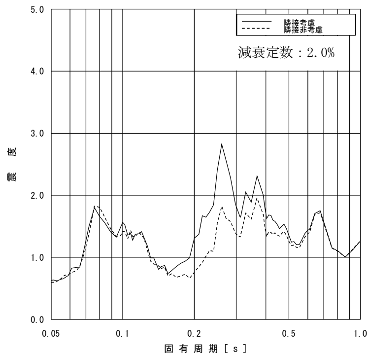
図 2-4 床応答スペクトルの比較 (原子炉遮蔽壁 T.M.S.L. 18. 440m, 水平方向, 減衰定数 2.0%)
