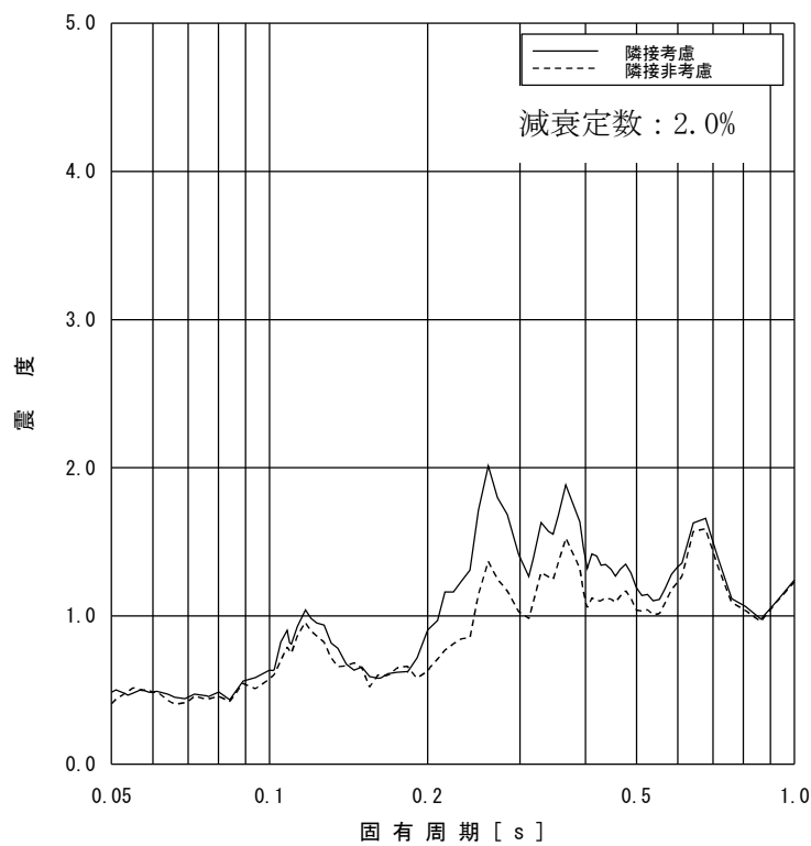
図 2-20 床応答スペクトルの比較 (原子炉压力容器 T. M. S. L. 5. 066m, 水平方向, 減衰定数 2. 0%)
