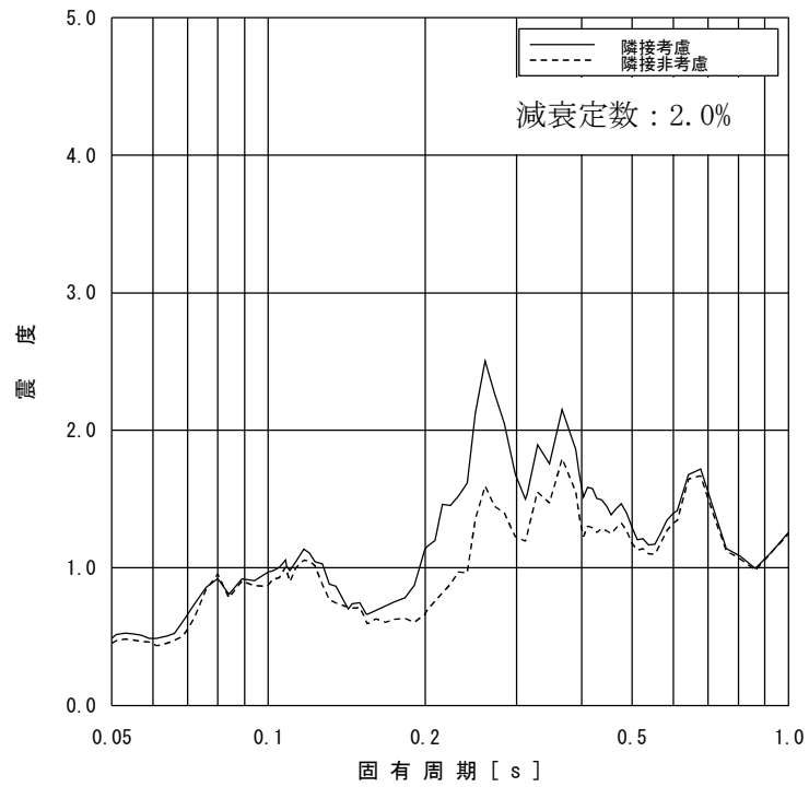
図 2-7 床応答スペクトルの比較 (原子炉遮蔽壁 T. M. S. L. 13. 9500m, 水平方向, 減衰定数 2. 0%)
