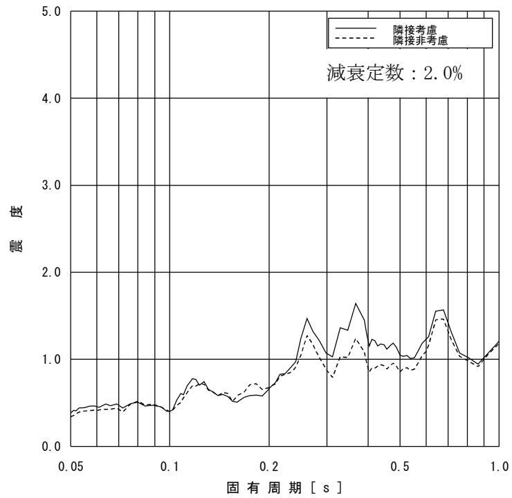
図 2-15 床応答スペクトルの比較 (原子炉本体基礎 T.M.S.L.-4.700m, 水平方向, 減衰定数 2.0%)
