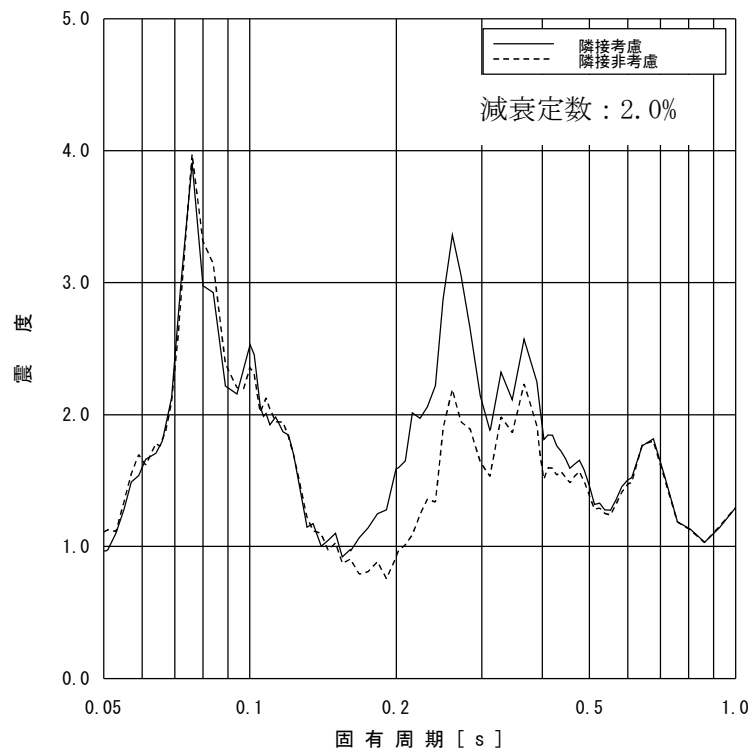
図 2-16 床応答スペクトルの比較 (原子炉圧力容器 T.M.S.L. 26.013m, 水平方向, 減衰定数 2.0%)
