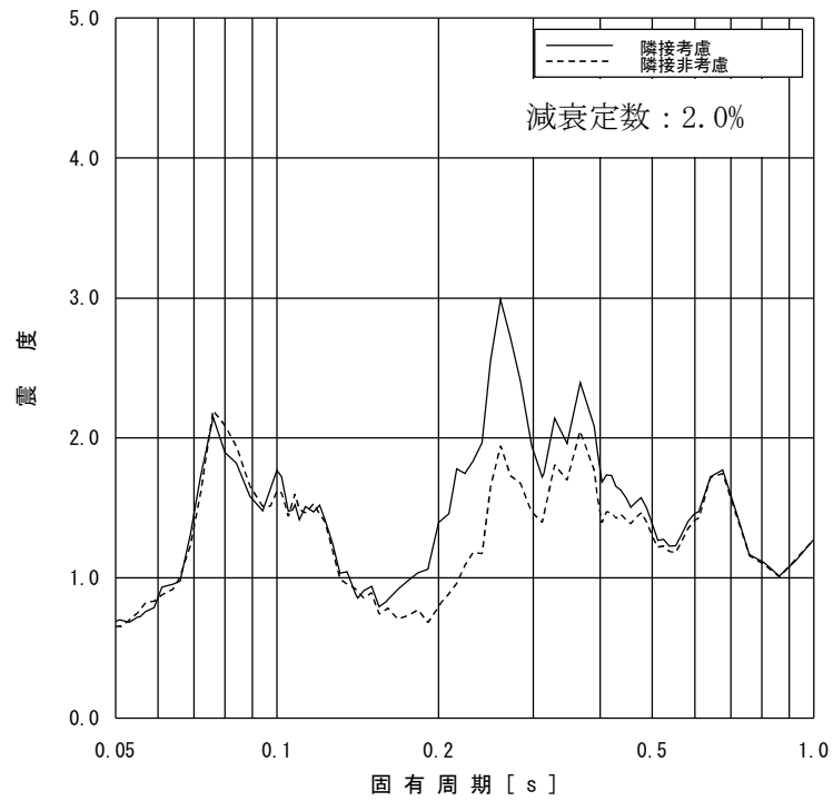
図 2-3 床応答スペクトルの比較 (原子炉遮蔽壁 T.M.S.L. 21. 200m, 水平方向, 減衰定数 2.0%)
