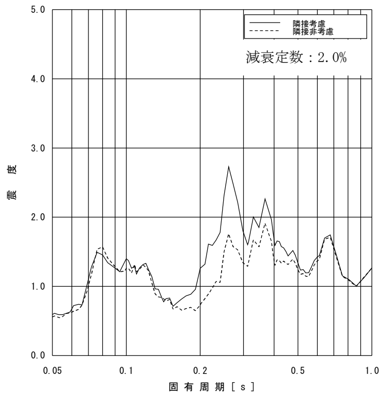
図 2-5 床応答スペクトルの比較 (原子炉遮蔽壁 T.M.S.L.17.020m, 水平方向, 減衰定数 2.0%)
