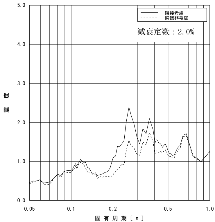
図 2-8 床応答スペクトルの比較 (原子炉本体基礎 T. M. S. L. 12. 300m, 水平方向, 減衰定数 2. 0%)
