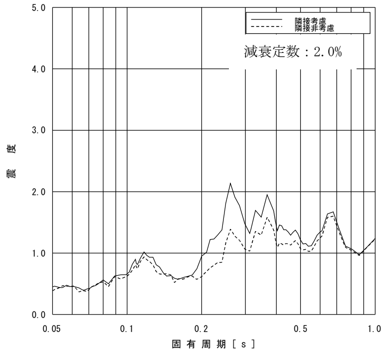
図 2-9 床応答スペクトルの比較 (原子炉本体基礎 T.M.S.L. 8.200m, 水平方向, 減衰定数 2.0%)
