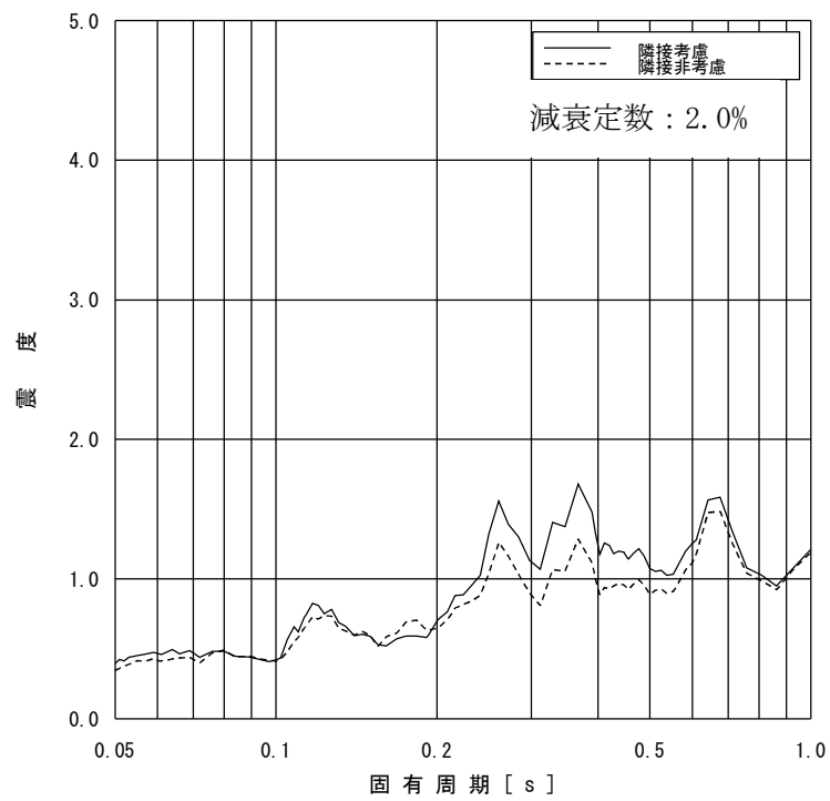
図 2-14 床応答スペクトルの比較 (原子炉本体基礎 T.M.S.L. -2.100m, 水平方向, 減衰定数 2.0%)
