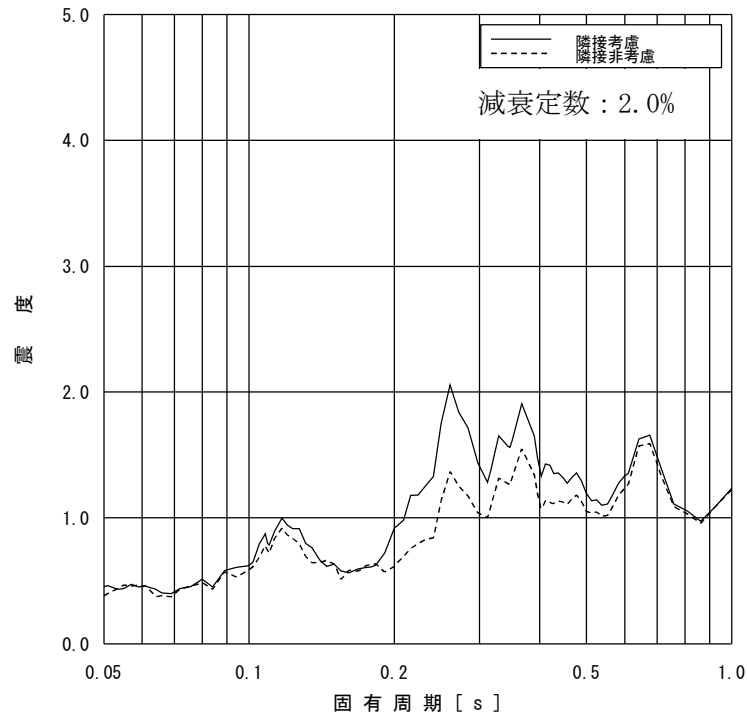
図 2-10 床応答スペクトルの比較 (原子炉本体基礎 T.M.S.L. 7.000m, 水平方向, 減衰定数 2.0%)
