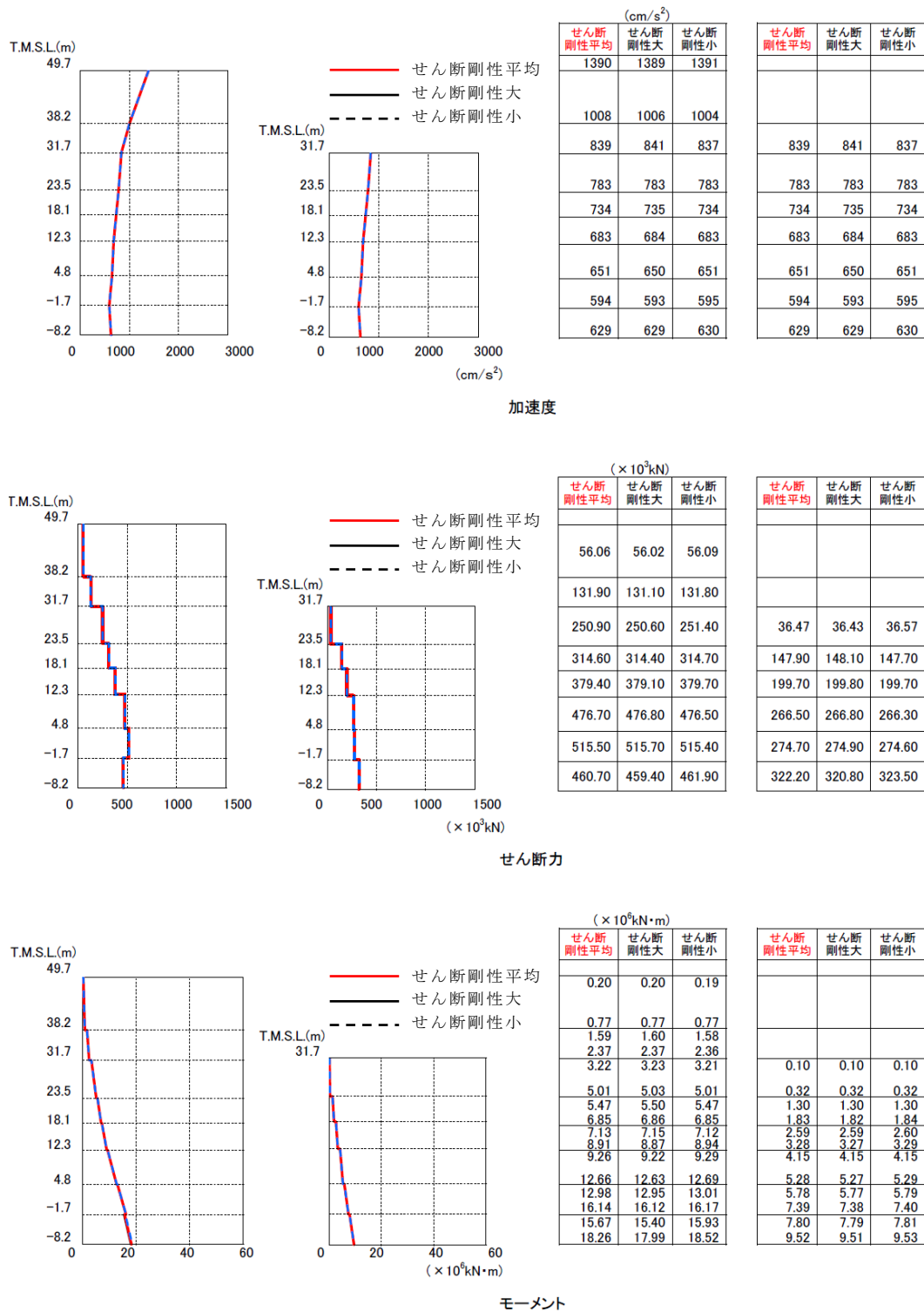
図 4-39 建屋の最大応答分布の比較 (せん断剛性: 平均, 大, 小)
