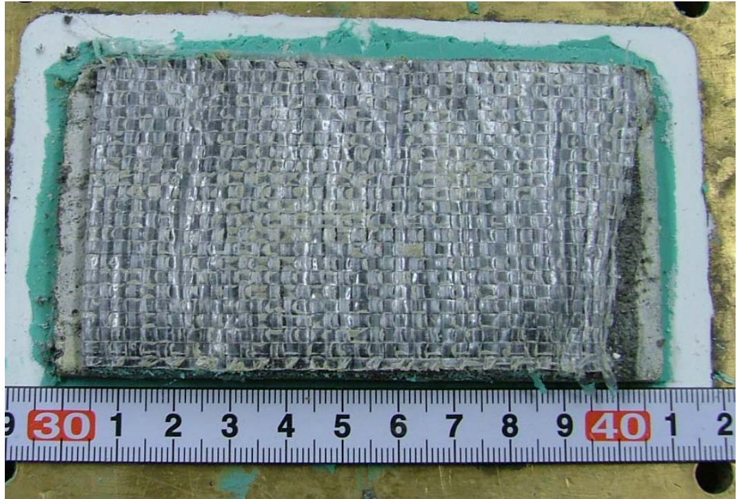
図 3-38 スケール影響試験後の供試体状況 ケース 2-1 (保護層表面)
