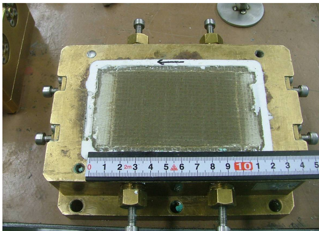
図 3-27 繰返し载荷試験後の供試体状況 ケース 1-6 (マンメイドロック表面)
