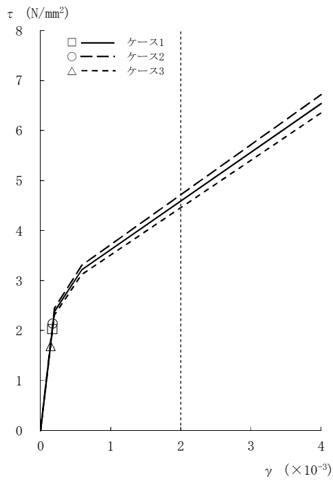
図4-20 τ - γ 関係と最大応答値 (Ss-1, NS方向, 4F) (2/8)
