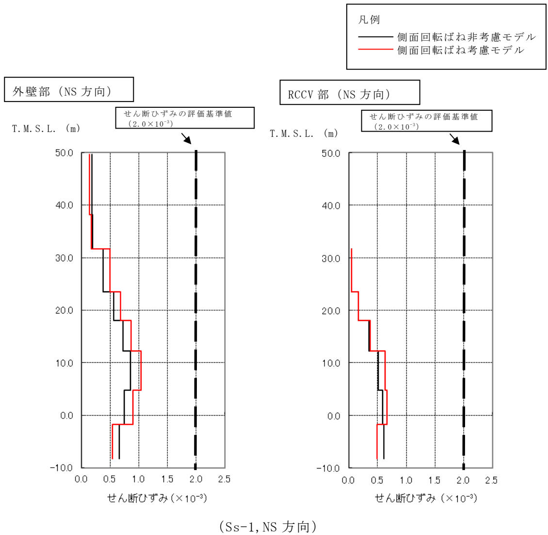
図 2-14 側面回転ばねが応答せん断ひずみに与える影響
