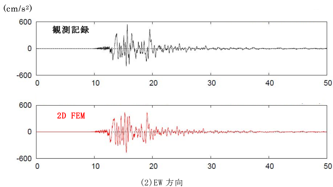
図 7 観測記録と解析結果の加速度波形の比較 (6号機原子炉建屋 3階 : T. M. S. L. 23.5m)
