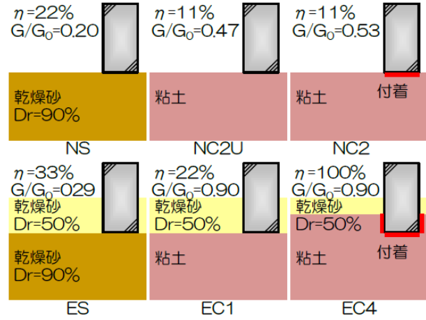
図3 遠心振動台実験のシミュレーション解析ケース
