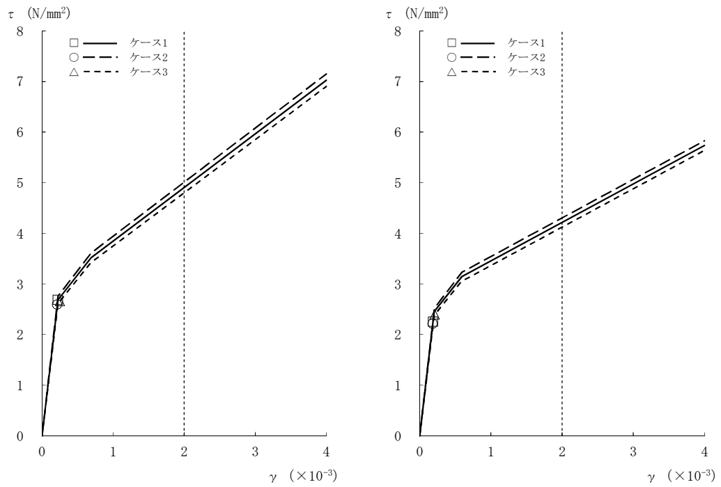
図2-18 \tau - \gamma 関係と最大応答値 (Ss-1, NS方向, B3F) (8/8)
