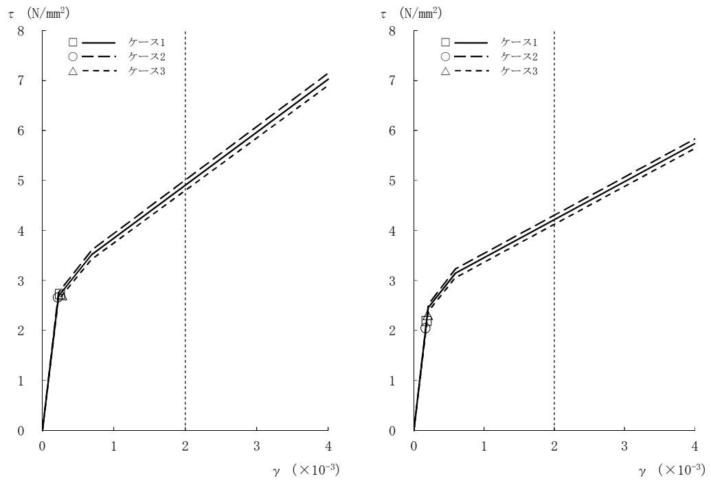
図2-21 \tau - \gamma 関係と最大応答値 (Ss-8, NS方向, B3F) (8/8)
