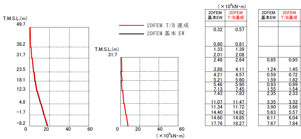
モーメント
