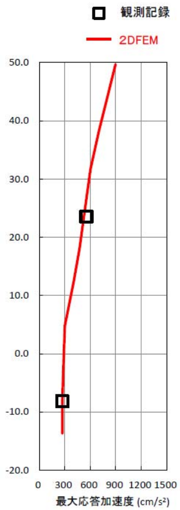
(1)NS 方向
