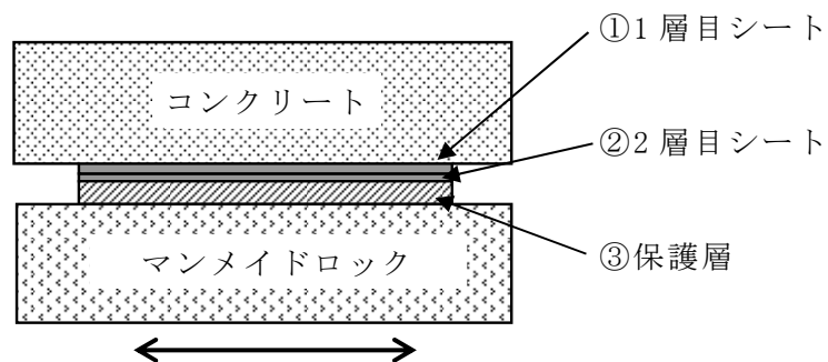
図 3-12 一方向載荷及び繰返し載荷試験供試体
