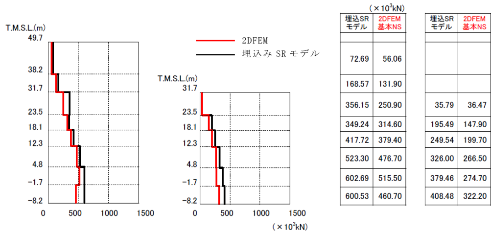
せん断力
