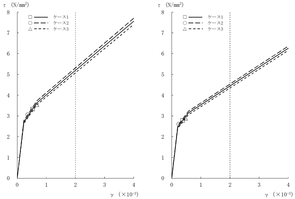
図2-21 \tau - \gamma 関係と最大応答値 (Ss-8, NS方向, B2F) (7/8)
