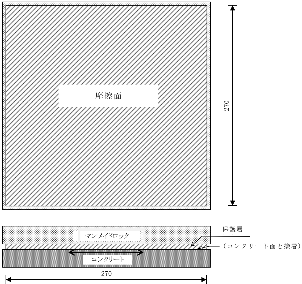
(大型供試体)
