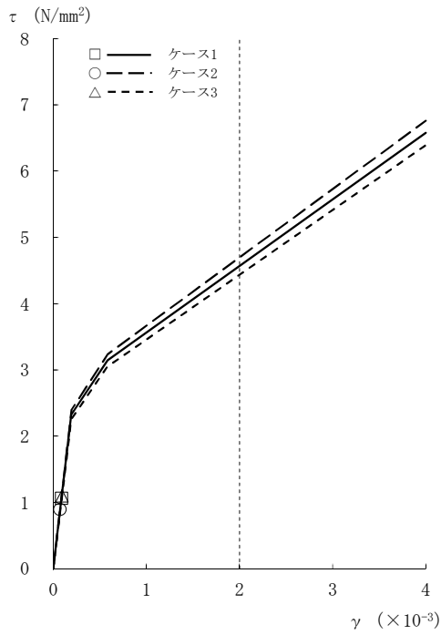
図2-23 \tau - \gamma 関係と最大応答値 (Ss-2, EW方向, CRF) (1/8)
