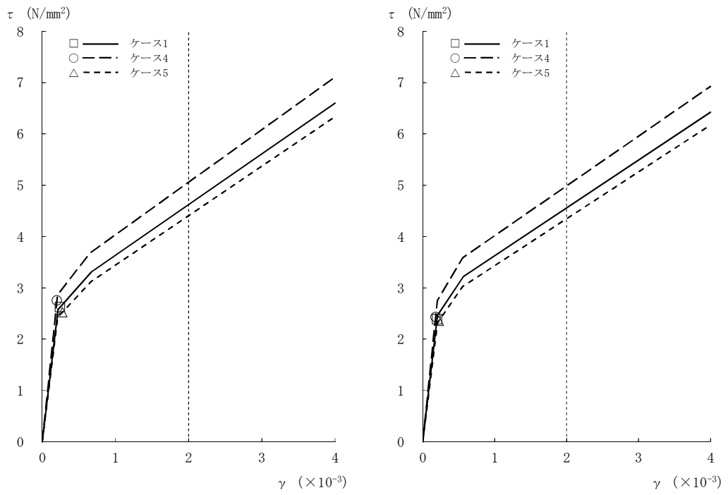
図4-40 \tau - \gamma 関係と最大応答値 (Ss-1, EW方向, B3F) (8/8)
