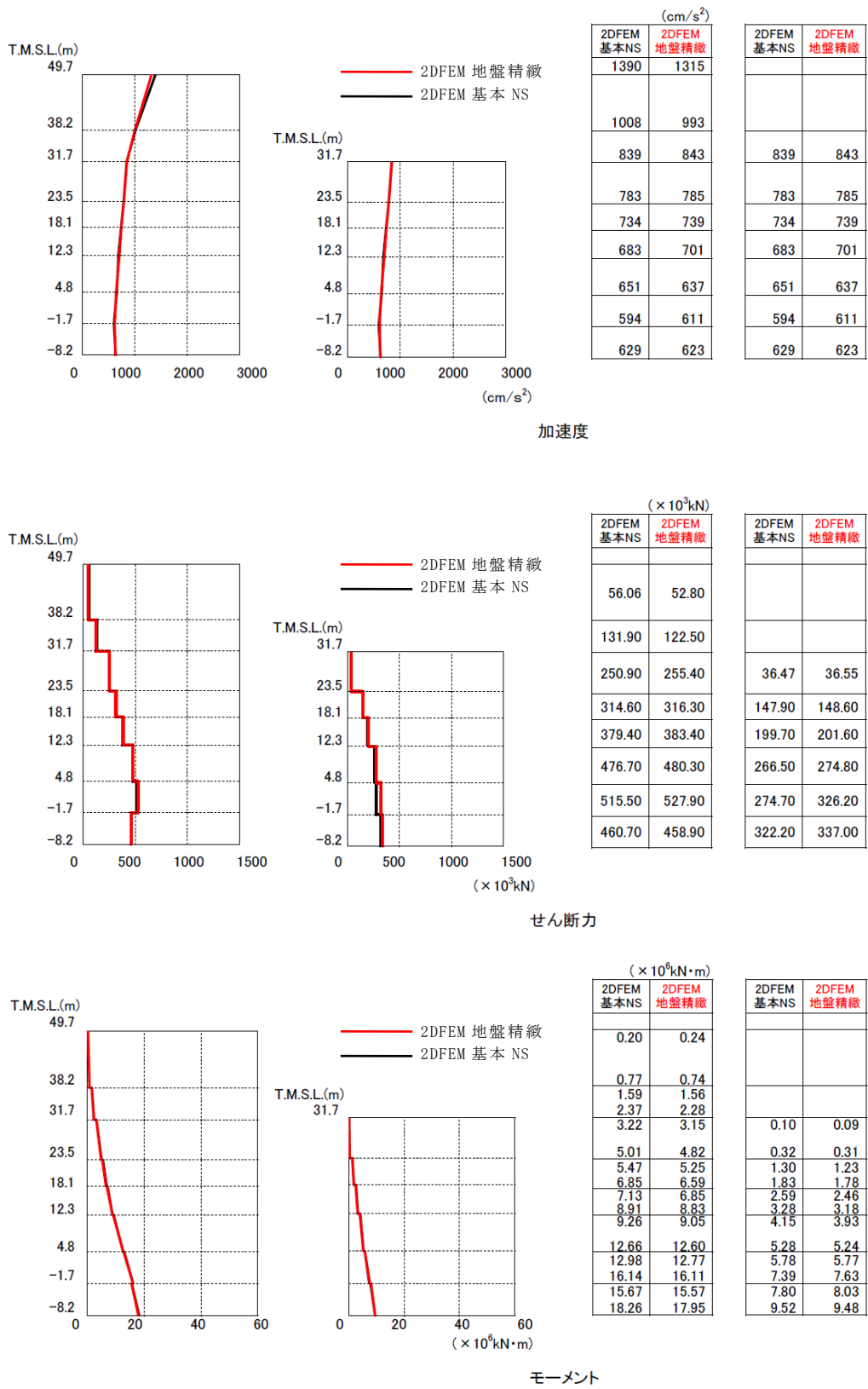
図 5-14 建屋の最大応答分布の比較 (基本モデルと地盤精緻化モデル, NS 方向)
