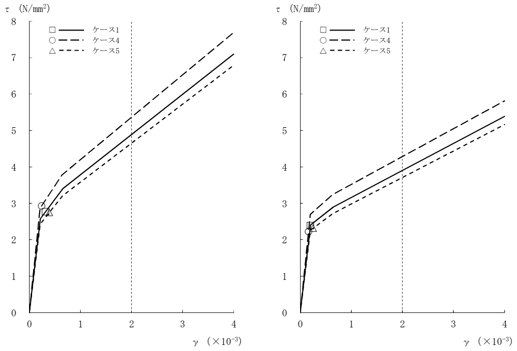
図4-40 \tau - \gamma 関係と最大応答値 (Ss-1, EW方向, B2F) (7/8)
