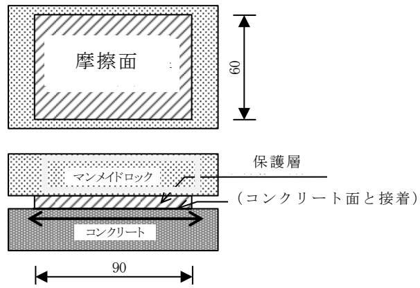
(中型供試体)
