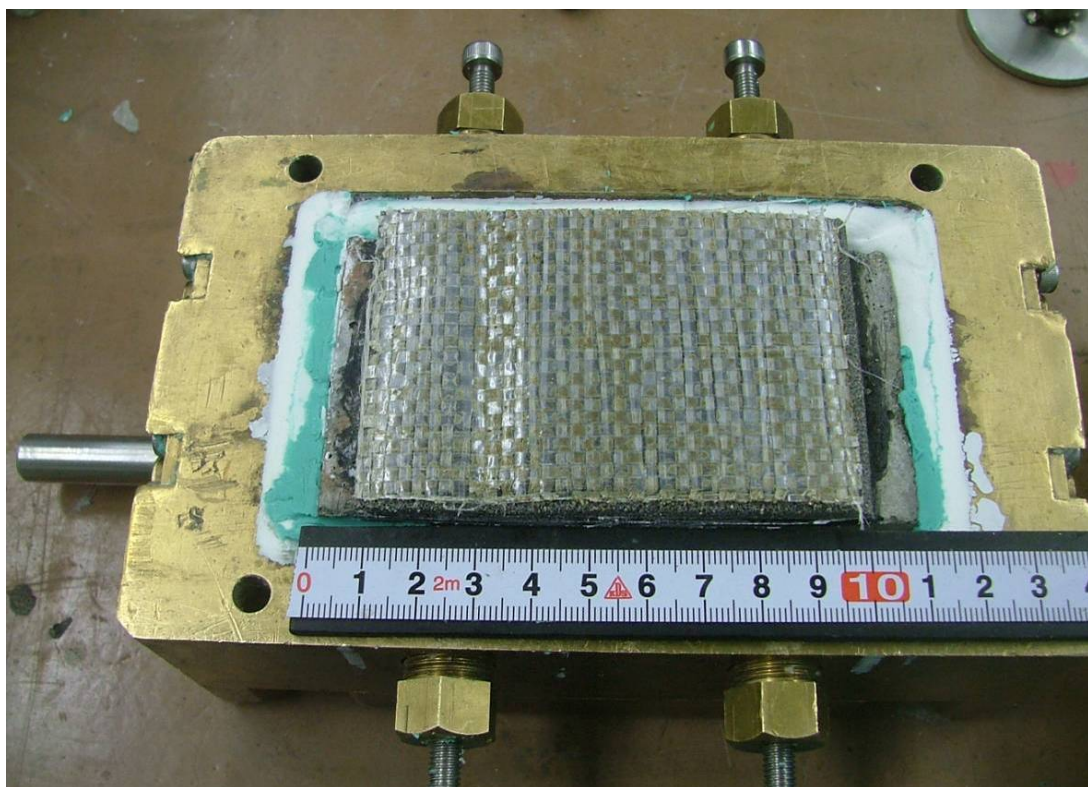
図 3-26 繰返し载荷試験後の供試体状況 ケース 1-6 (保護層表面)
