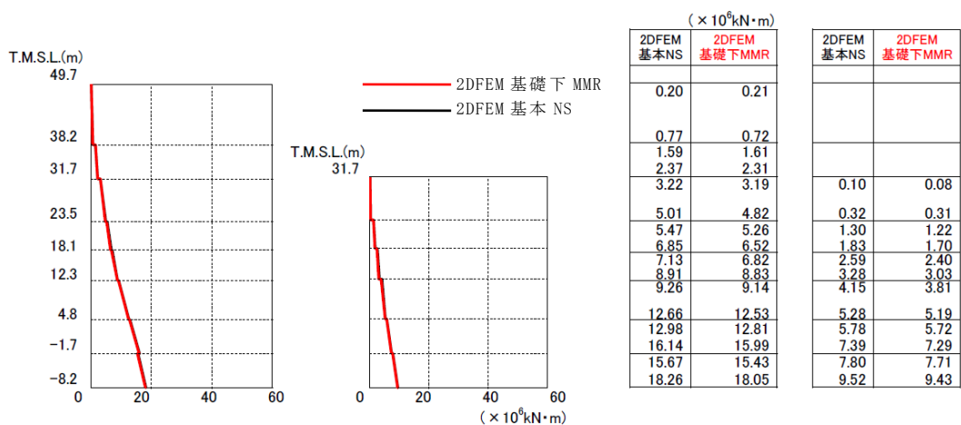
モーメント
