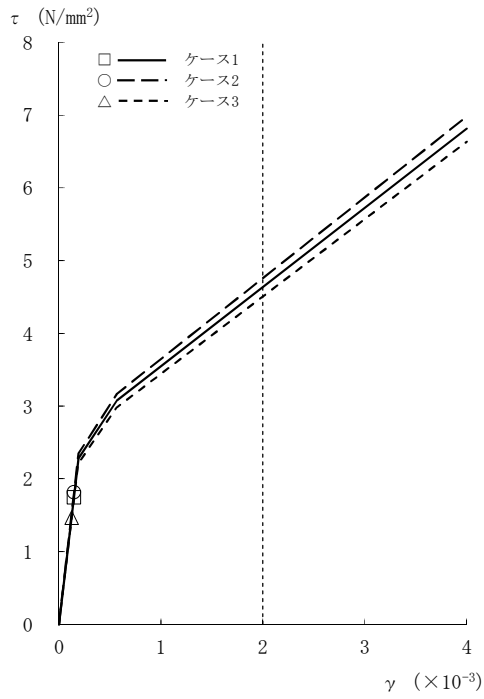
図4-20 τ - γ 関係と最大応答値 (Ss-1, NS方向, CRF) (1/8)
