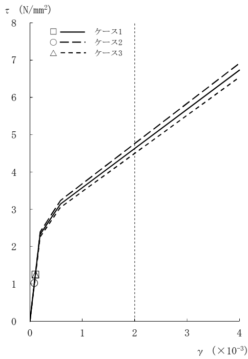
図2-23 \tau - \gamma 関係と最大応答値 (Ss-2, EW方向, 4F) (2/8)
