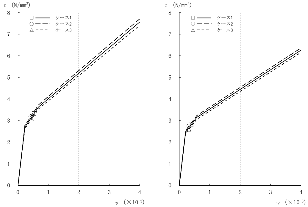
図2-18 \tau - \gamma 関係と最大応答値 (Ss-1, NS方向, B2F) (7/8)
