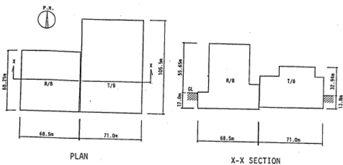
建屋の概要
