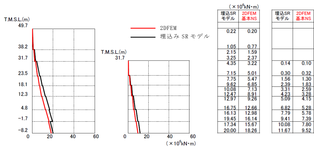
モーメント
