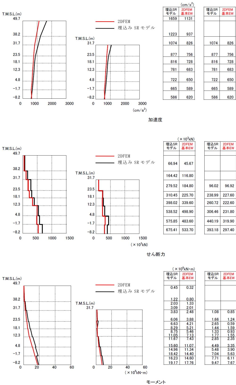
図 4-36 建屋の最大応答分布の比較 (基本モデルと埋込み SR モデル) (EW 方向)
