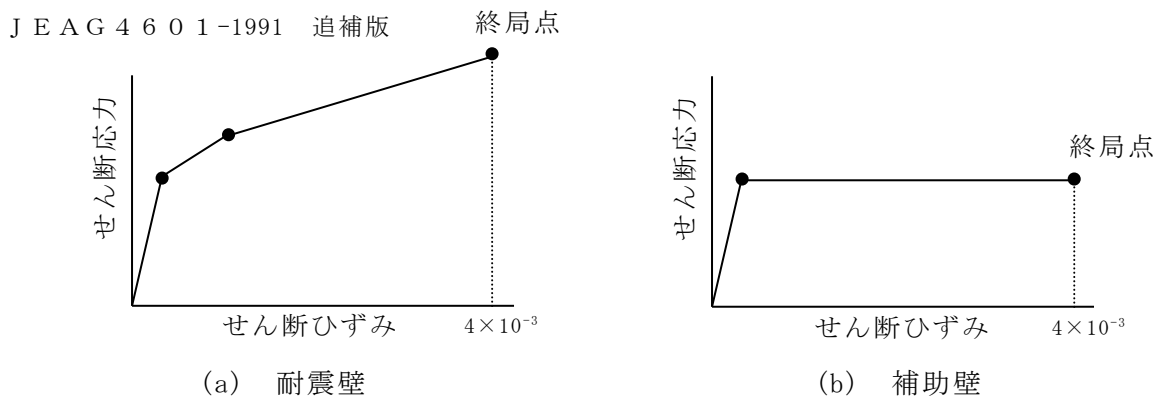
図3-1 せん断に関するスケルトン曲線の概念図
