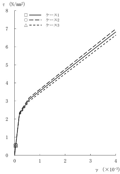
図2-38 \tau - \gamma 関係と最大応答値 (Sd-2, NS方向, CRF) (1/8)
