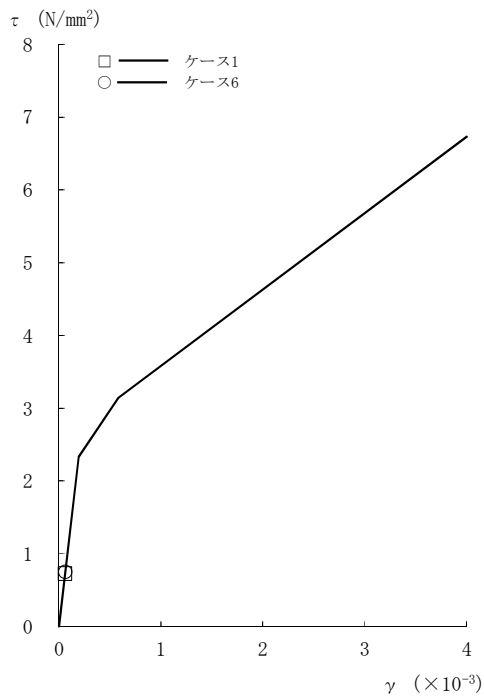
図2-120 \tau - \gamma 関係と最大応答値 (Sd-1, EW方向, 4F) (2/8)
