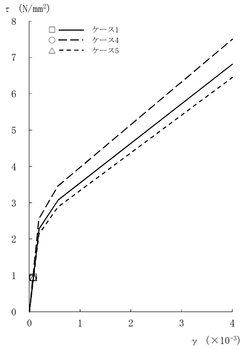
図2-78 \tau - \gamma 関係と最大応答値 (Sd-1, NS方向, CRF) (1/8)
