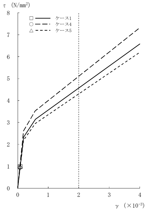
図2-66 \tau - \gamma 関係と最大応答値 (Ss-8, EW方向, CRF) (1/8)
