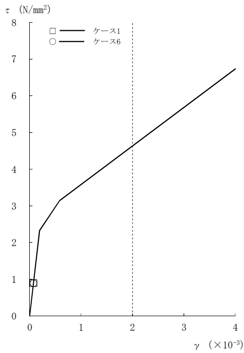
図2-106 τ - γ 関係と最大応答値 (Ss-3, EW方向, 4F) (2/8)
