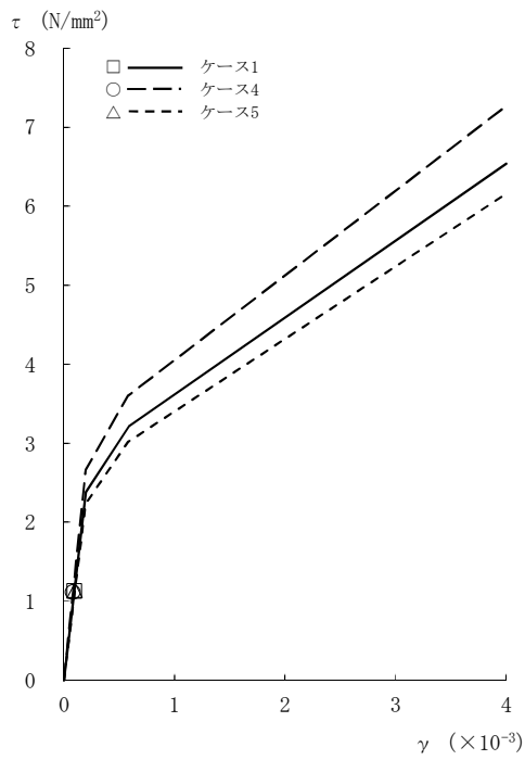
図2-78 \tau - \gamma 関係と最大応答値 (Sd-1, NS方向, 4F) (2/8)
