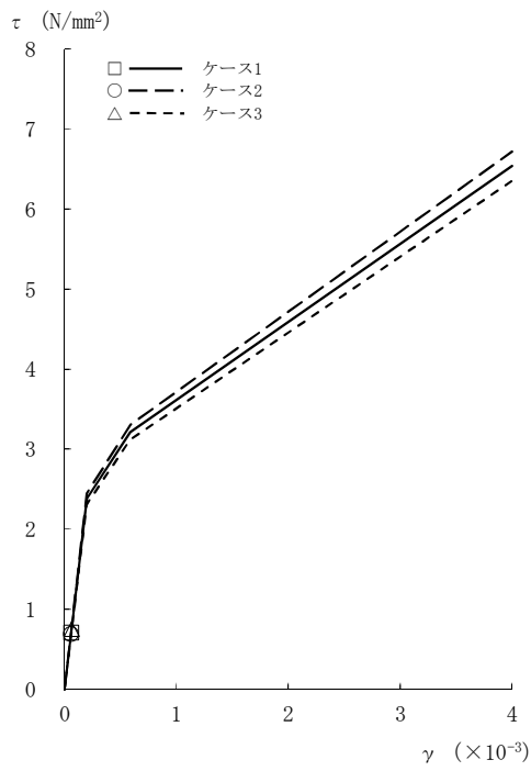
図2-39 \tau - \gamma 関係と最大応答値 (Sd-3, NS方向, 4F) (2/8)
