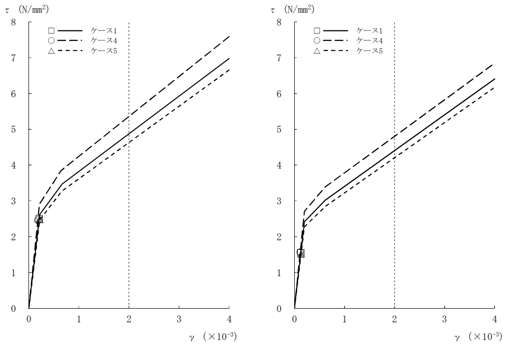
図2-61 \tau - \gamma 関係と最大応答値 (Ss-3, NS方向, B1F) (6/8)
