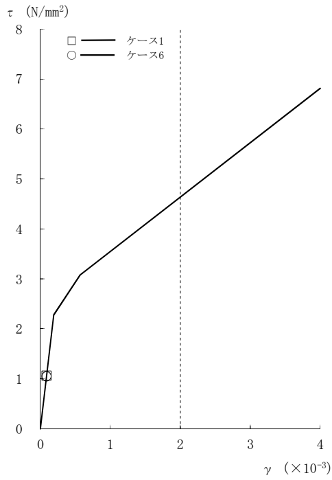
図2-102 τ - γ 関係と最大応答値 (Ss-3, NS方向, CRF) (1/8)
