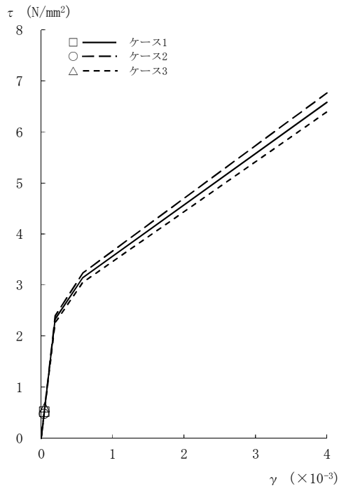
図2-42 \tau - \gamma 関係と最大応答値 (Sd-2, EW方向, CRF) (1/8)
