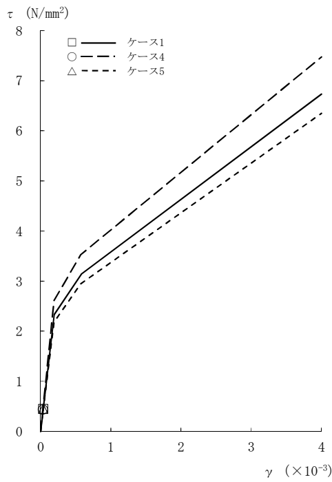
図2-84 \tau - \gamma 関係と最大応答値 (Sd-3, EW方向, 4F) (2/8)
