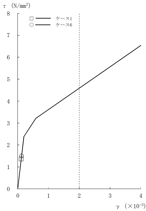
図2-101 τ - γ 関係と最大応答値 (Ss-2, NS方向, 4F) (2/8)
