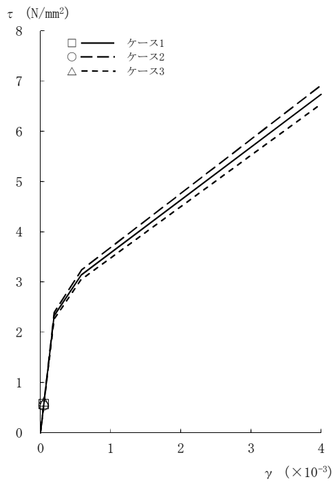
図2-44 \tau - \gamma 関係と最大応答値 (Sd-8, EW方向, 4F) (2/8)
