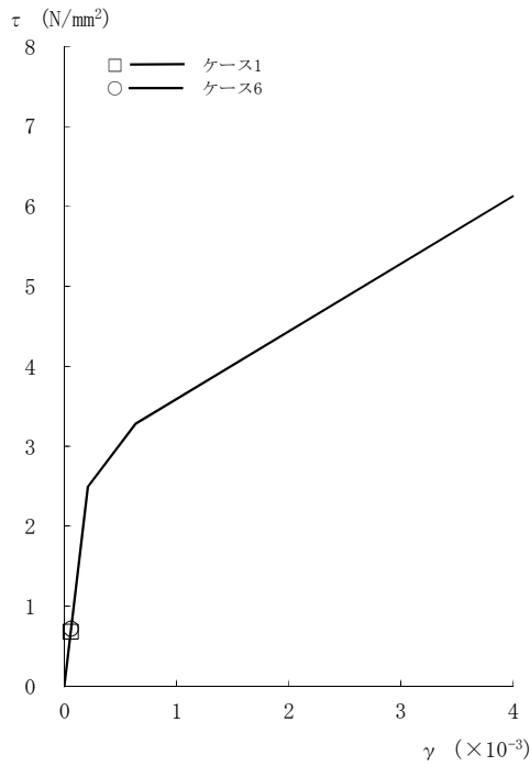
図2-123 τ - γ 関係と最大応答値 (Sd-8, EW方向, 3F) (3/8)
