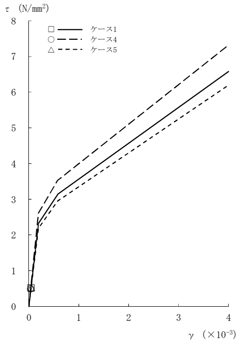
図2-83 \tau - \gamma 関係と最大応答値 (Sd-2, EW方向, CRF) (1/8)
