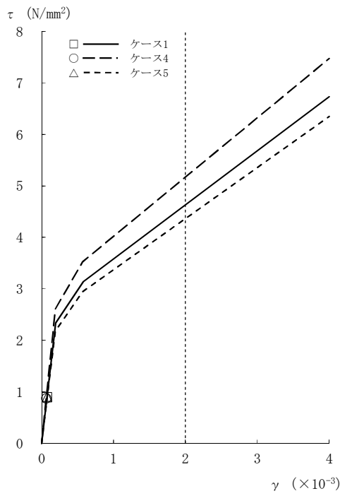
図2-65 \tau - \gamma 関係と最大応答値 (Ss-3, EW方向, 4F) (2/8)
