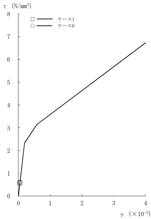
図2-123 \tau - \gamma 関係と最大応答値 (Sd-8, EW方向, 4F) (2/8)
