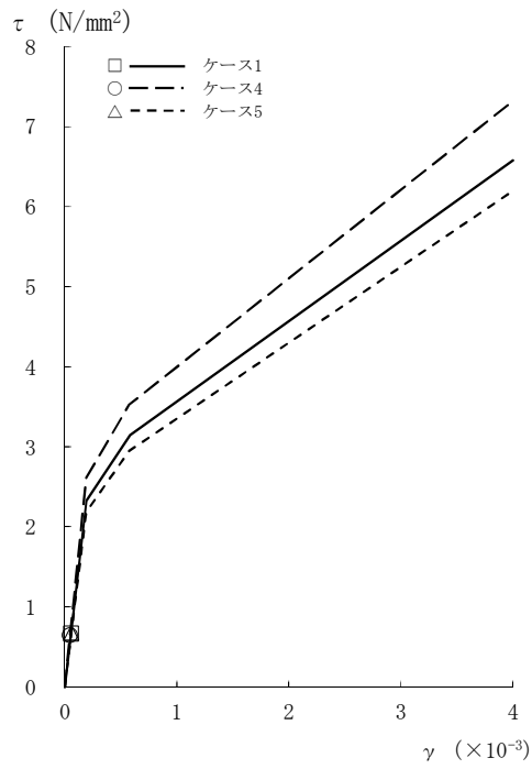
図2-82 τ - γ 関係と最大応答値 (Sd-1, EW方向, CRF) (1/8)
