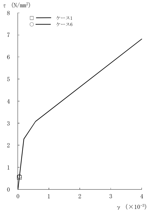
図2-118 \tau - \gamma 関係と最大応答値 (Sd-3, NS方向, CRF) (1/8)
