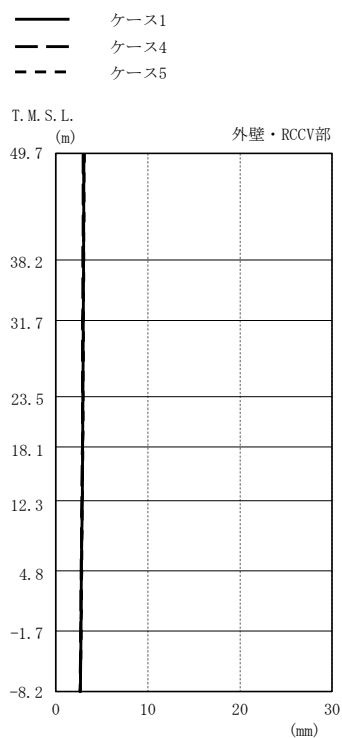
図2-54 最大応答変位(基準地震動 S s , 鉛直方向)(2/2)
