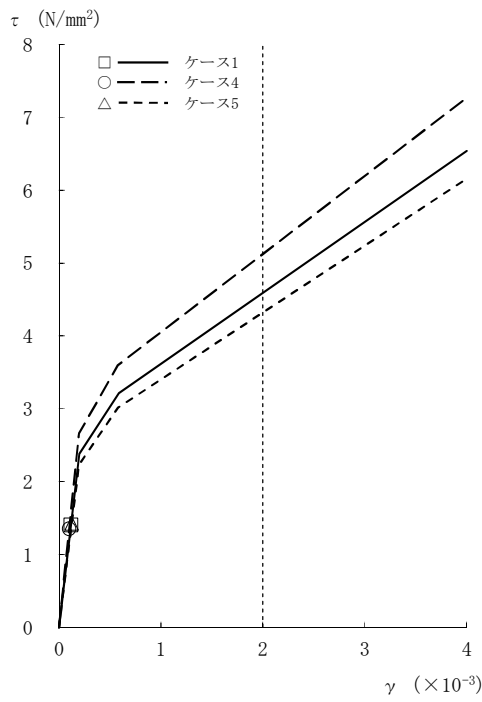
図2-61 \tau - \gamma 関係と最大応答値 (Ss-3, NS方向, 4F) (2/8)
