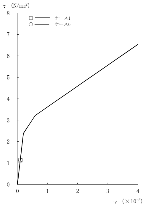
図2-116 \tau - \gamma 関係と最大応答値 (Sd-1, NS方向, 4F) (2/8)
