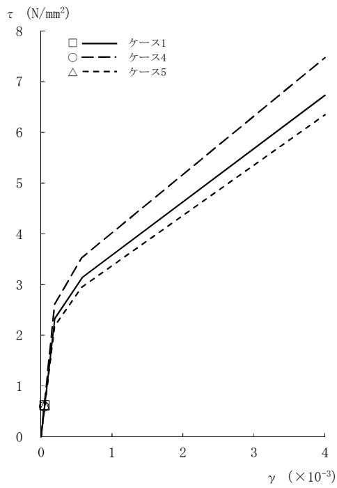
図2-83 \tau - \gamma 関係と最大応答値 (Sd-2, EW方向, 4F) (2/8)
