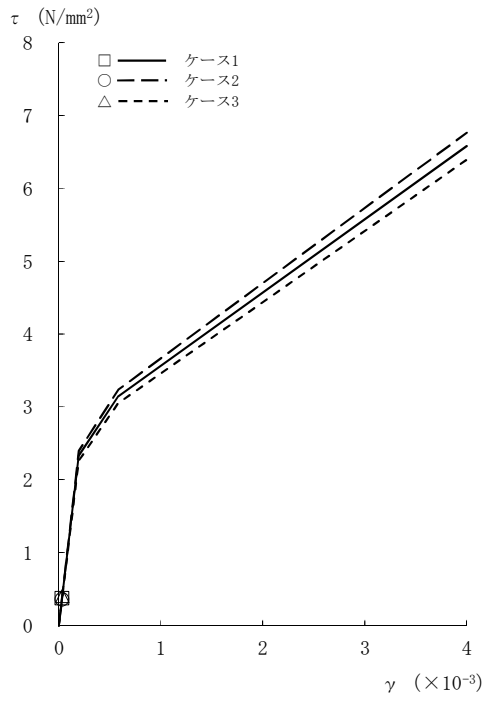
図2-43 \tau - \gamma 関係と最大応答値 (Sd-3, EW方向, CRF) (1/8)
