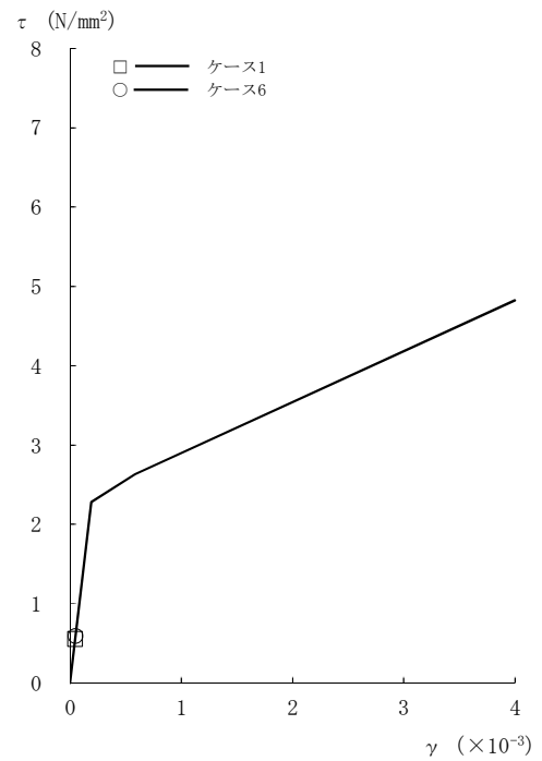
図2-123 τ - γ 関係と最大応答値 (Sd-8, EW方向, 2F) (4/8)
