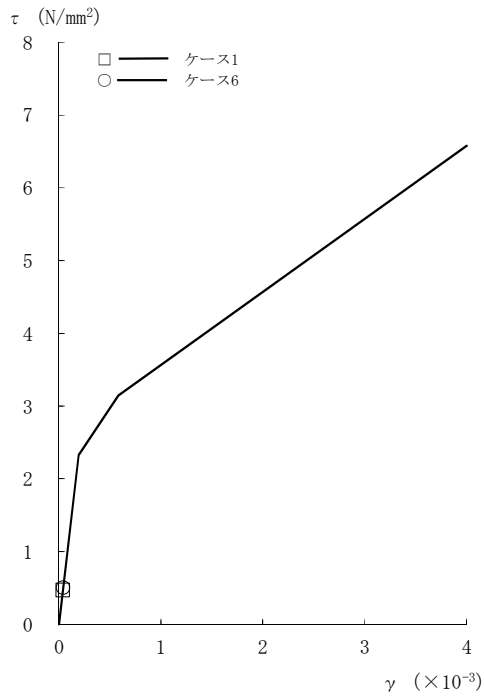
図2-123 \tau - \gamma 関係と最大応答値 (Sd-8, EW方向, CRF) (1/8)
