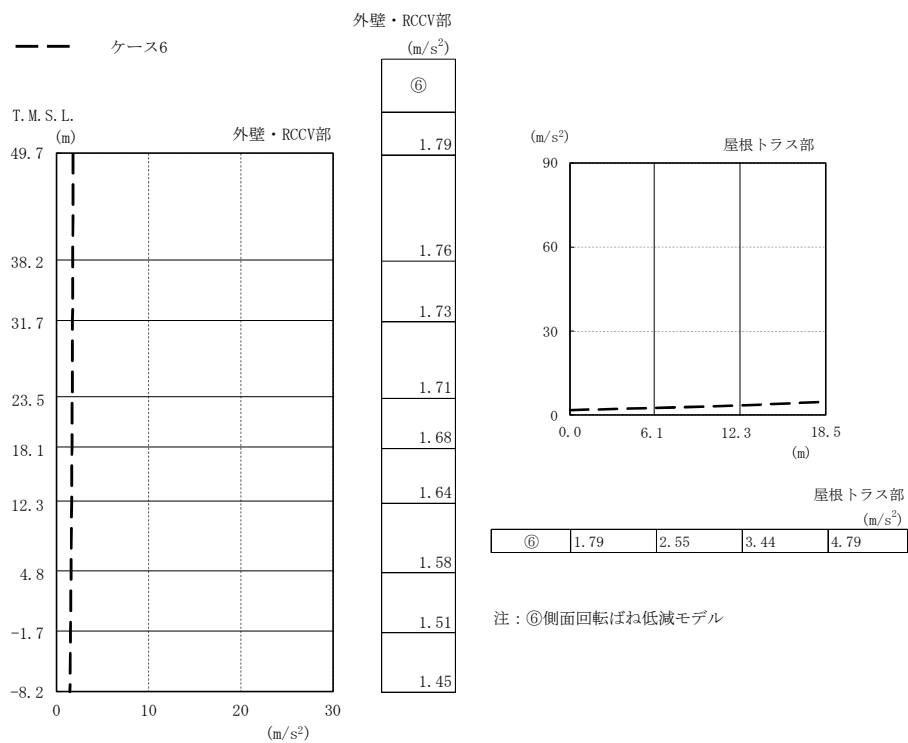
図2-97 最大応答加速度（基準地震動 S s ，EW方向，誘発上下動）（2/2）
