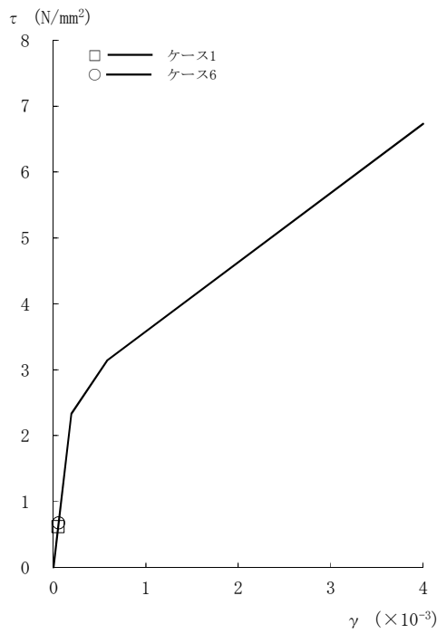
図2-121 \tau - \gamma 関係と最大応答値 (Sd-2, EW方向, 4F) (2/8)
