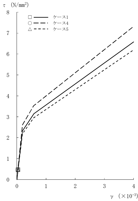
図2-85 \tau - \gamma 関係と最大応答値 (Sd-8, EW方向, CRF) (1/8)
