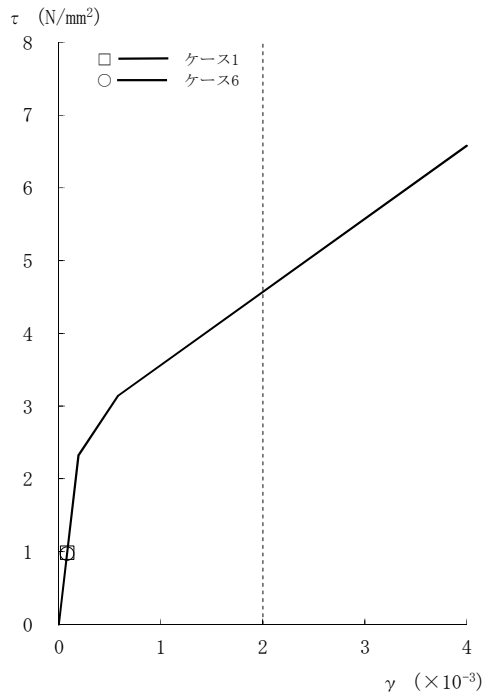
図2-107 \tau - \gamma 関係と最大応答値 (Ss-8, EW方向, CRF) (1/8)
