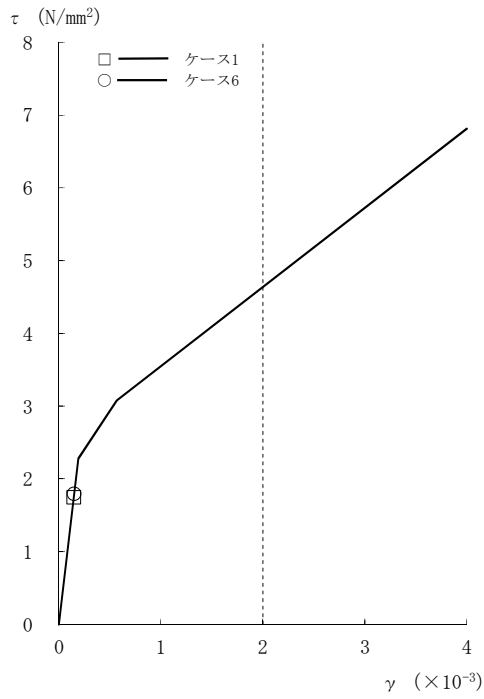
図2-100 \tau - \gamma 関係と最大応答値 (Ss-1, NS方向, CRF) (1/8)
