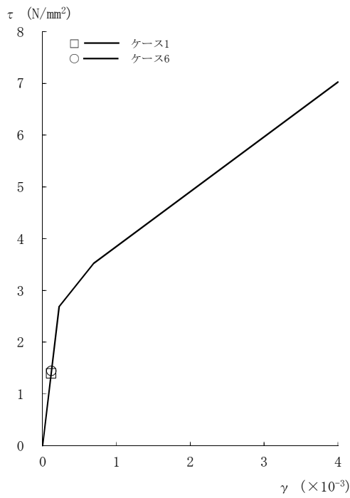
図2-119 τ - γ 関係と最大応答値 (Sd-8, NS方向, B3F) (8/8)
