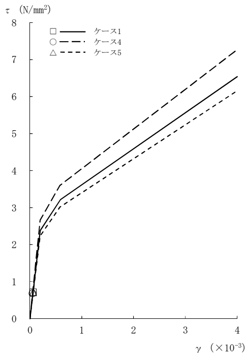
図2-80 \tau - \gamma 関係と最大応答値 (Sd-3, NS方向, 4F) (2/8)
