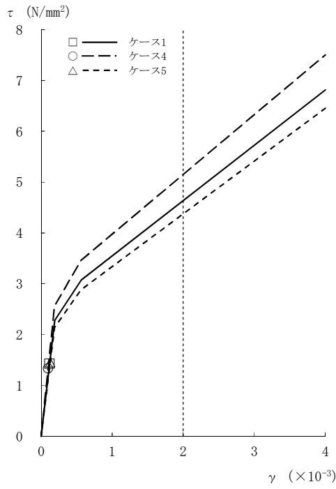
図2-62 τ - γ 関係と最大応答値 (S s -8, NS方向, CRF) (1/8)
