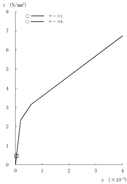
図2-122 \tau - \gamma 関係と最大応答値 (Sd-3, EW方向, 4F) (2/8)
