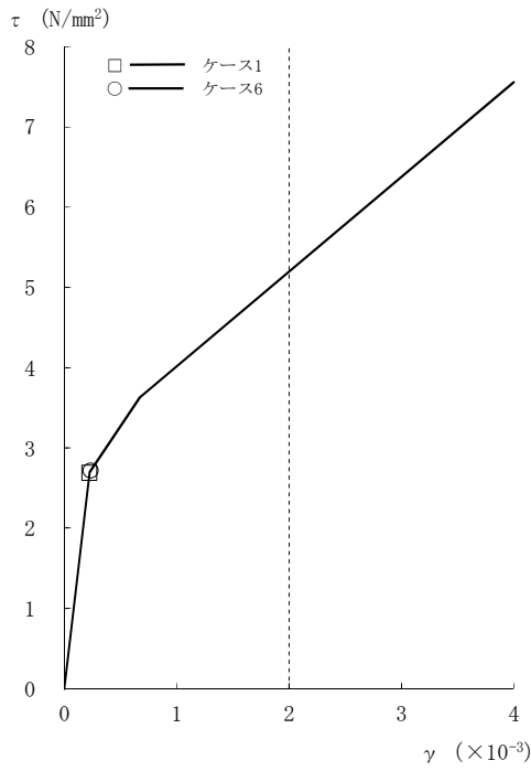
図2-101 τ - γ 関係と最大応答値 (Ss-2, NS方向, B2F) (7/8)
