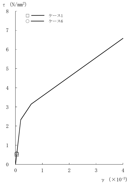
図2-121 \tau - \gamma 関係と最大応答値 (Sd-2, EW方向, CRF) (1/8)
