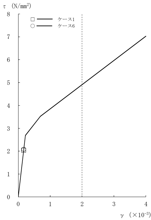
図2-101 τ - γ 関係と最大応答値 (Ss-2, NS方向, B3F) (8/8)
