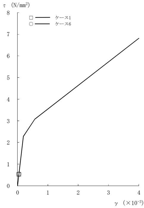
図2-117 \tau - \gamma 関係と最大応答値 (Sd-2, NS方向, CRF) (1/8)
