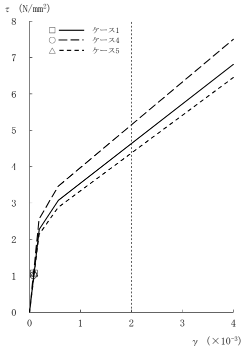
図2-61 \tau - \gamma 関係と最大応答値 (Ss-3, NS方向, CRF) (1/8)
