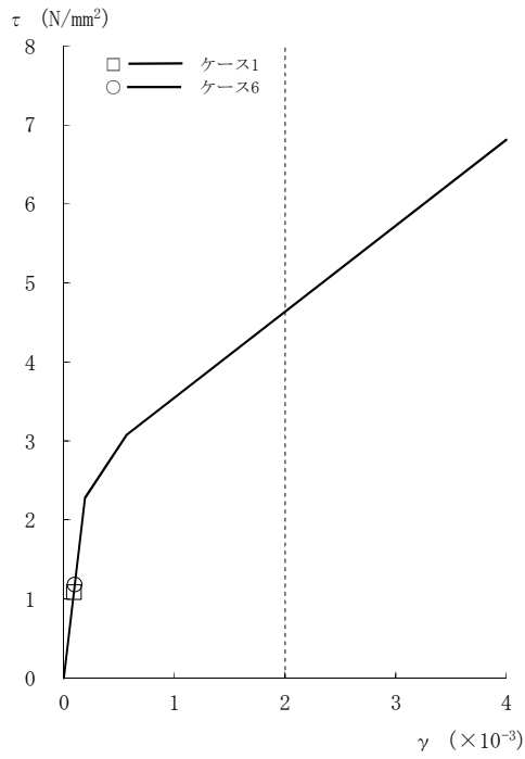
図2-101 τ - γ 関係と最大応答値 (Ss-2, NS方向, CRF) (1/8)
