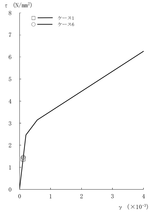
図2-119 τ - γ 関係と最大応答値 (Sd-8, NS方向, B2F) (7/8)
