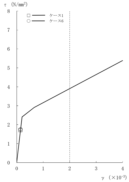
図2-106 τ - γ 関係と最大応答値 (Ss-3, EW方向, B2F) (7/8)
