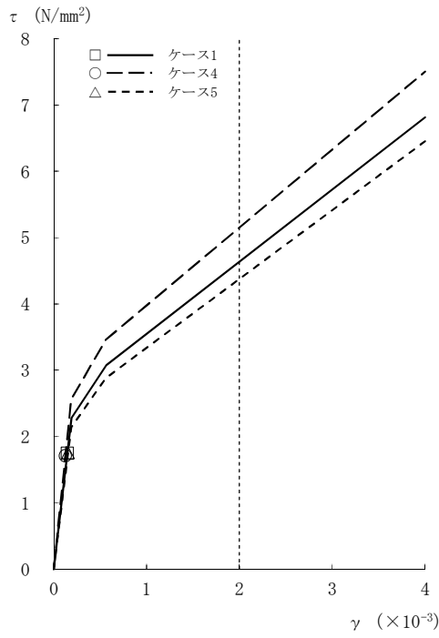
図2-59 \tau - \gamma 関係と最大応答値 (Ss-1, NS方向, CRF) (1/8)
