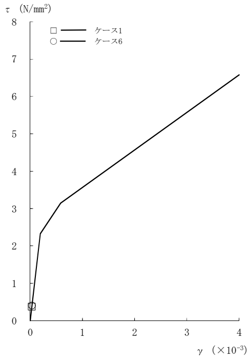
図2-122 \tau - \gamma 関係と最大応答値 (Sd-3, EW方向, CRF) (1/8)
