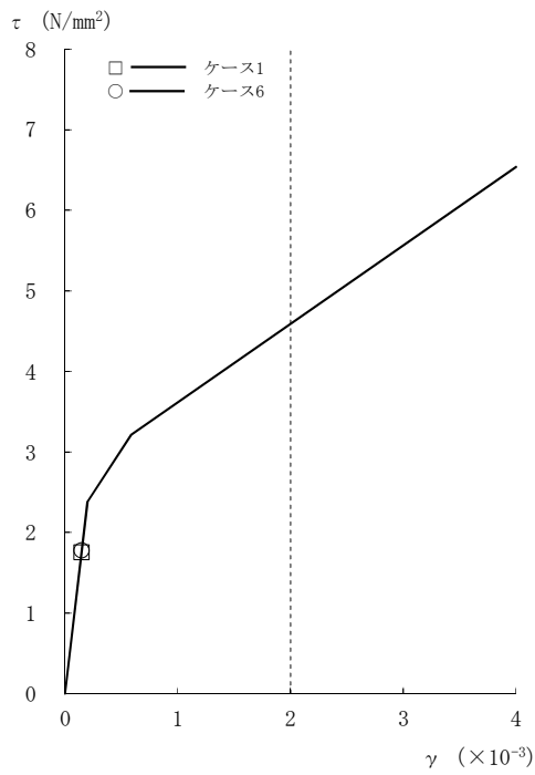
図2-103 τ - γ 関係と最大応答値 (Ss-8, NS方向, 4F) (2/8)
