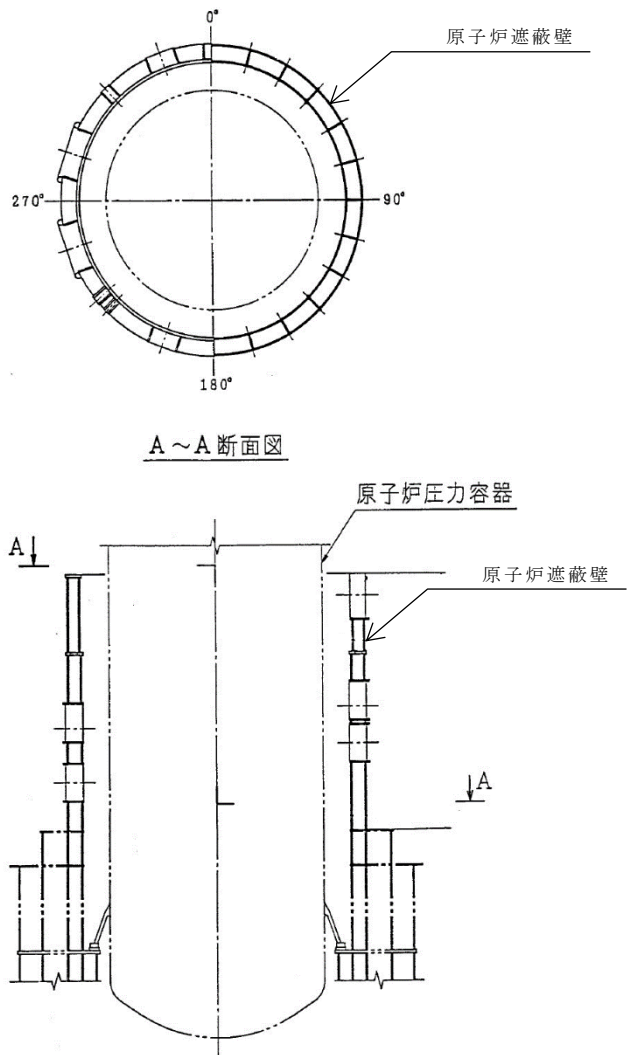
建設時工認 IV-4-6「原子炉しゃへい壁構造図」より抜粋
