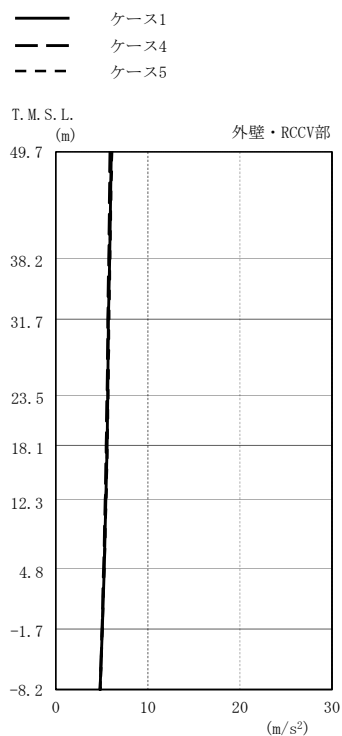
図2-53 最大応答加速度(基準地震動 S s , 鉛直方向)(1/2)
