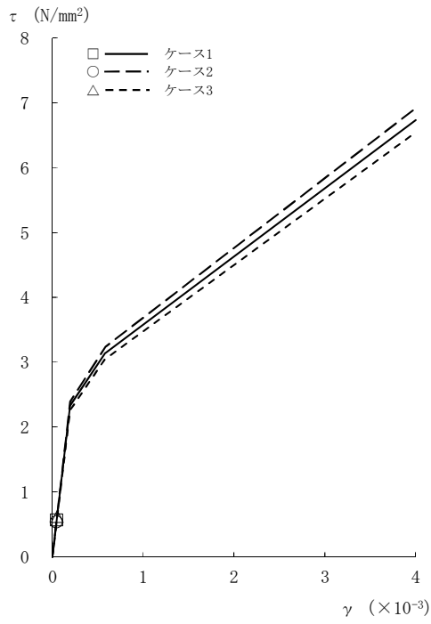
図2-44 \tau - \gamma 関係と最大応答値 (Sd-8, EW方向, CRF) (1/8)
