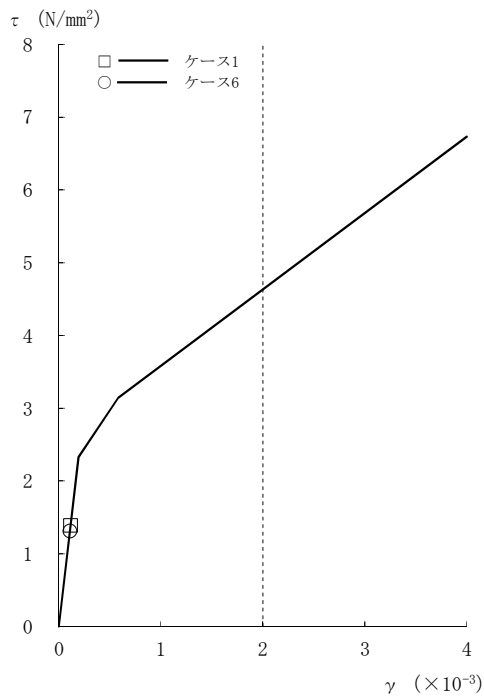
図2-104 τ - γ 関係と最大応答値 (Ss-1, EW方向, 4F) (2/8)
