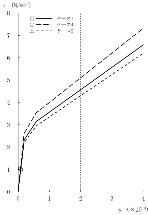
図2-64 τ - γ 関係と最大応答値 (Ss-2, EW方向, CRF) (1/8)
