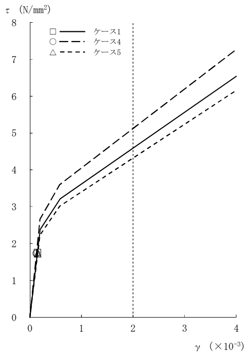
図2-62 τ - γ 関係と最大応答値 (S s -8, NS方向, 4F) (2/8)
