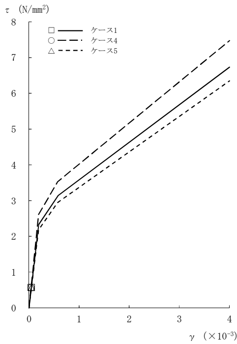
図2-85 \tau - \gamma 関係と最大応答値 (Sd-8, EW方向, 4F) (2/8)
