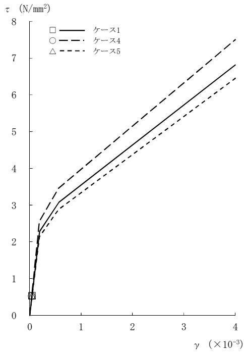
図2-79 \tau - \gamma 関係と最大応答値 (Sd-2, NS方向, CRF) (1/8)
