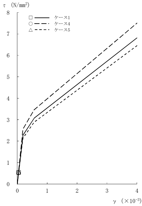
図2-80 \tau - \gamma 関係と最大応答値 (Sd-3, NS方向, CRF) (1/8)
