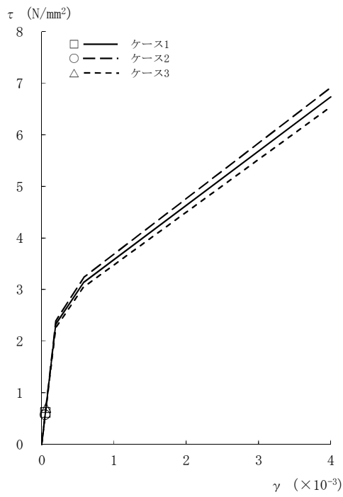
図2-42 \tau - \gamma 関係と最大応答値 (Sd-2, EW方向, 4F) (2/8)
