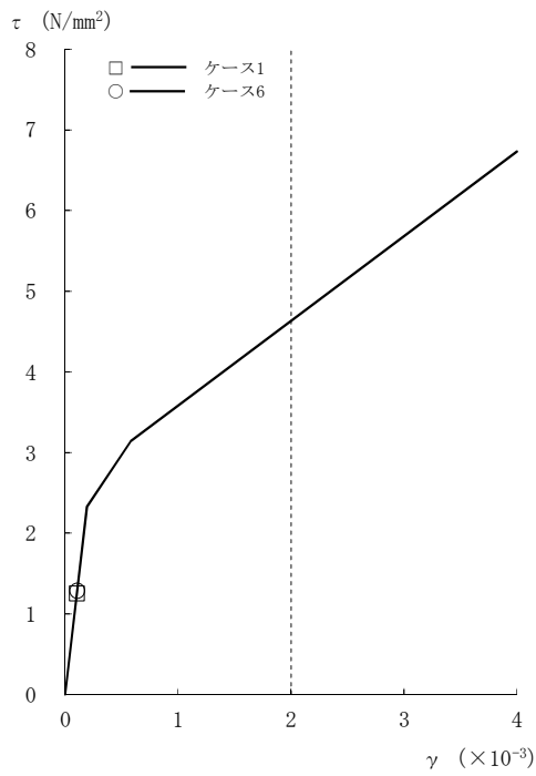
図2-105 τ - γ 関係と最大応答値 (Ss-2, EW方向, 4F) (2/8)
