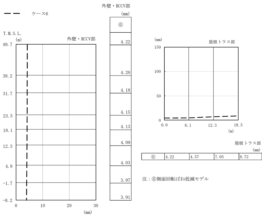
図2-98 最大応答変位 (基準地震動 S_s , EW方向, 誘発上下動) (2/2)
