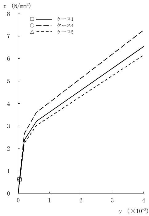
図2-79 \tau - \gamma 関係と最大応答値 (Sd-2, NS方向, 4F) (2/8)
