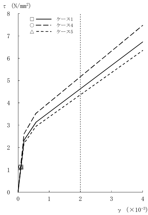
図2-66 \tau - \gamma 関係と最大応答値 (Ss-8, EW方向, 4F) (2/8)
