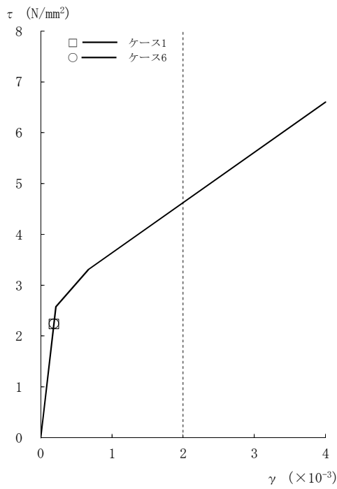
図2-106 τ - γ 関係と最大応答値 (Ss-3, EW方向, B3F) (8/8)
