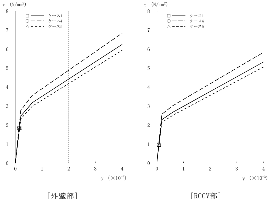
図2-65 \tau - \gamma 関係と最大応答値 (Ss-3, EW方向, 1F) (5/8)
