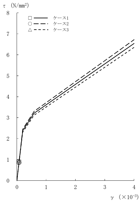
図2-40 \tau - \gamma 関係と最大応答値 (Sd-8, NS方向, 4F) (2/8)
