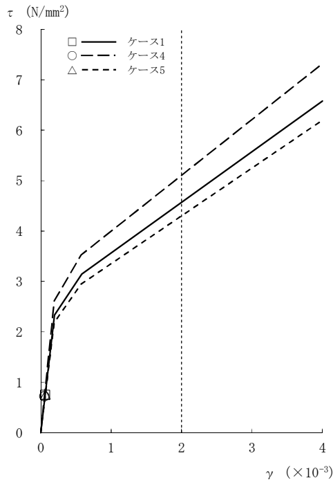
図2-65 \tau - \gamma 関係と最大応答値 (Ss-3, EW方向, CRF) (1/8)
