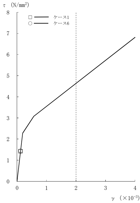
図2-103 τ - γ 関係と最大応答値 (Ss-8, NS方向, CRF) (1/8)
