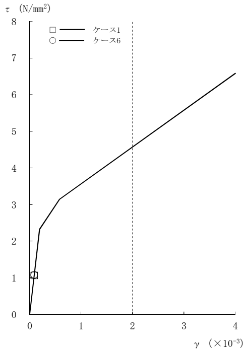
図2-105 τ - γ 関係と最大応答値 (Ss-2, EW方向, CRF) (1/8)
