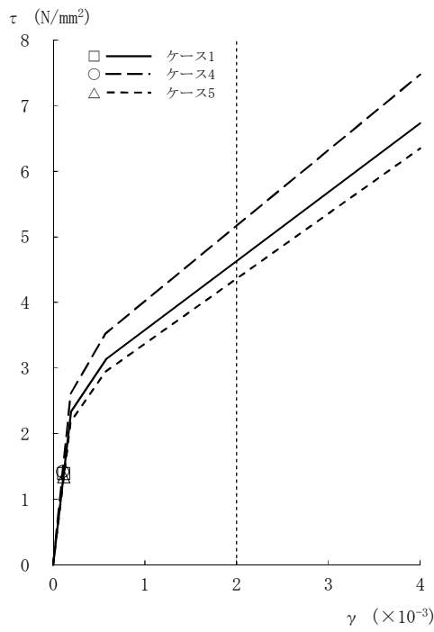
図2-63 \tau - \gamma 関係と最大応答値 (Ss-1, EW方向, 4F) (2/8)
