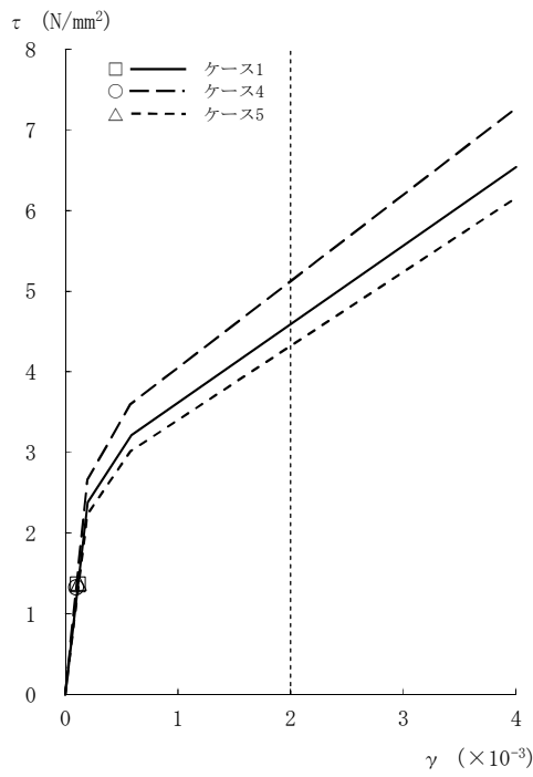
図2-60 \tau - \gamma 関係と最大応答値 (S s -2, NS方向, 4F) (2/8)
