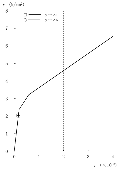
図2-100 \tau - \gamma 関係と最大応答値 (Ss-1, NS方向, 4F) (2/8)
