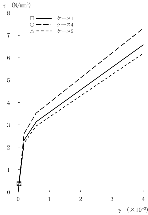
図2-84 \tau - \gamma 関係と最大応答値 (Sd-3, EW方向, CRF) (1/8)
