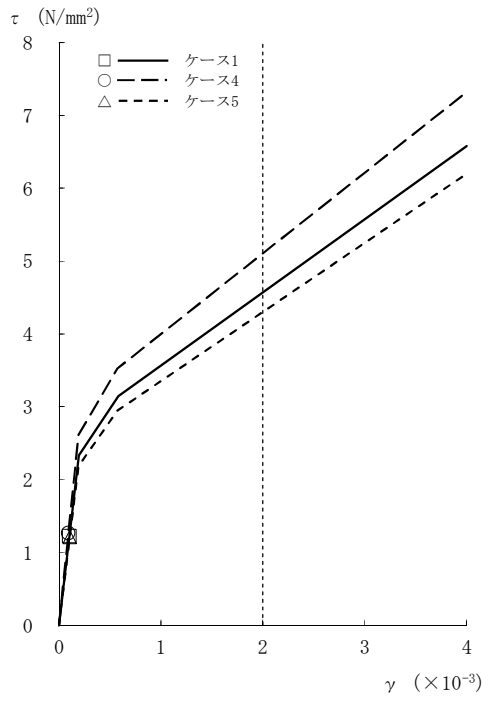
図2-63 \tau - \gamma 関係と最大応答値 (Ss-1, EW方向, CRF) (1/8)
