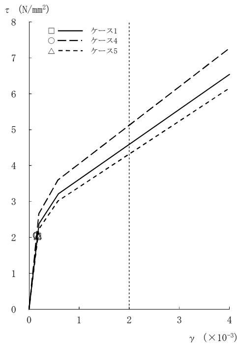
図2-59 \tau - \gamma 関係と最大応答値 (Ss-1, NS方向, 4F) (2/8)
