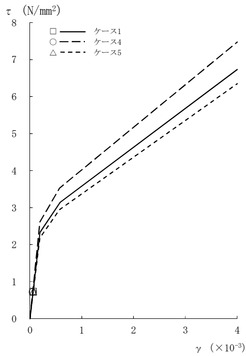
図2-82 τ - γ 関係と最大応答値 (Sd-1, EW方向, 4F) (2/8)
