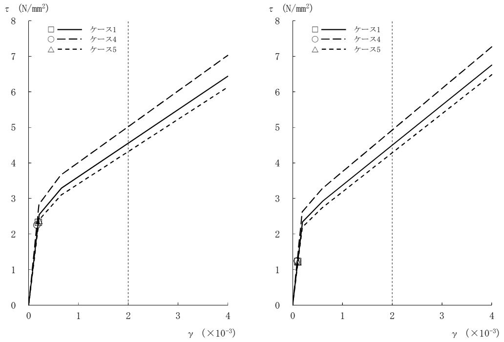
図2-61 \tau - \gamma 関係と最大応答値 (Ss-3, NS方向, 1F) (5/8)
