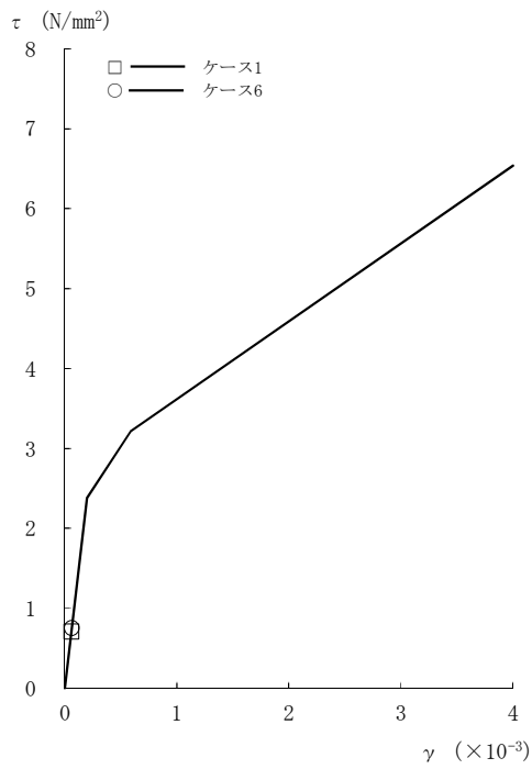
図2-118 \tau - \gamma 関係と最大応答値 (Sd-3, NS方向, 4F) (2/8)
