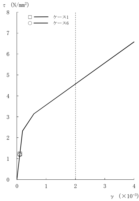
図2-104 τ - γ 関係と最大応答値 (Ss-1, EW方向, CRF) (1/8)
