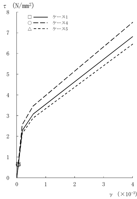
図2-81 \tau - \gamma 関係と最大応答値 (Sd-8, NS方向, CRF) (1/8)
