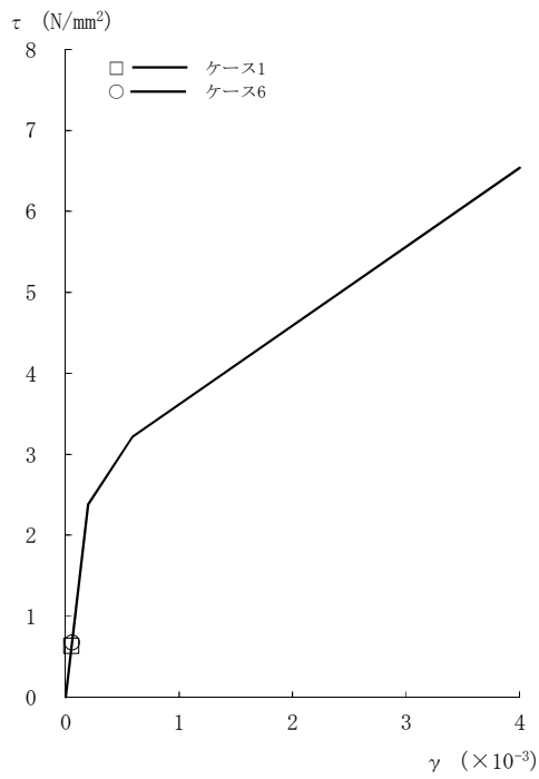
図2-117 \tau - \gamma 関係と最大応答値 (Sd-2, NS方向, 4F) (2/8)
