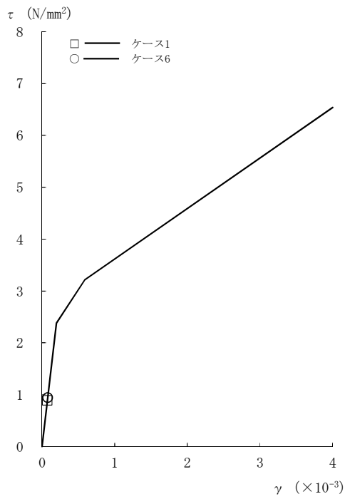
図2-119 τ - γ 関係と最大応答値 (Sd-8, NS方向, 4F) (2/8)
