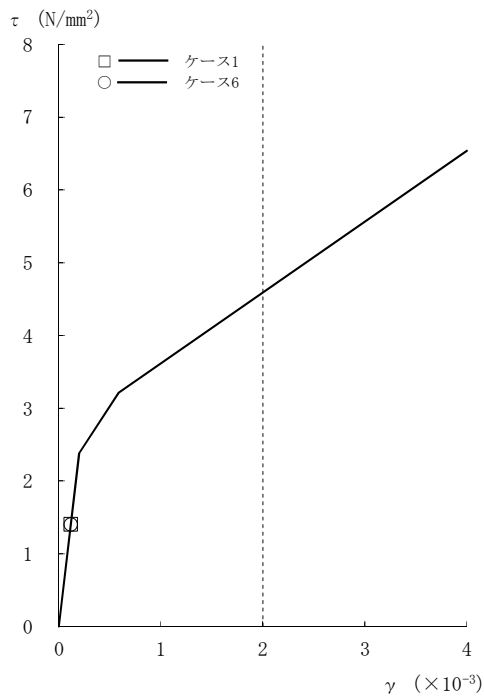
図2-102 τ - γ 関係と最大応答値 (Ss-3, NS方向, 4F) (2/8)
