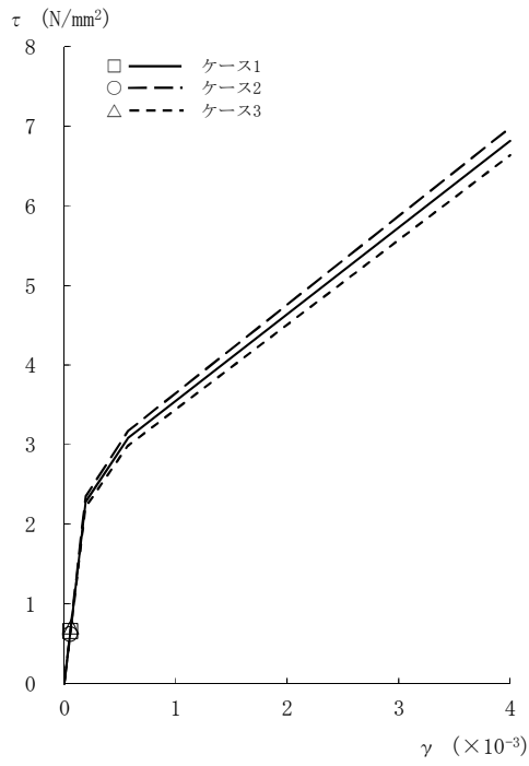
図2-40 \tau - \gamma 関係と最大応答値 (Sd-8, NS方向, CRF) (1/8)
