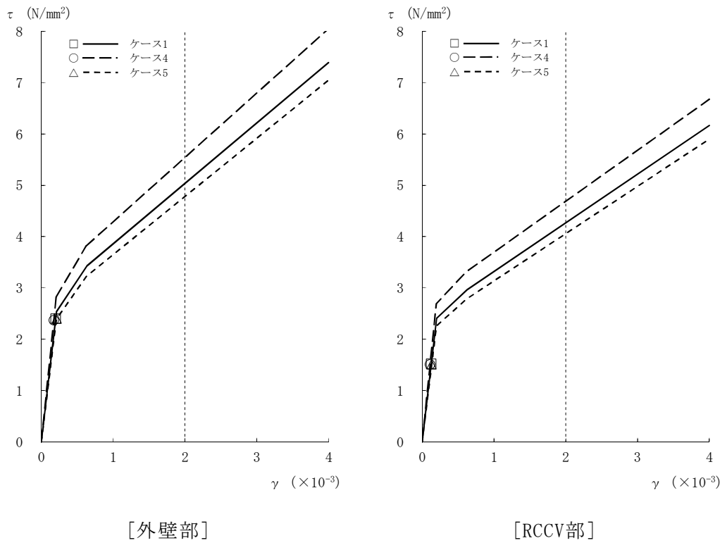
図2-65 \tau - \gamma 関係と最大応答値 (Ss-3, EW方向, B1F) (6/8)
