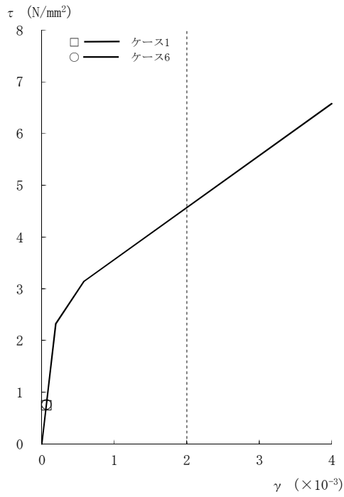
図2-106 τ - γ 関係と最大応答値 (Ss-3, EW方向, CRF) (1/8)
