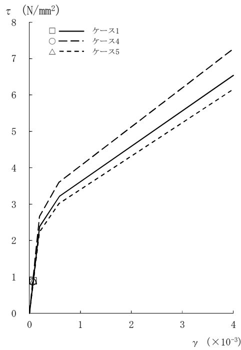
図2-81 \tau - \gamma 関係と最大応答値 (Sd-8, NS方向, 4F) (2/8)
