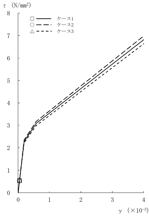
図2-39 \tau - \gamma 関係と最大応答値 (Sd-3, NS方向, CRF) (1/8)
