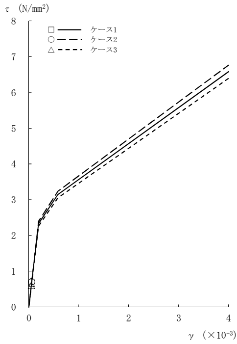
図2-41 \tau - \gamma 関係と最大応答値 (Sd-1, EW方向, CRF) (1/8)
