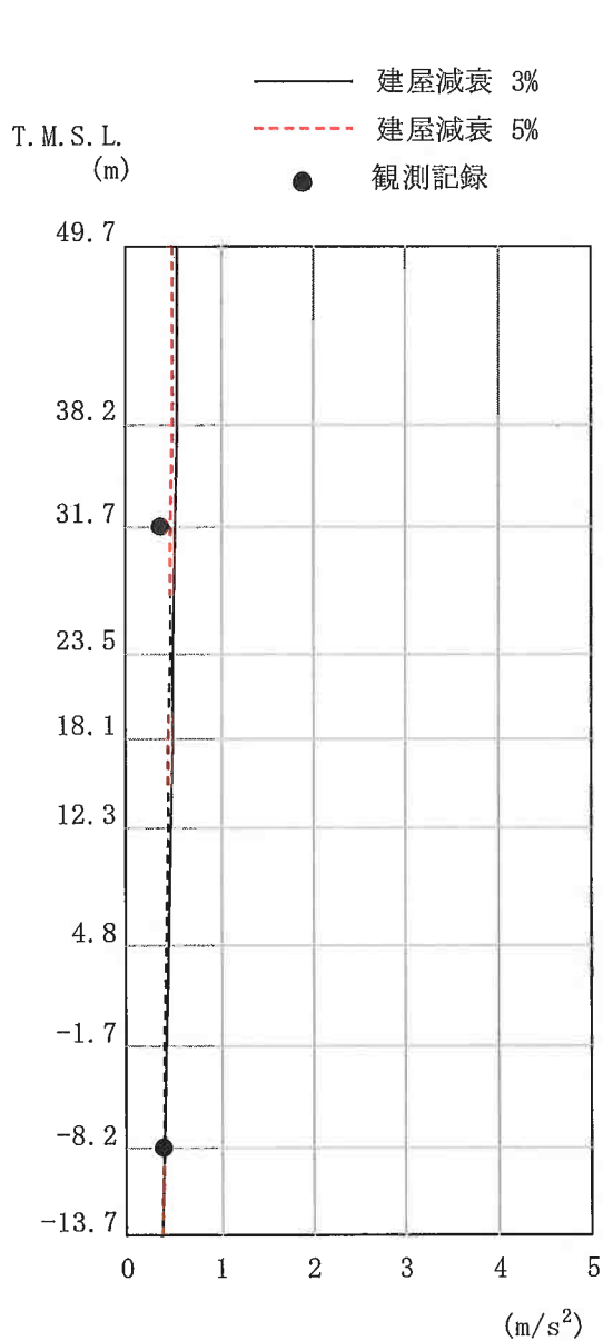
図 2-1 最大応答加速度分布の比較 (鉛直方向) : 中越地震 (余震) 観測記録 (3/3)
