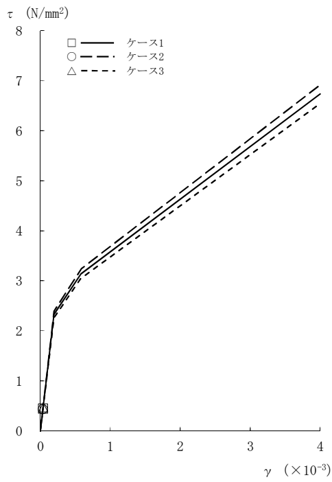
図2-43 \tau - \gamma 関係と最大応答値 (Sd-3, EW方向, 4F) (2/8)
