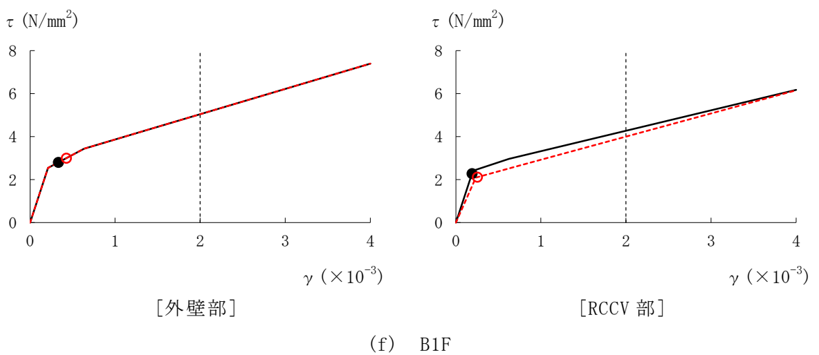
図 3-18 せん断スケルトン曲線上の最大応答値 (Ss-1, EW 方向) (2/3)
