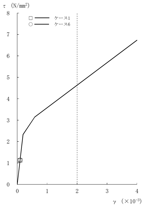
図2-107 \tau - \gamma 関係と最大応答値 (Ss-8, EW方向, 4F) (2/8)
