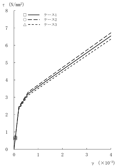
図2-38 \tau - \gamma 関係と最大応答値 (Sd-2, NS方向, 4F) (2/8)
