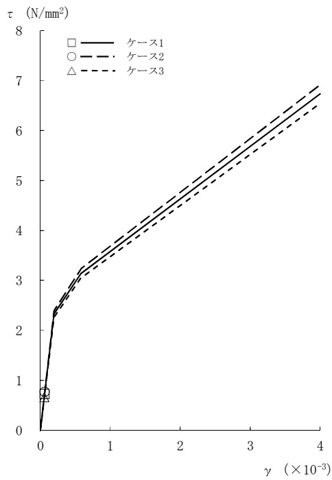
図2-41 \tau - \gamma 関係と最大応答値 (Sd-1, EW方向, 4F) (2/8)
