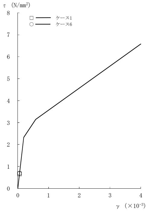
図2-120 \tau - \gamma 関係と最大応答値 (Sd-1, EW方向, CRF) (1/8)
