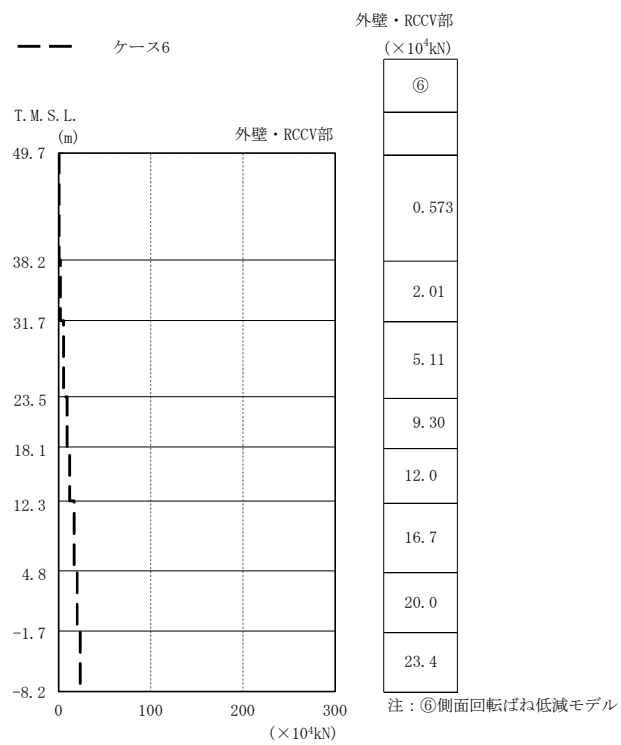
図2-99 最大応答軸力（基準地震動 S s , EW方向, 誘発上下動）(2/2)
