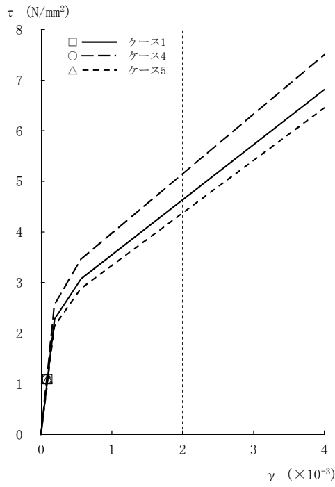
図2-60 \tau - \gamma 関係と最大応答値 (S s -2, NS方向, CRF) (1/8)
