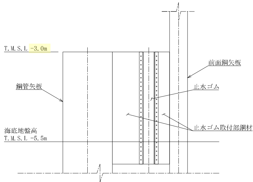
図 2.6-3-18 海水貯留堰（6号機設備）接続部の構造概念図
