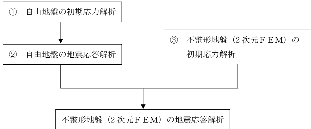
図 2.5-3-8 自由地盤の初期応力解析から不整形地盤（2次元FEM）の地震応答解析までのフロー
