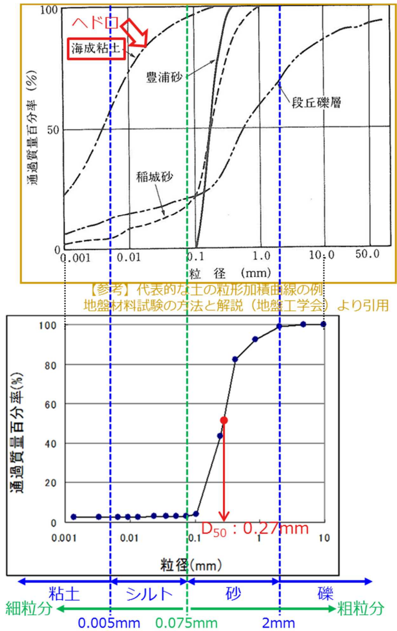
図 3.1-参 1-5 代表的な土の粒形加積曲線の例と 発電所港湾内の底質土砂の粒形加積曲線の比較
