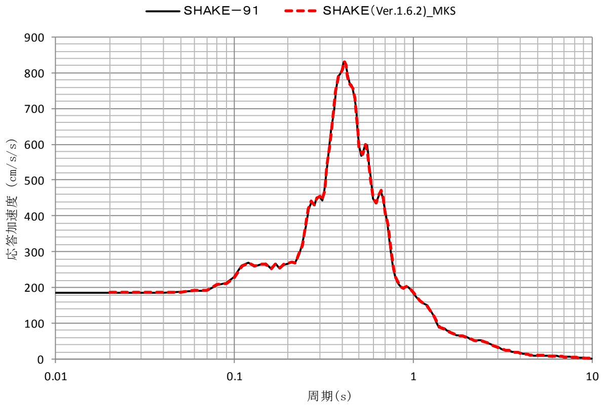
図 3-10 地表の加速度応答スペクトル (h=0.05)
