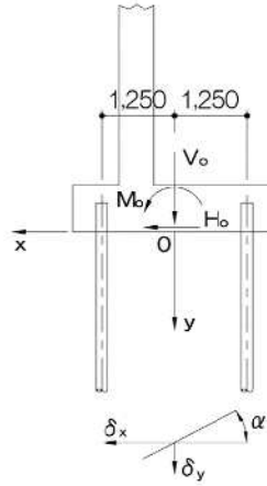
図 3-12 変位法による計算座標
