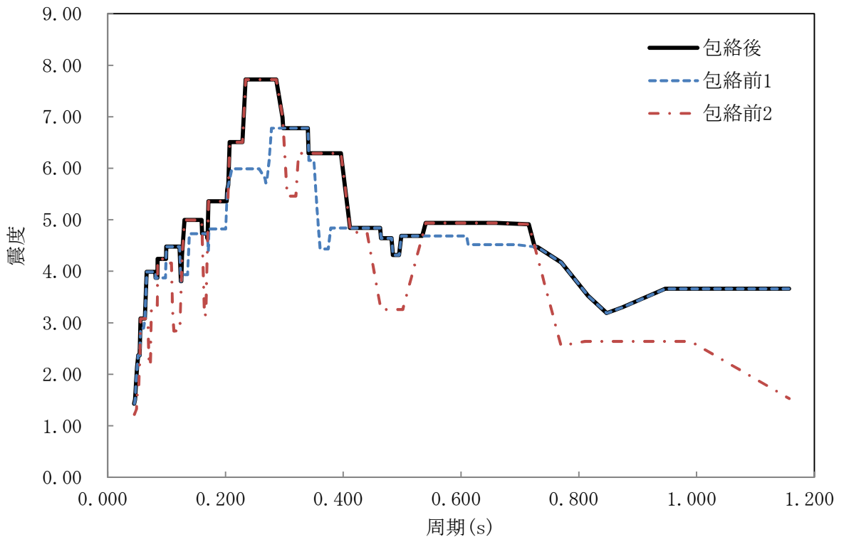
図 3.5-4 包絡結果
