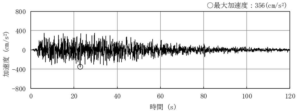
(a) 加速度波形
