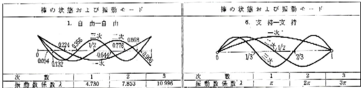
図 3-7 一様断面はりの横振動（出典：機械工学便覧）
