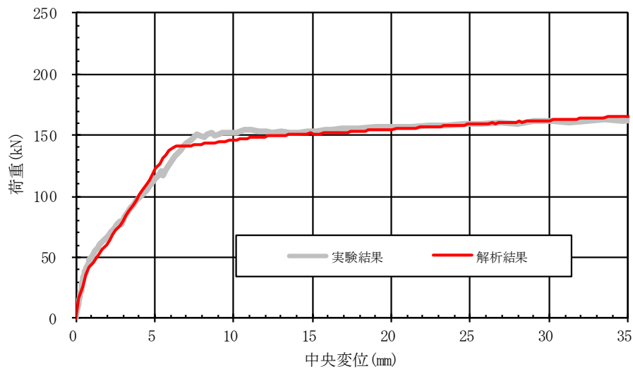
図 3-7 荷重－変位関係の比較
