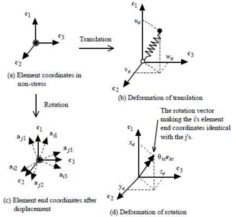
図 3-1 ばね要素の要素変形と要素座標系
