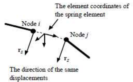
図 3-3 2 重節点
