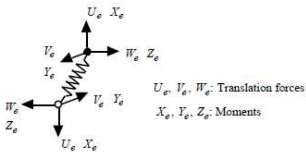
図 3-2 ばね要素の要素端力
