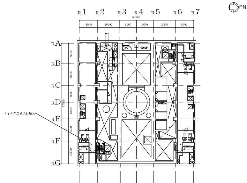
図16 機器配置図 (原子炉建屋地上中3階)
