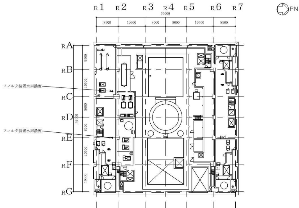
図17 機器配置図 (原子炉建屋地上3階)
