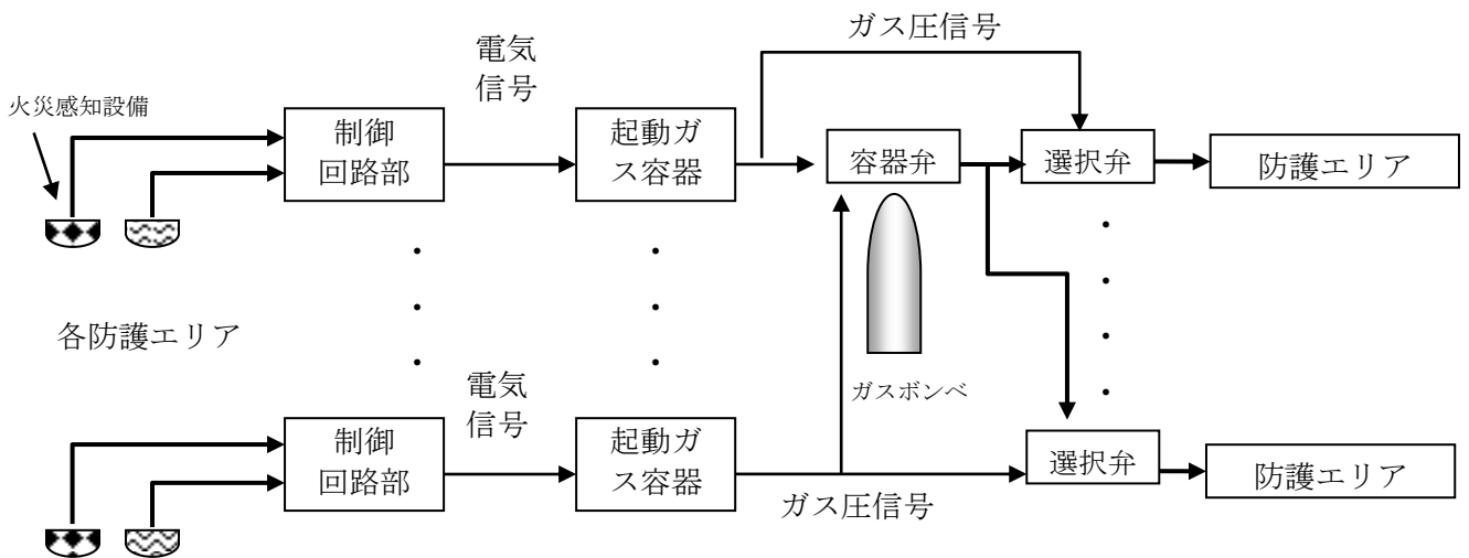
第4図 二酸化炭素消火設備の系統構成
