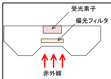
図 火災感知器の原理
