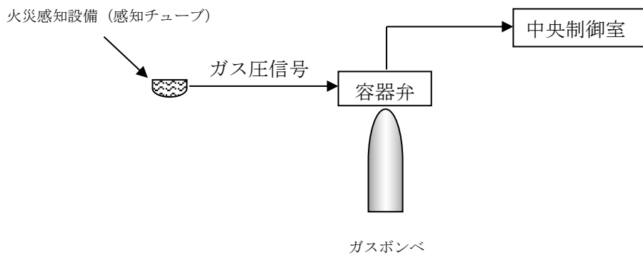
第2図 ケーブルトレイ消火設備の系統構成
