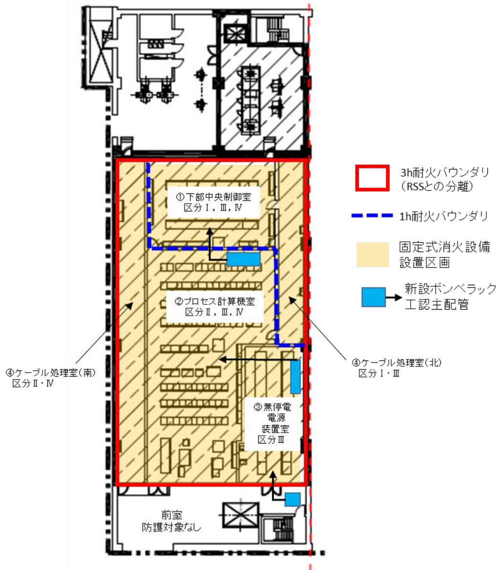
図1 下部中央制御室の火災防護対策
