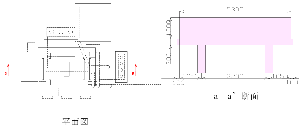
(c) 予備変圧器の基礎構造
