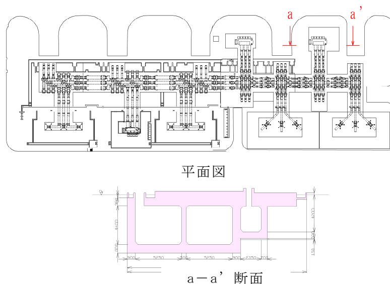
(a) 500kV 超高圧開閉所基礎構造図
