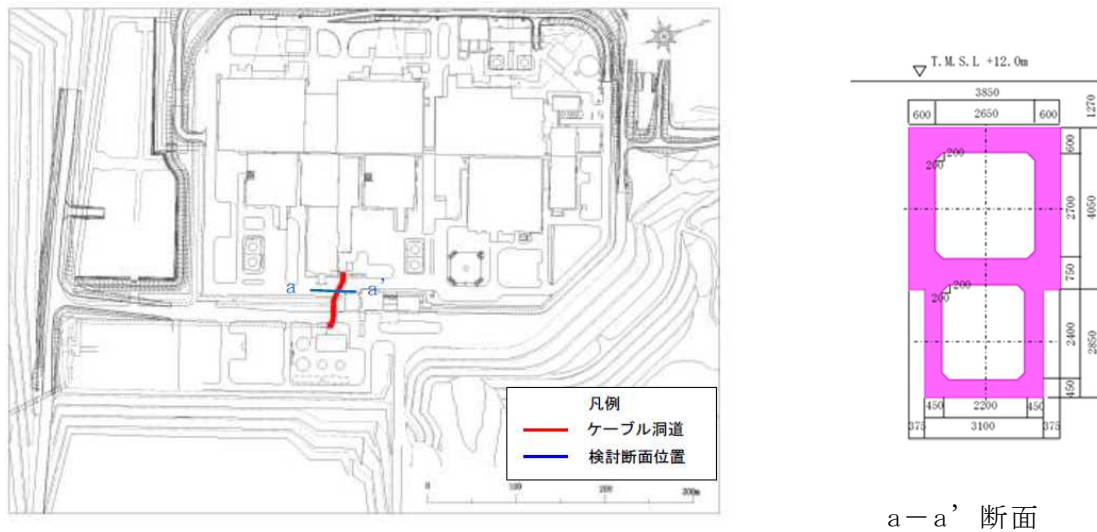
(d) 6号機 CV ケーブル洞道位置図・断面図
