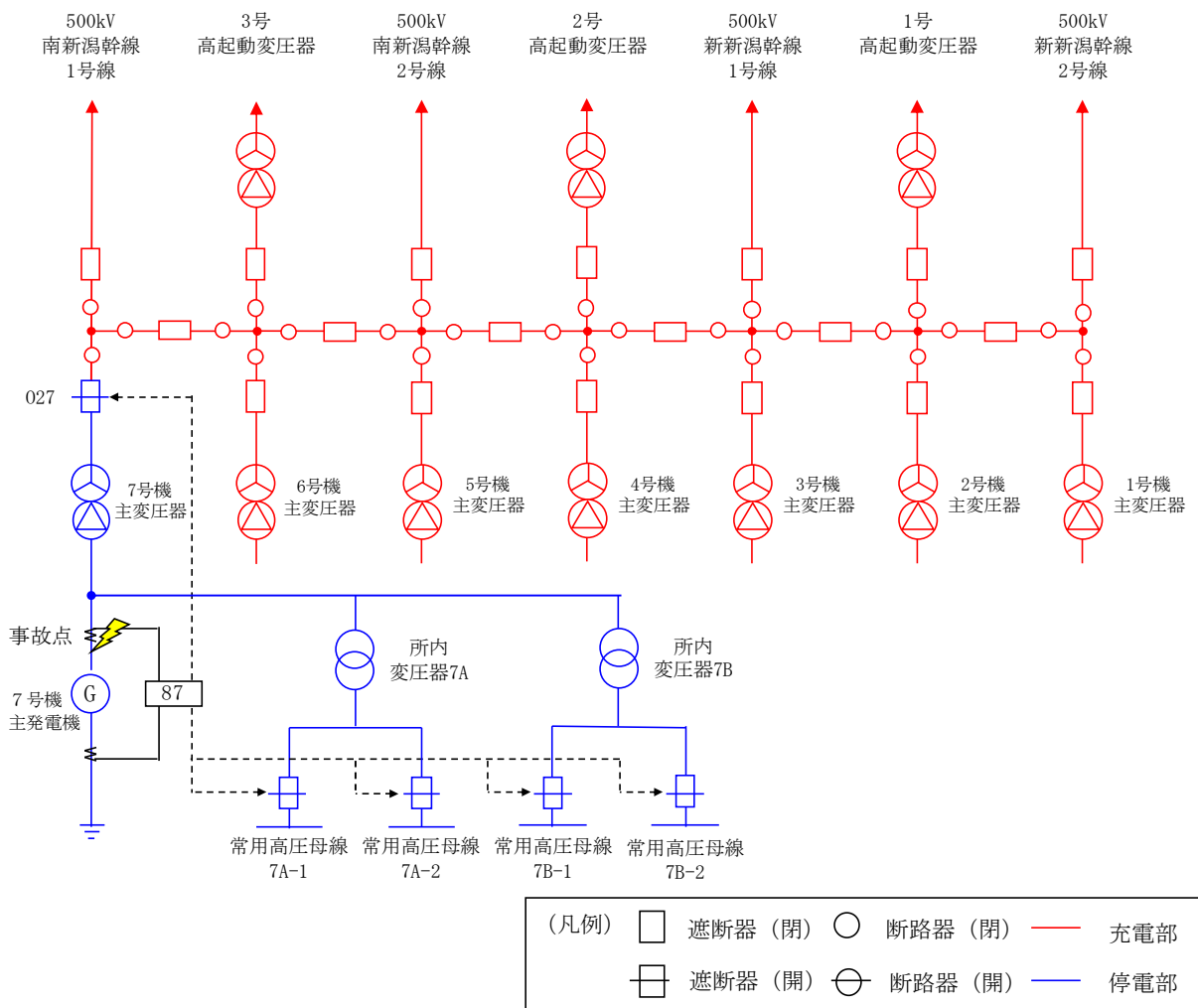
図 7 発電機保護
