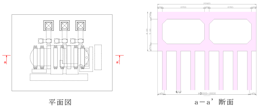
(a) 主変圧器の基礎構造
