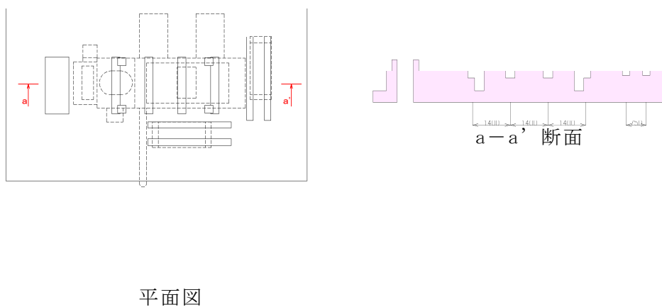
(b) 低起動変圧器の基礎構造
