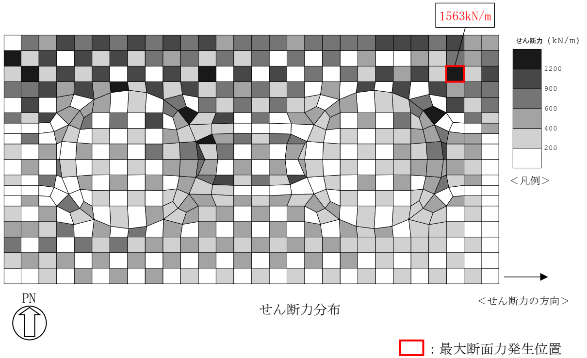
図 4-2 (2) 鉄筋コンクリート部材のせん断力照査値最大時の断面力分布図 (解析ケース③, Ss-8++, t=8.12s)
