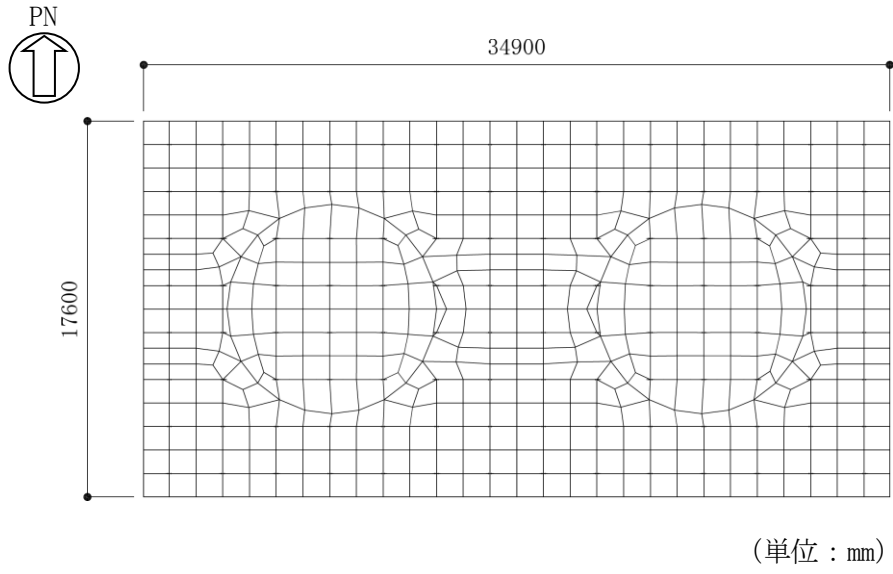
図 3-4 要素分割図
