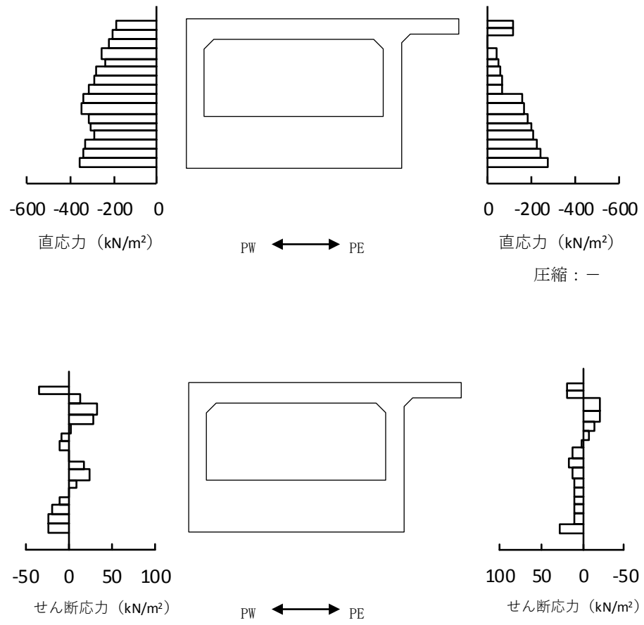
図 3-9 (2) 第一ガスタービン発電機用燃料タンク基礎の作用荷重分布図 (EW 断面, 解析ケース①, Ss-1-)
