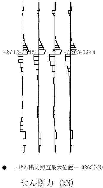
図 4-6 (1) 鋼管杭のせん断力照査値最大時の断面力分布図 (A-A断面, 解析ケース②, Ss-3++, t=17.71s)
