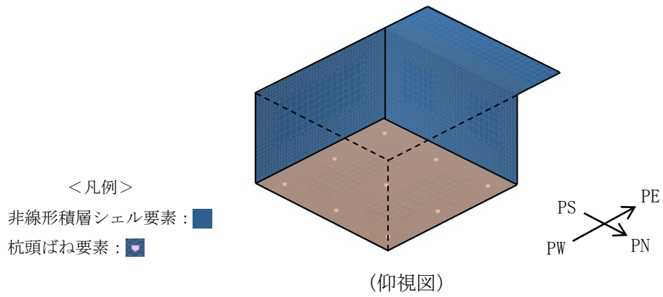
図 3-5 第一ガスタービン発電機用燃料タンク基礎モデル概念図
