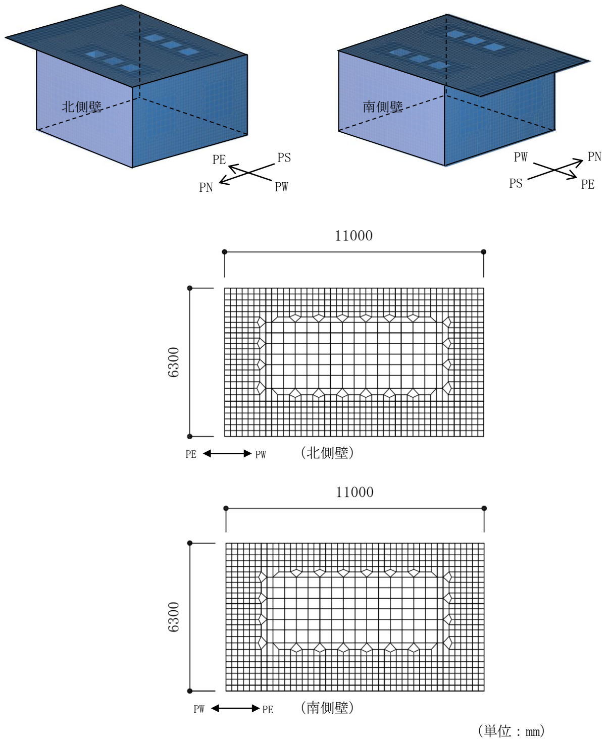
図 3-6 (3) 第一ガスタービン発電機用燃料タンク 基礎要素分割図
