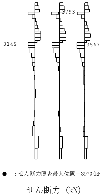
図 4-6 (2) 鋼管杭のせん断力照査値最大時の断面力分布図 (B-B断面, 解析ケース①, Ss-3++, t=17.89s)
