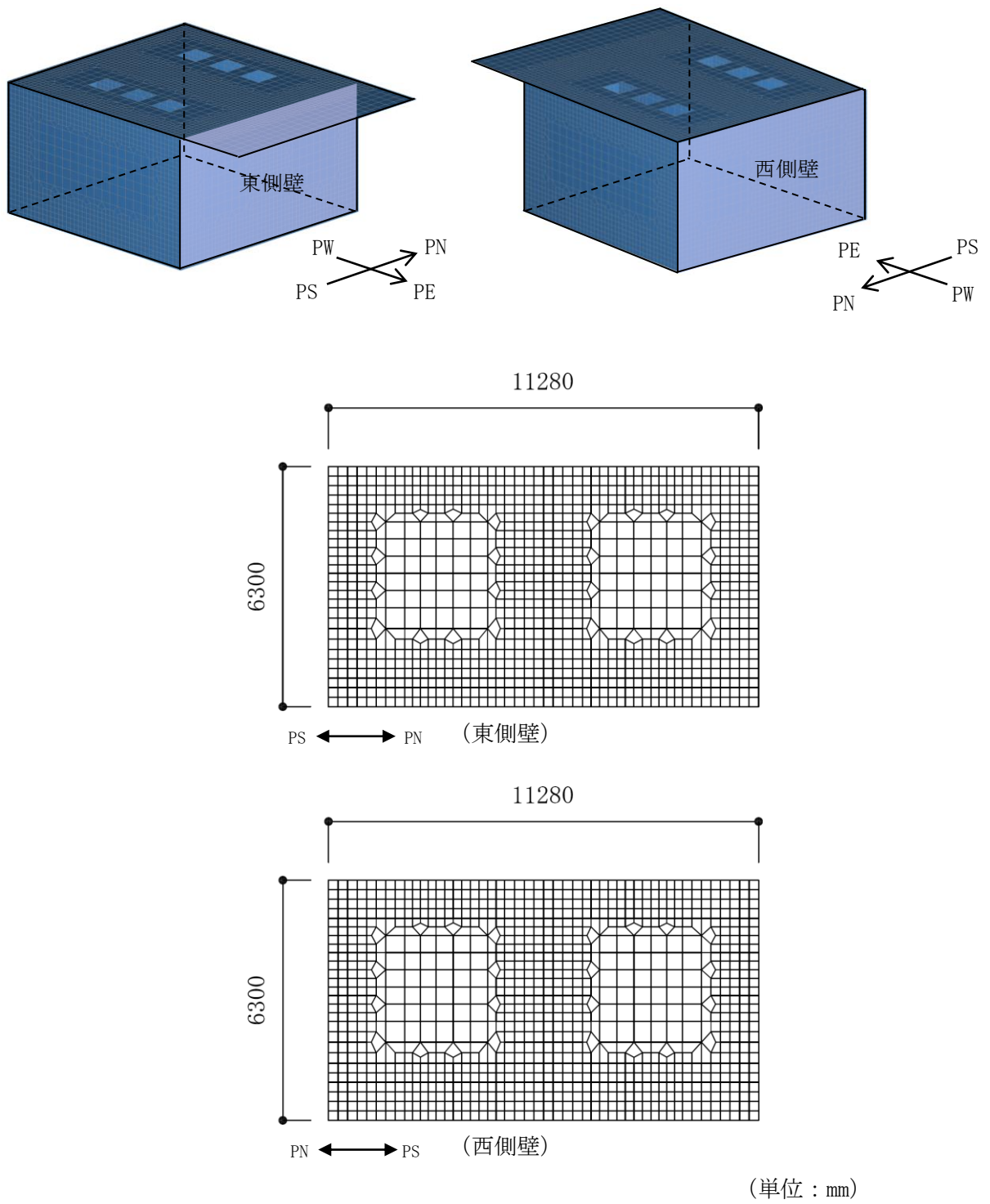
図 3-6 (2) 第一ガスタービン発電機用燃料タンク基礎要素分割図
