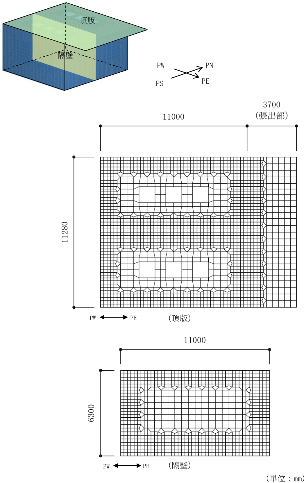
図 3-6 (1) 第一ガスタービン発電機用燃料タンク基礎要素分割図
