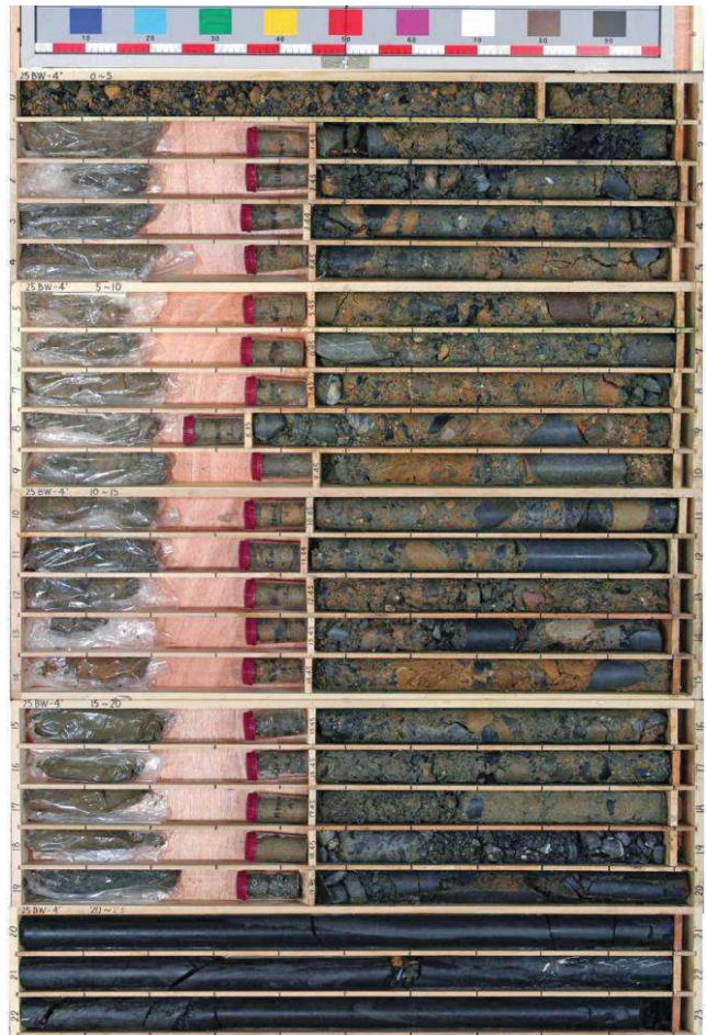
図 1.1-6 ボーリング柱状図・コア写真 (25BW-4)
