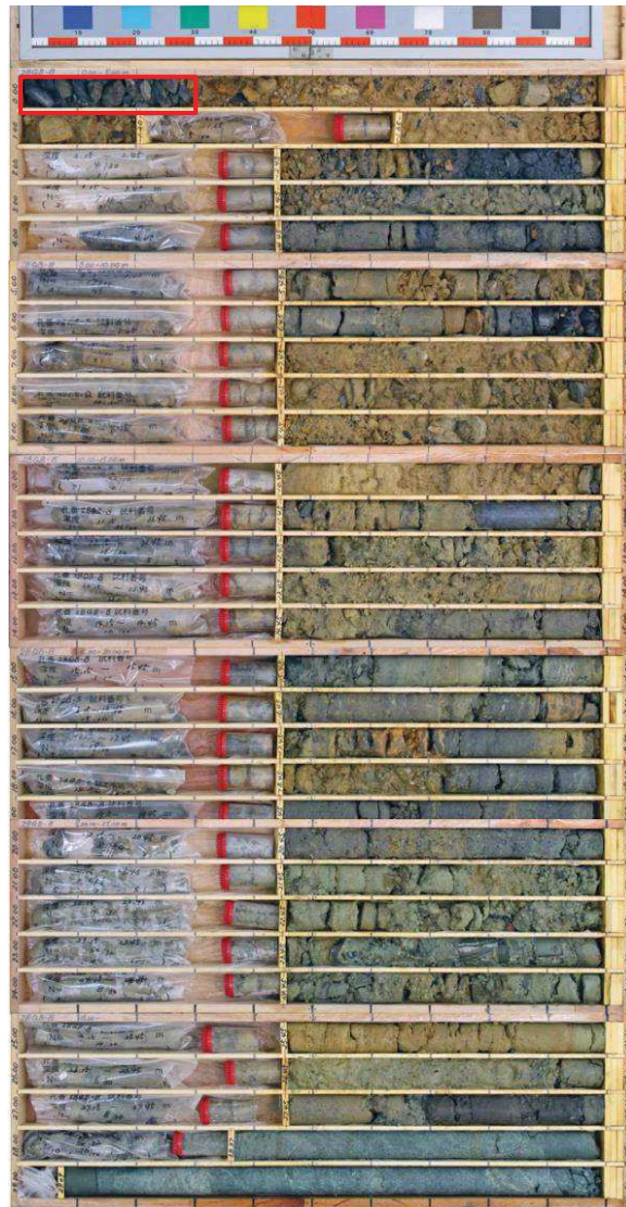
図 1.1-35 ボーリング柱状図・コア写真 (28QB-8)
