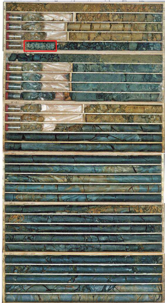
図 1.2-22 ボーリング柱状図・コア写真 (SP-2)
