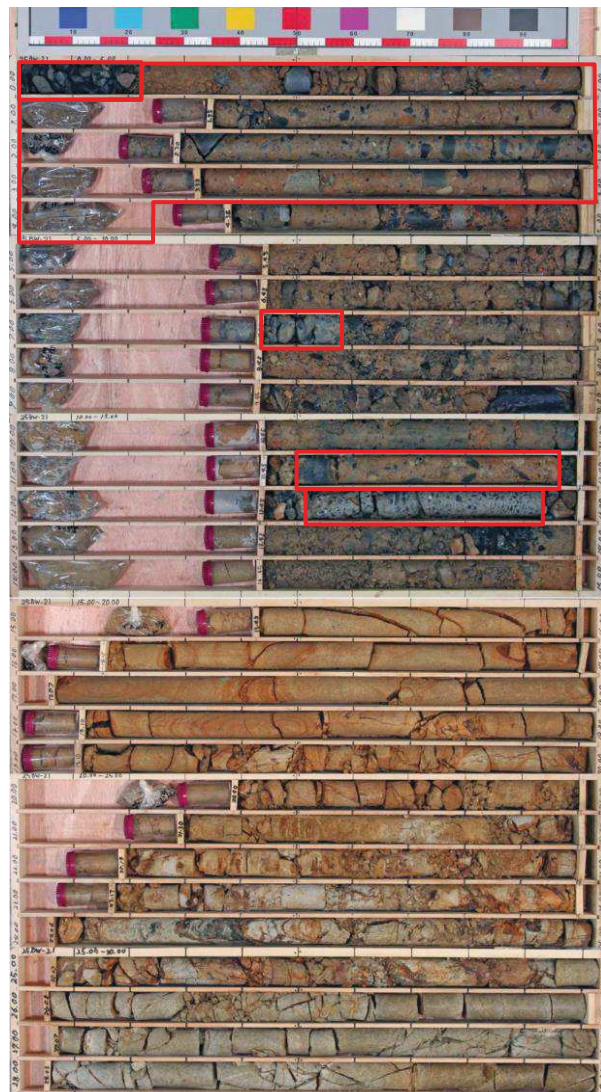
図 1.2-12 ボーリング柱状図・コア写真 (25BW-21)
