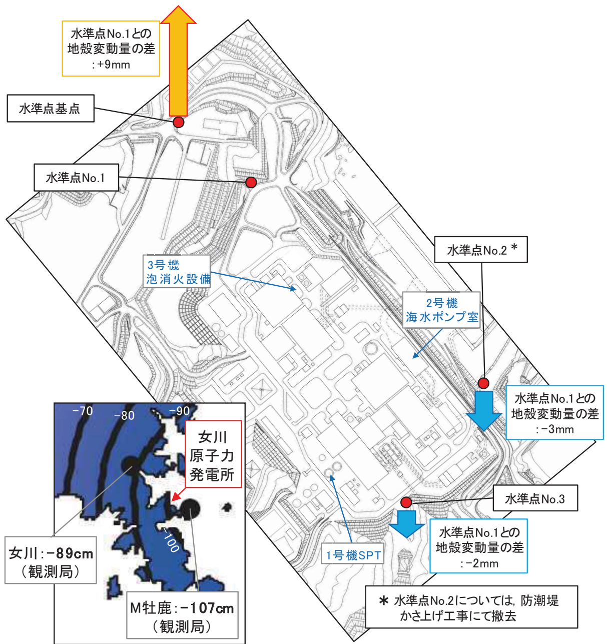
図 2-21 水准点 No. 1 に対する地殻変動量の差
