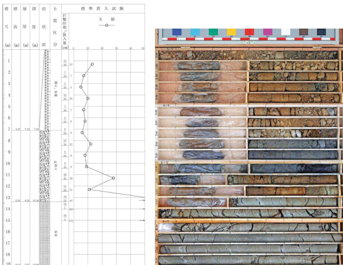
図 1.2-34 ボーリング柱状図・コア写真 (B-9)
