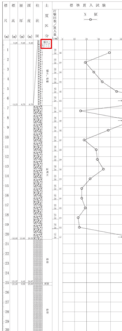
図 1.2-21 ボーリング柱状図・コア写真 (P-6)
