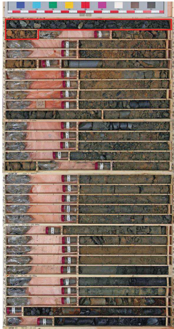
図 1.1-11 ボーリング柱状図・コア写真 (25BW-10)
