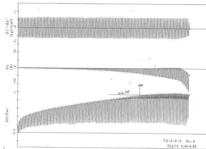
図 2.2-8 液状化強度試験結果 (A-1-2 試料 (供試体 No. 4) )
