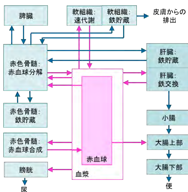
図 C1 鉄の組織系動態モデル
