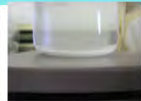
共沈
