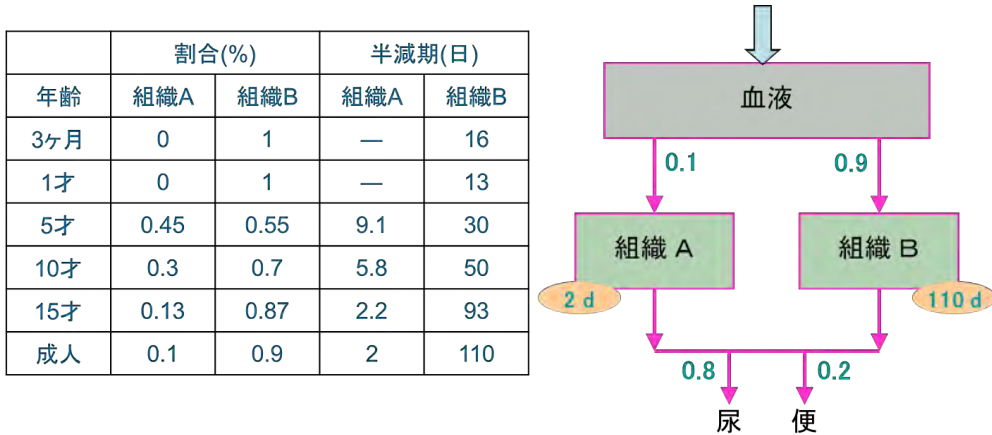
図 C4 セシウムの組織系動態モデル
