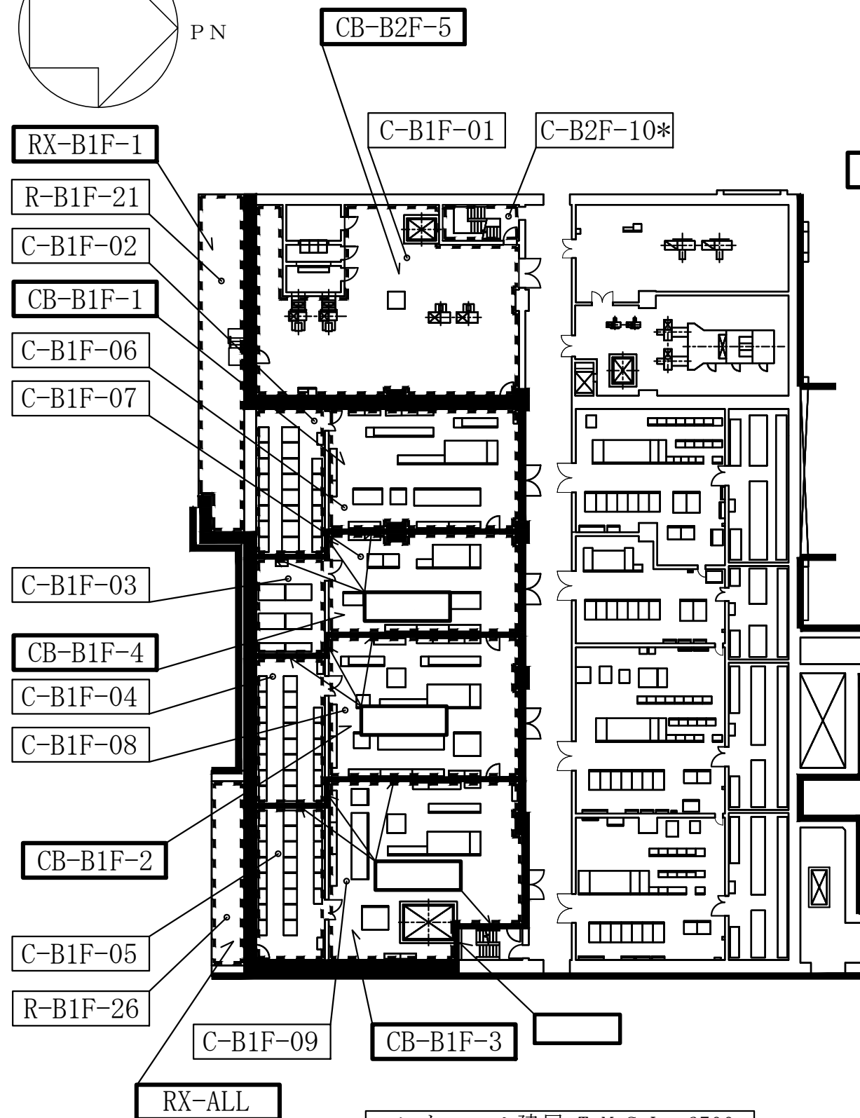
コントロール建屋 T.M.S.L. 6500
