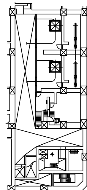
原子炉建屋 T.M.S.L. 23500
