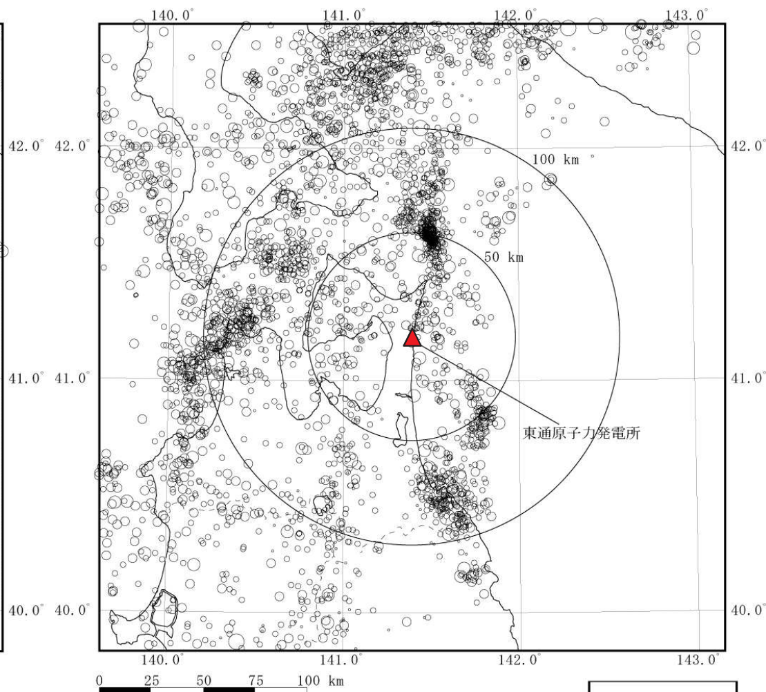
震源深さ 100km以深
