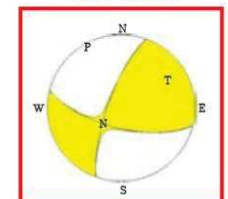
今回の地震の最大余震の発震機構 (USGSのCMT解)
