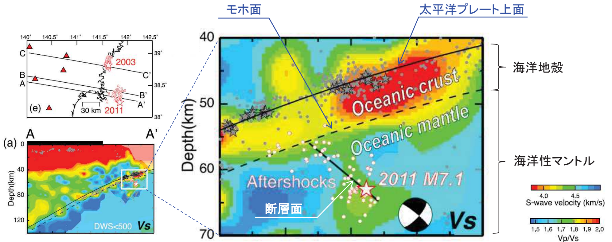
4.7地震震源域の鉛直分布図〔Nakajima et al.(2011)一部加筆〕
