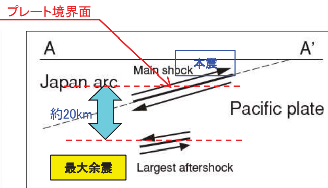
推定された断層面(断面)
