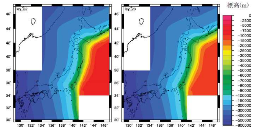
第22層 海洋地殻 (Vs(β)=3.5km/s)
