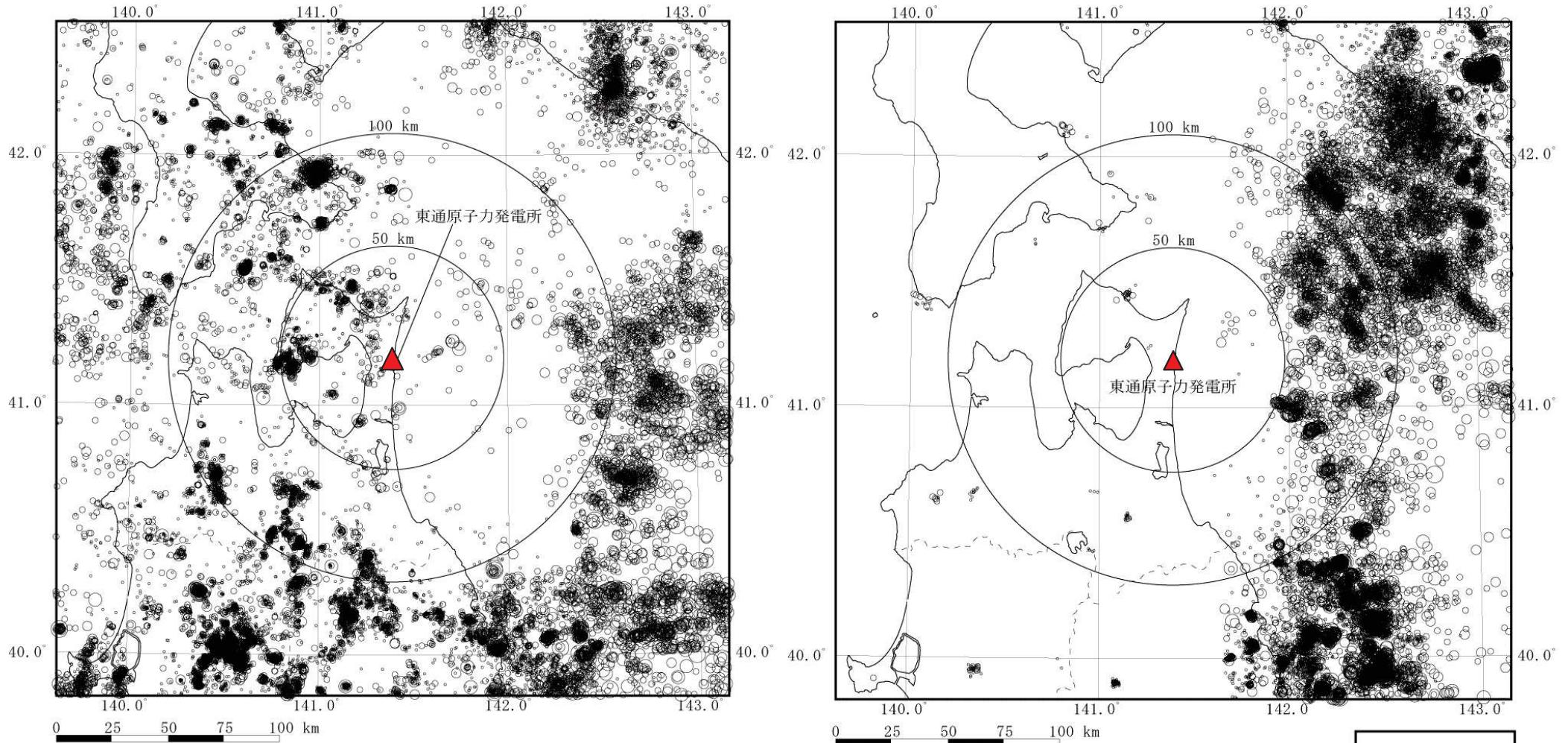
震源深さ 0~30km
