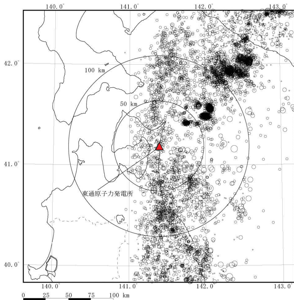
震源深さ 60~100km
