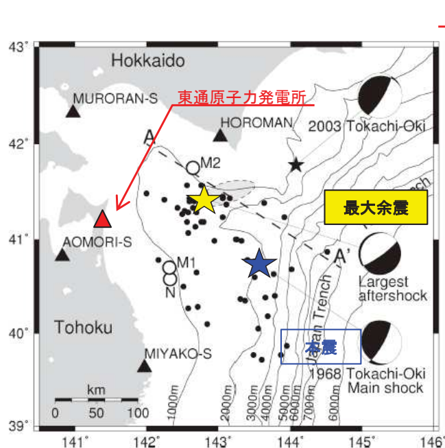
本震と最大余震の震央分布
