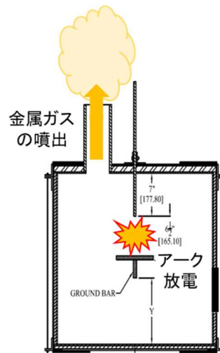
図1 HEAF時の金属蒸気噴出評価の模式図
