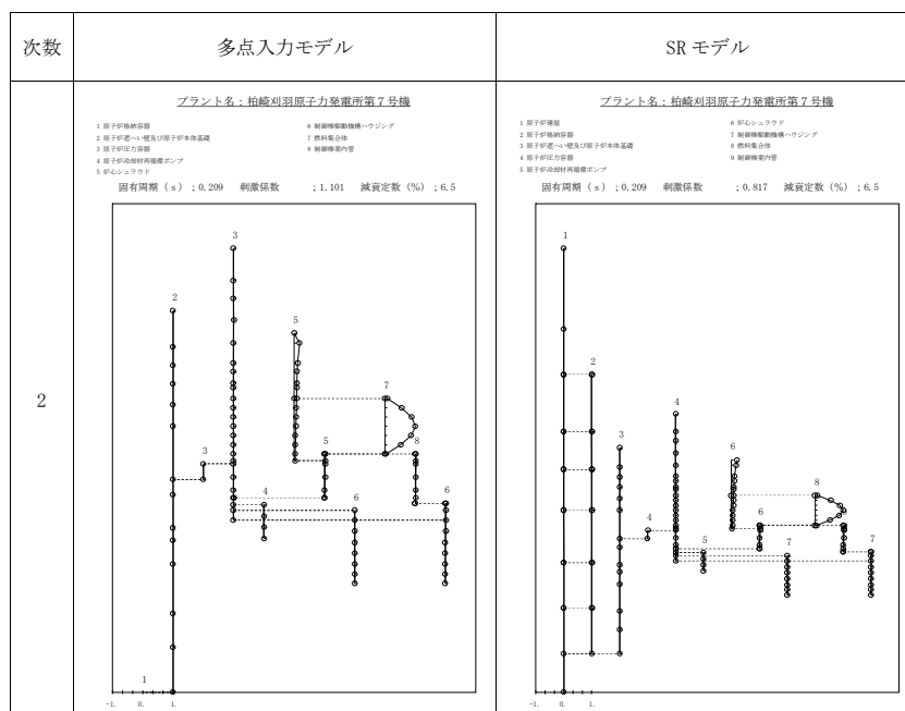
図添 9-2 振動モードの比較 (Sd-1, EW 方向) (2/11)
