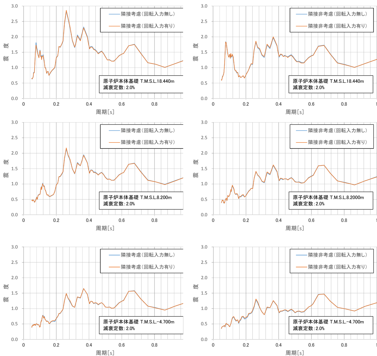
図添 6-2 回転入力の影響 (床応答スペクトル)
