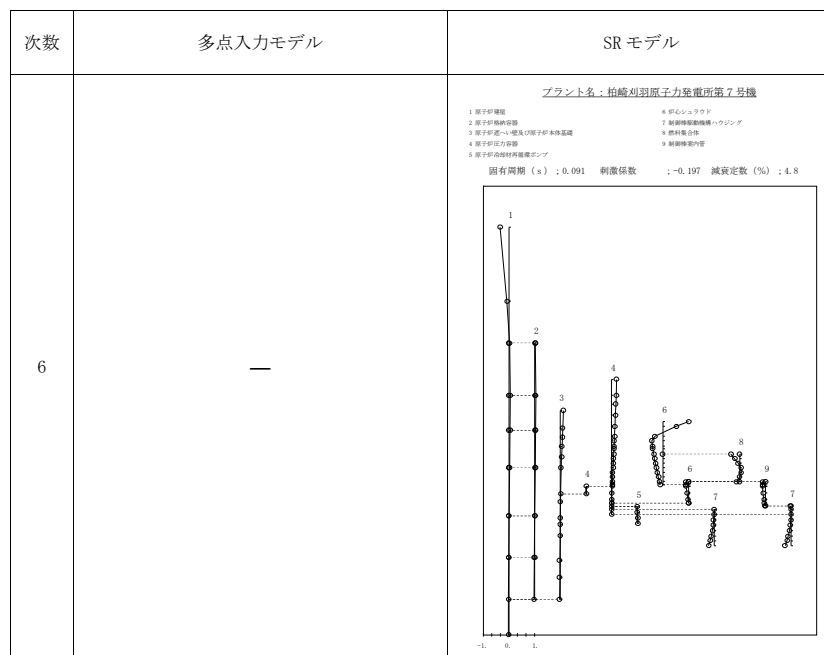
図添 9-1 振動モードの比較 (Sd-1, NS 方向) (6/11)
