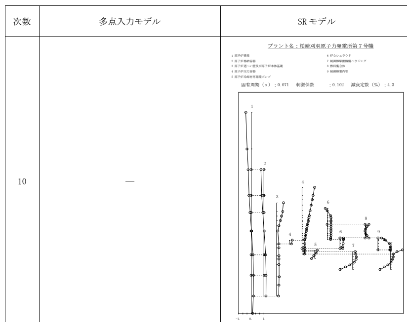
図添 9-2 振動モードの比較 (Sd-1, EW 方向) (10/11)
