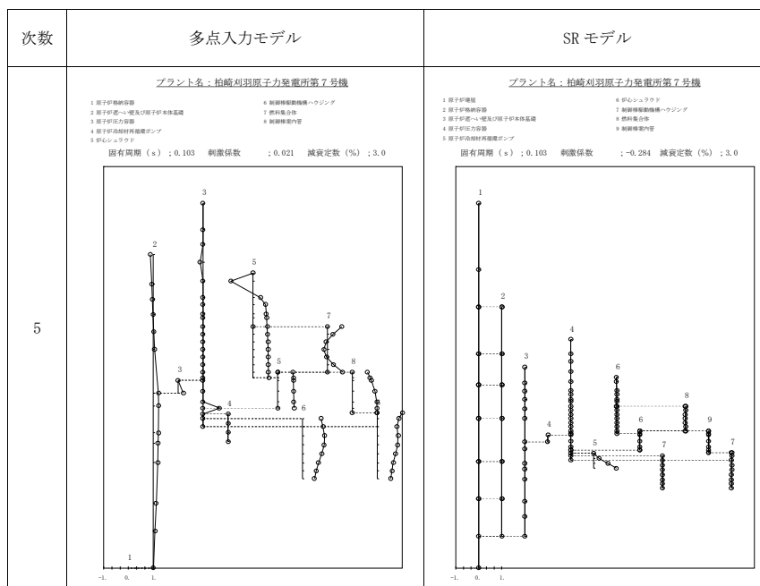
図添 9-2 振動モードの比較 (Sd-1, EW 方向) (5/11)
