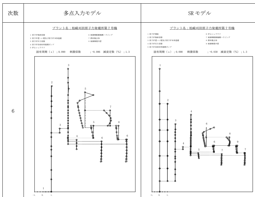
図添 9-2 振動モードの比較 (Sd-1, EW 方向) (6/11)
