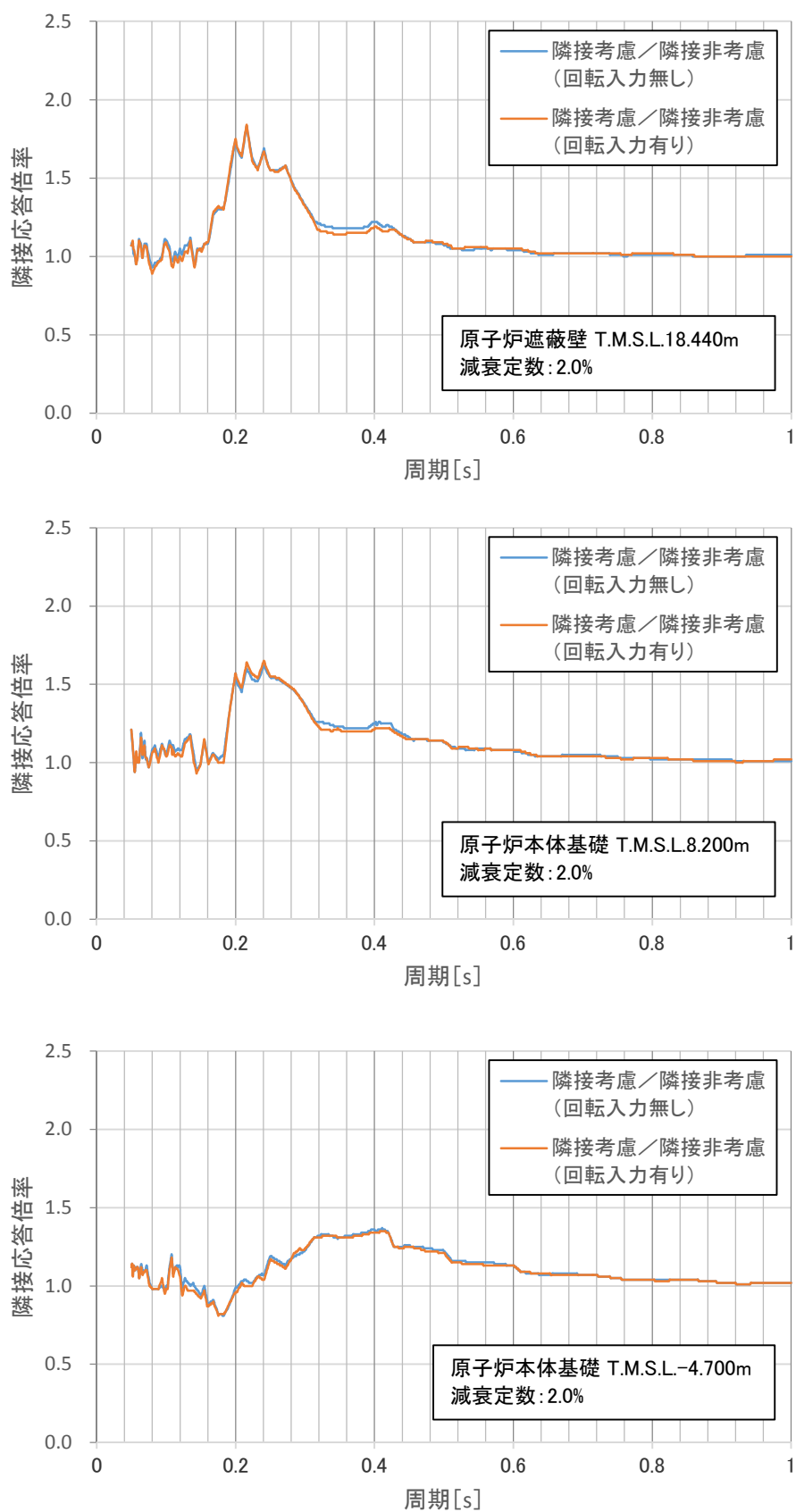
図添 6-1 回転入力の影響 (隣接応答倍率, 床応答スペクトル)
