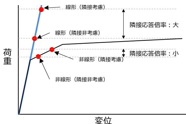
図添 8-1 荷重と変位の関係
