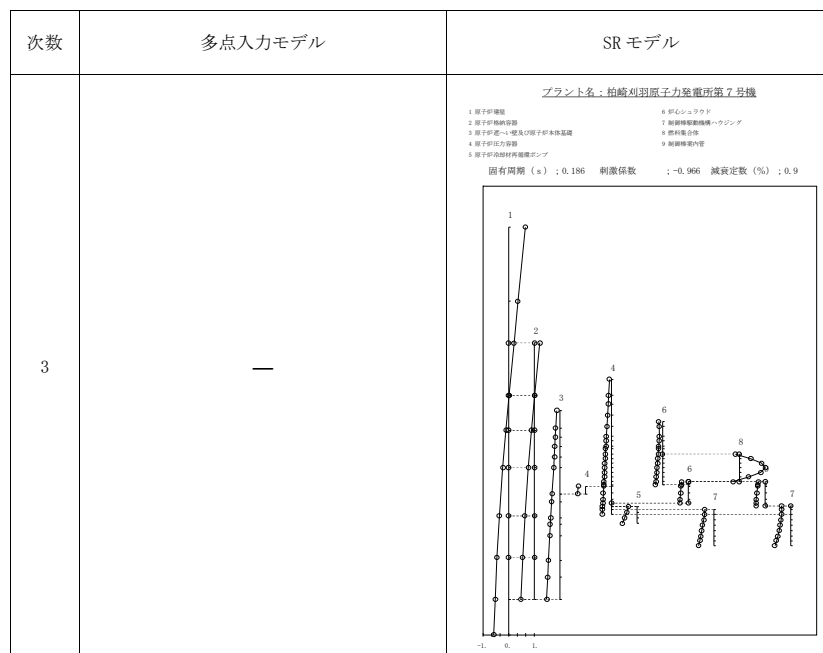
図添 9-2 振動モードの比較 (Sd-1, EW 方向) (3/11)
