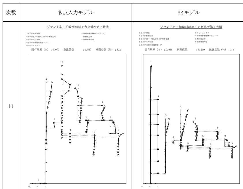
図添 9-1 振動モードの比較 (Sd-1, NS 方向) (11/11)
