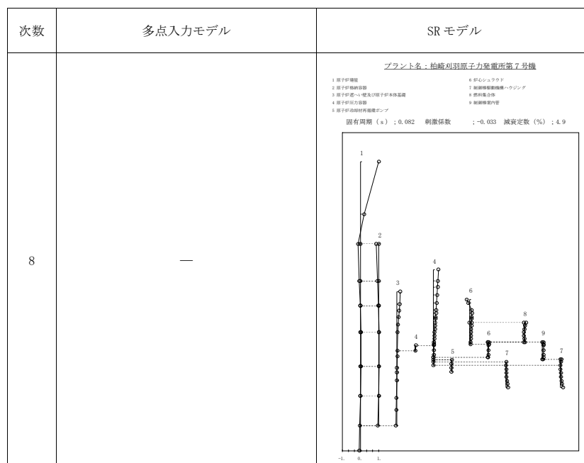
図添 9-2 振動モードの比較 (Sd-1, EW 方向) (8/11)
