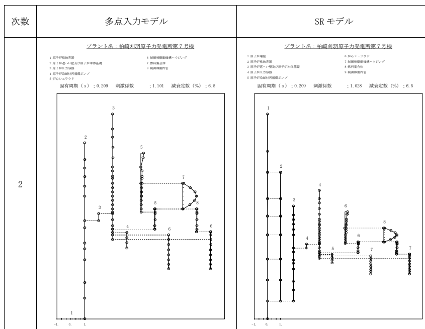
図添 9-1 振動モードの比較 (Sd-1, NS 方向) (2/11)
