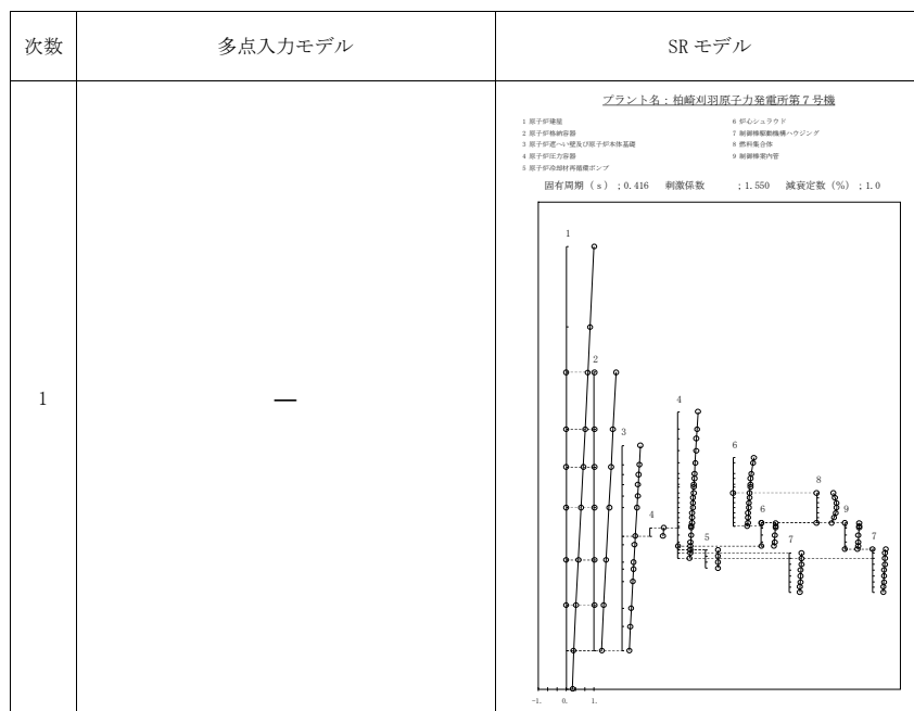
図添 9-2 振動モードの比較 (Sd-1, EW 方向) (1/11)
