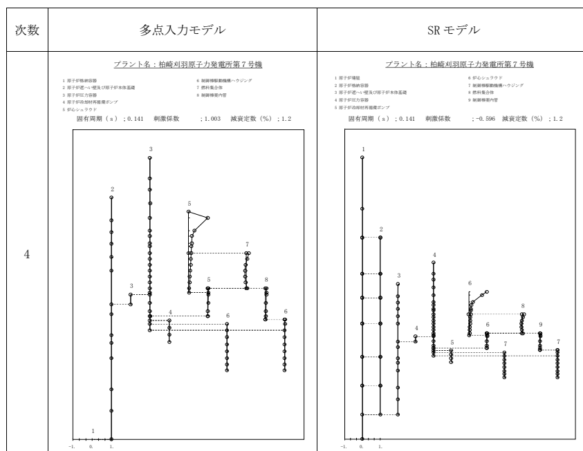
図添 9-2 振動モードの比較 (Sd-1, EW 方向) (4/11)
