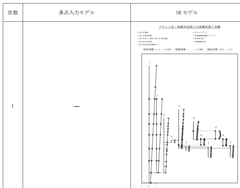
図添 9-1 振動モードの比較 (Sd-1, NS 方向) (1/11)
