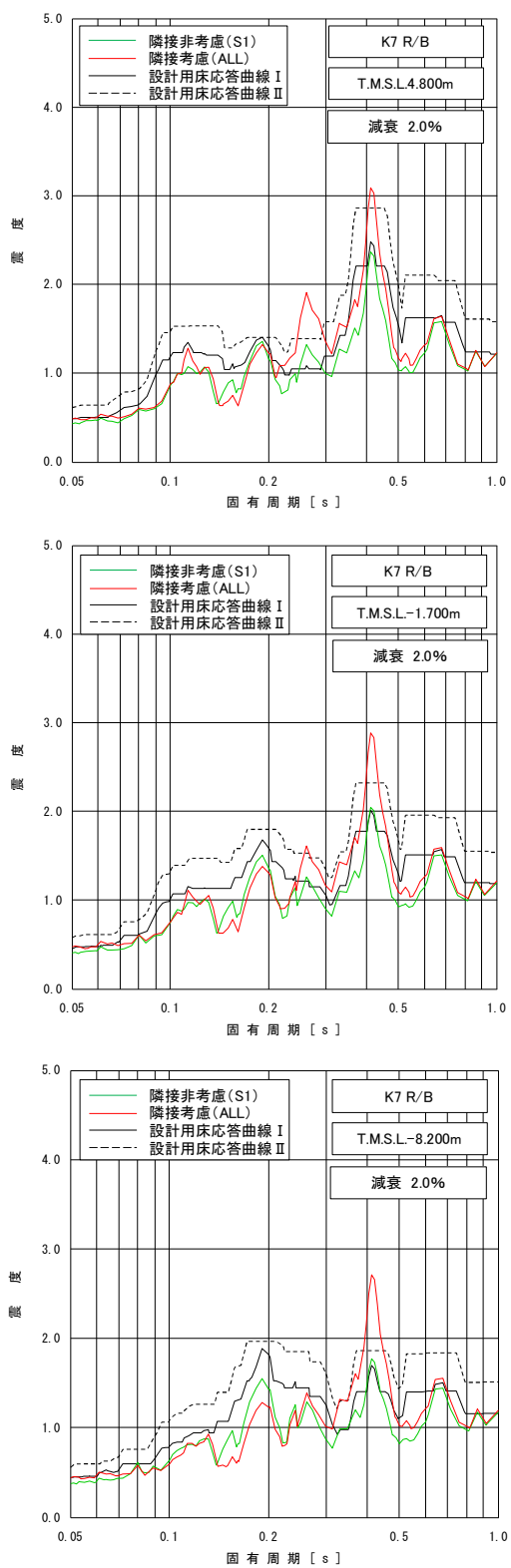
図添 1-1 床応答スペクトルの比較 (7号機原子炉建屋, 水平方向, 減衰 2.0%) (3/3)
