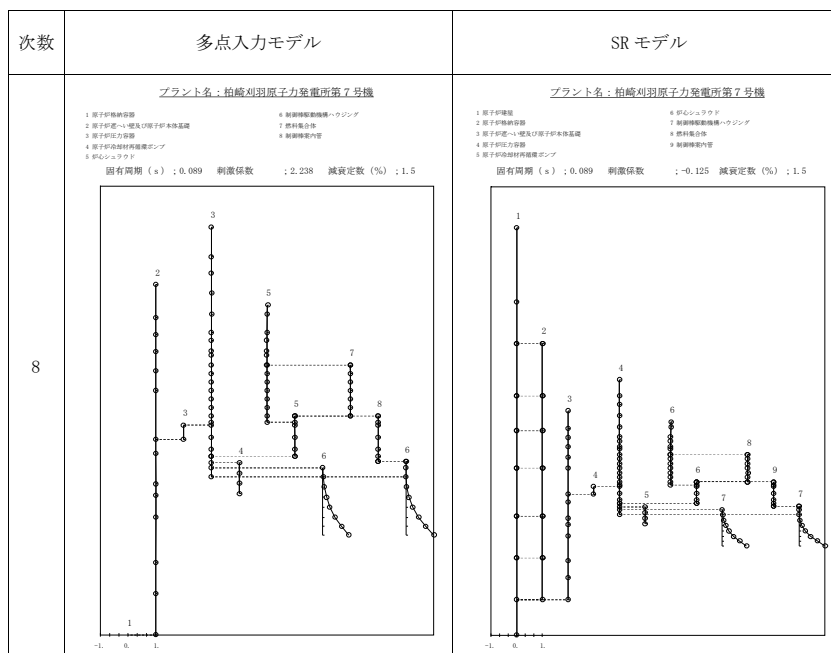
図添 9-1 振動モードの比較 (Sd-1, NS 方向) (8/11)
