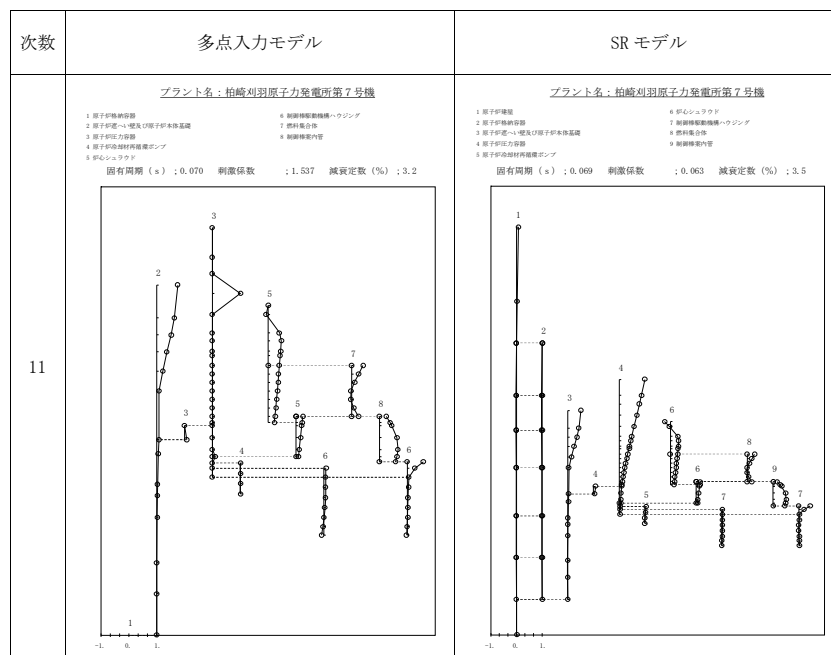
図添 9-2 振動モードの比較 (Sd-1, EW 方向) (11/11)
