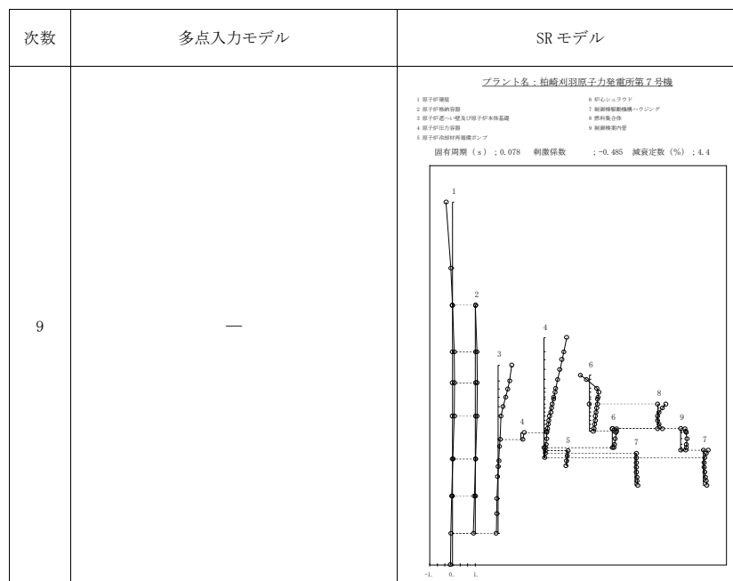
図添 9-2 振動モードの比較 (Sd-1, EW 方向) (9/11)
