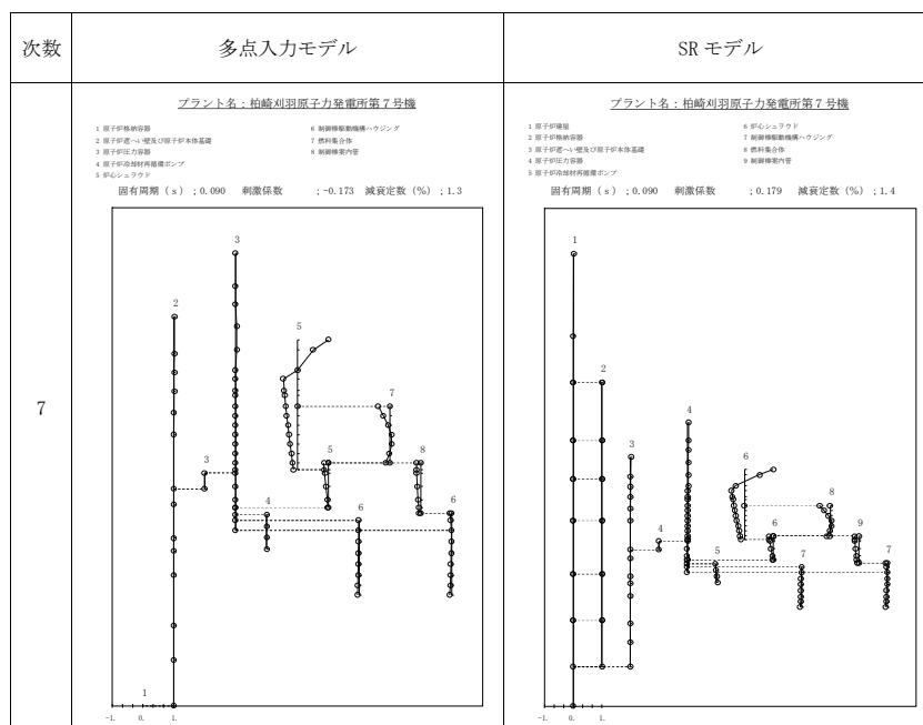
図添 9-1 振動モードの比較 (Sd-1, NS 方向) (7/11)
