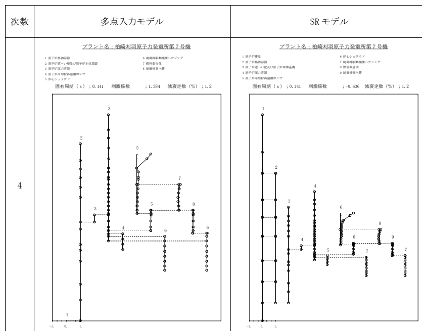
図添 9-1 振動モードの比較 (Sd-1, NS 方向) (4/11)
