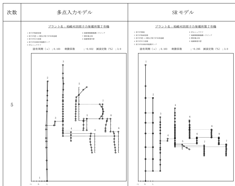
図添 9-1 振動モードの比較 (Sd-1, NS 方向) (5/11)
