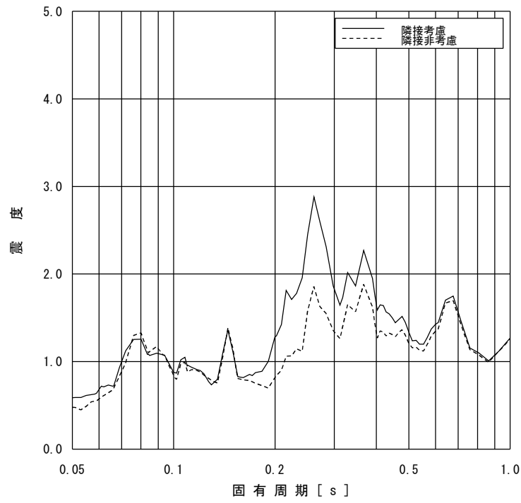
図 2-21 床応答スペクトルの比較 (炉心シュラウド T.M.S.L.14.433, 水平方向, 減衰 2.0%)
