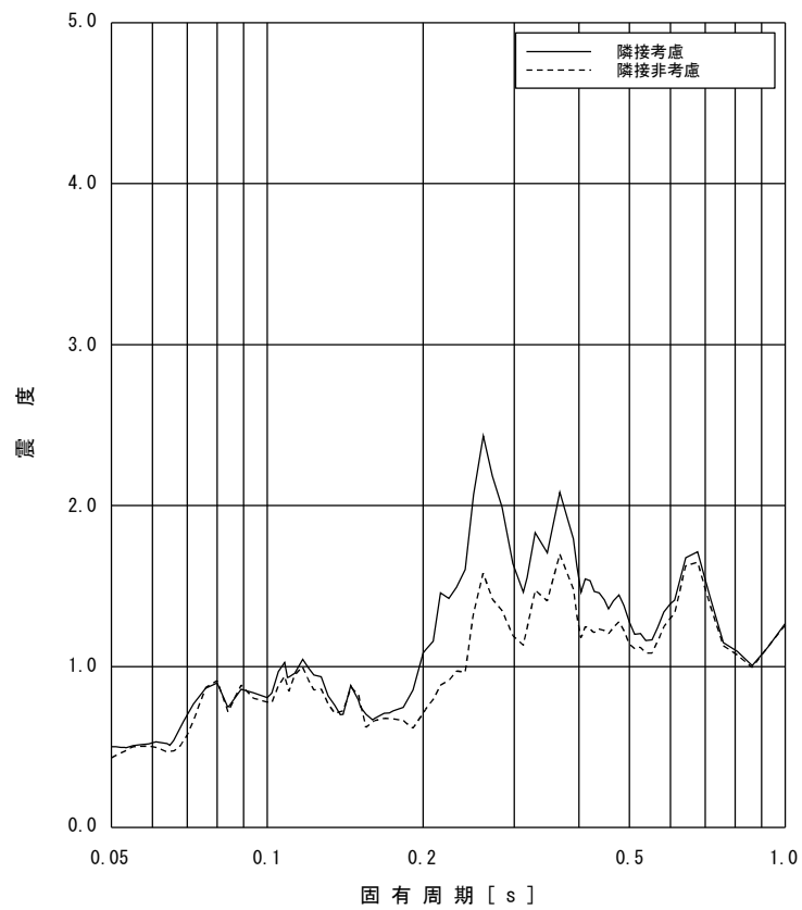
図 2-22 床応答スペクトルの比較 (炉心シュラウド T.M.S.L.10.161, 水平方向, 減衰 2.0%)
