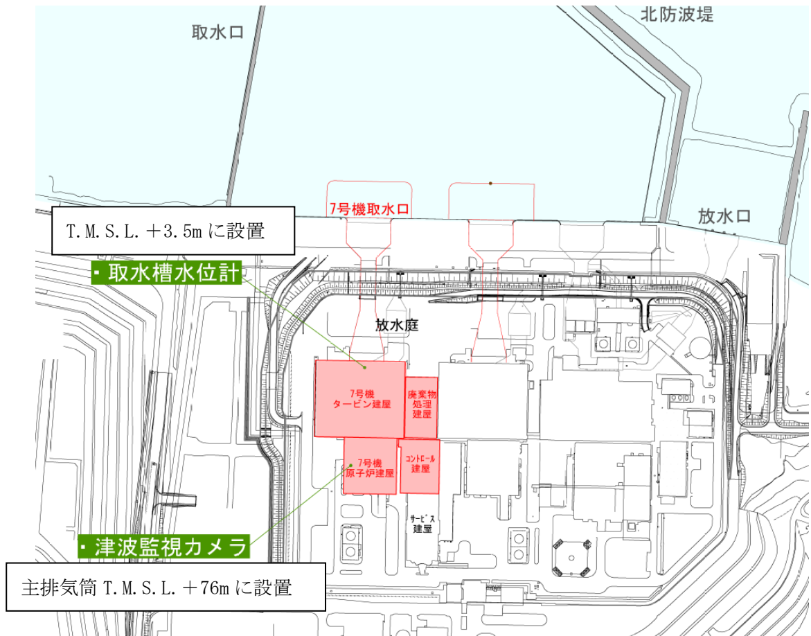
図 5.2-4 津波監視設備の配置図
