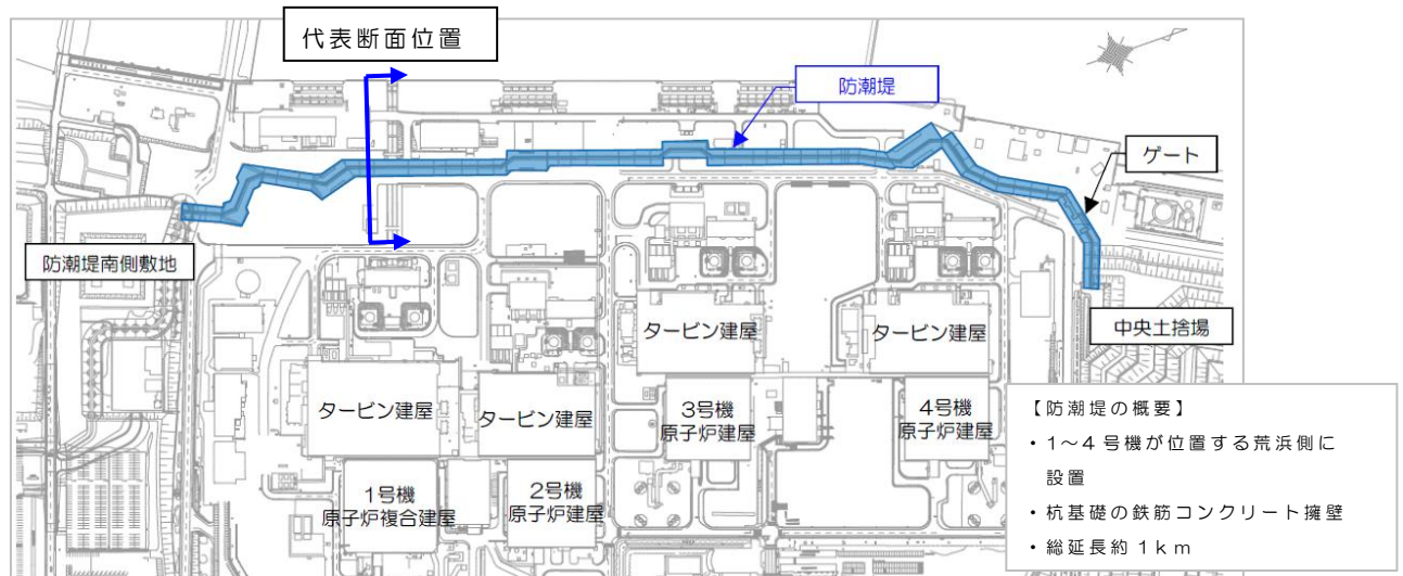
図 1.2-26(1) 荒浜側防潮堤の概要
