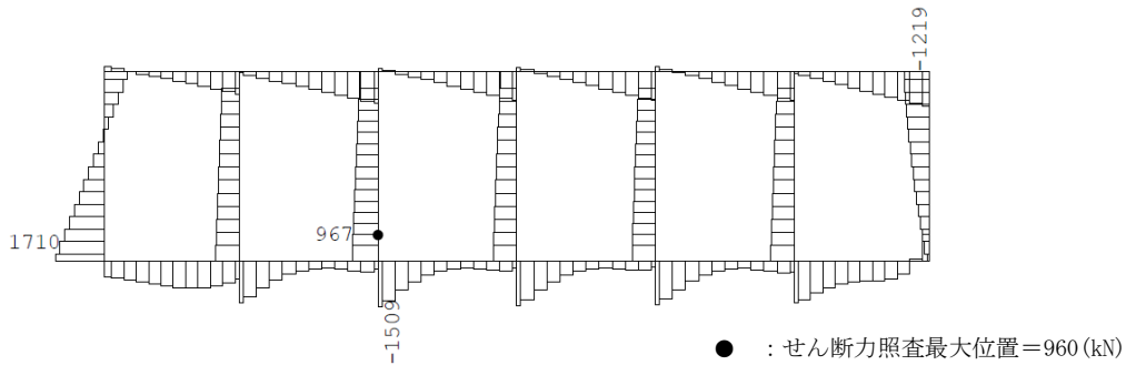
せん断力(kN)
