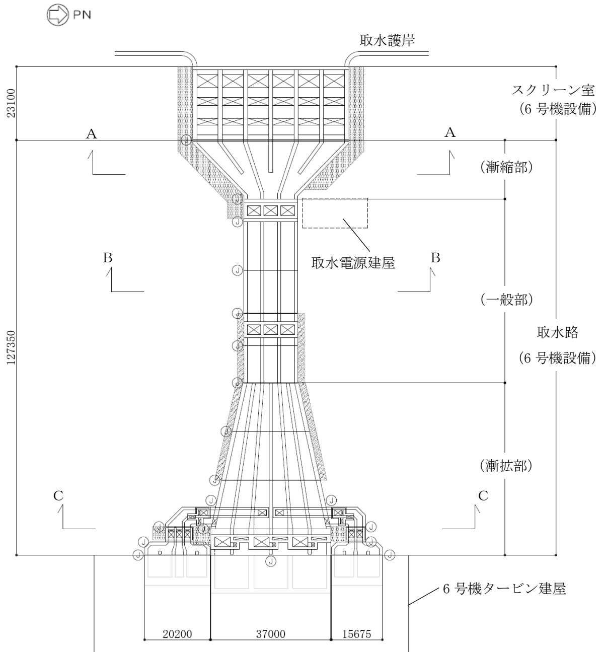
図2-2 取水路（6号機設備）の平面図
