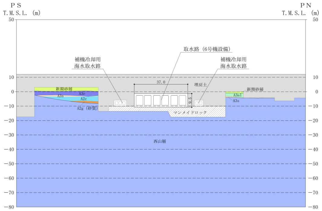
図 3-2 (3) 取水路 (6号機設備) の評価対象断面図 (C-C断面)
