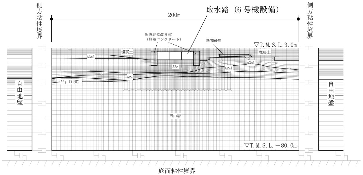
図 3-7 (1) 取水路 (6号機設備) の地震応答解析モデル (A-A断面)
