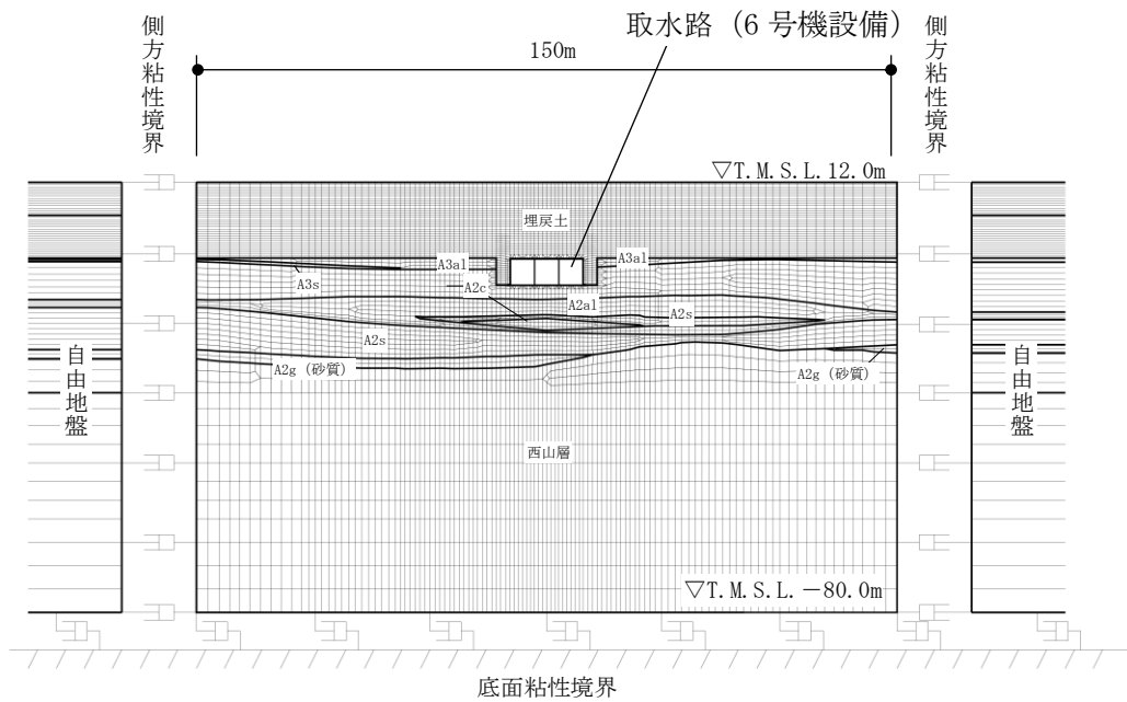
図 3-7 (2) 取水路 (6号機設備) の地震応答解析モデル (B-B断面)
