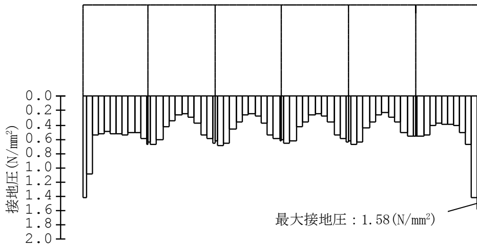
図3-10 C-C断面の最大接地圧分布図 (解析ケース②, Ss-1-+)
