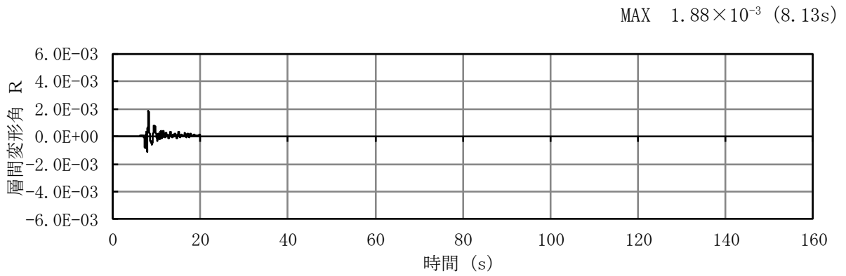
図 3-8 (2) B-B断面における層間変形角の時刻歴波形 (解析ケース⑤, S S -8++)
