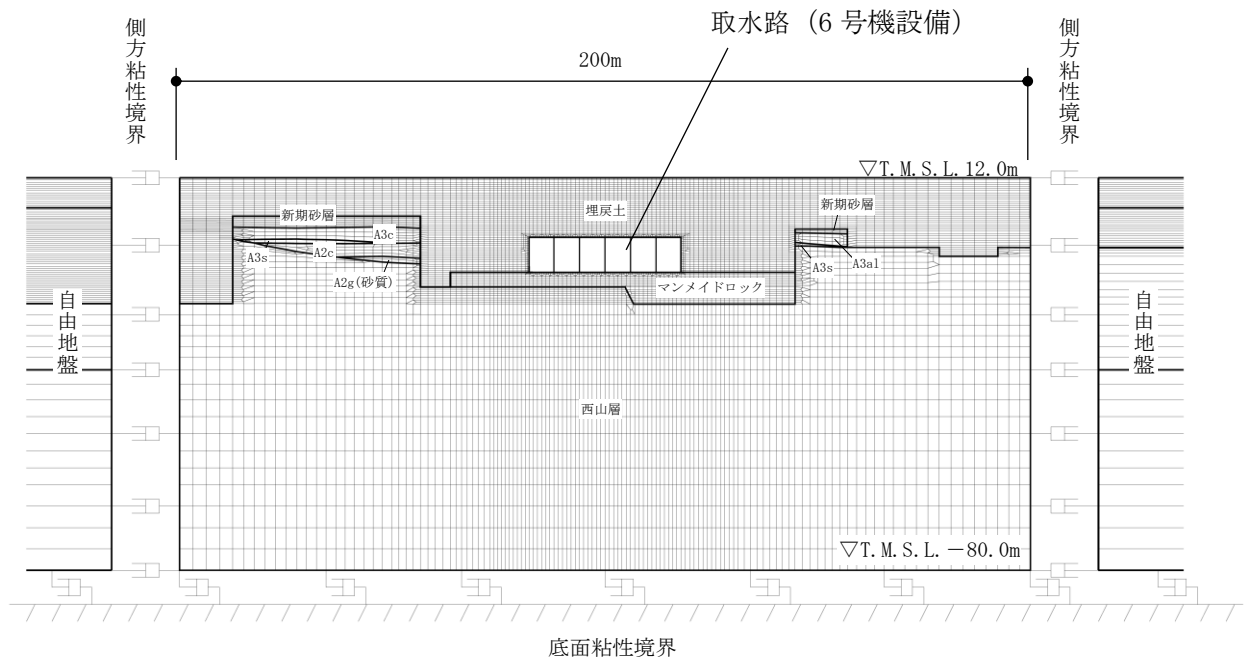
図 3-7 (3) 取水路 (6 号機設備) の地震応答解析モデル (C-C 断面)
