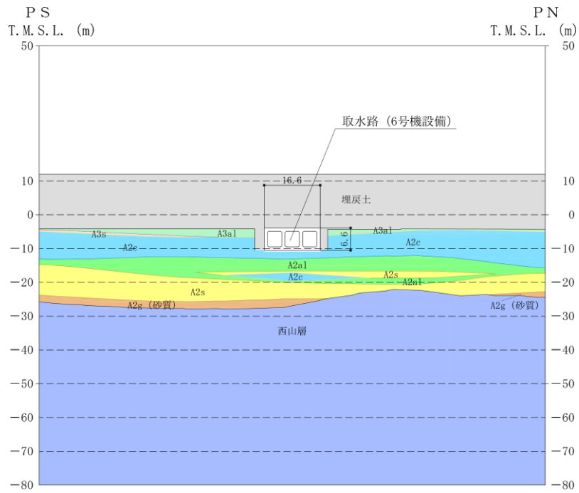
図 3-2 (2) 取水路 (6号機設備) の評価対象断面図 (B-B断面)
