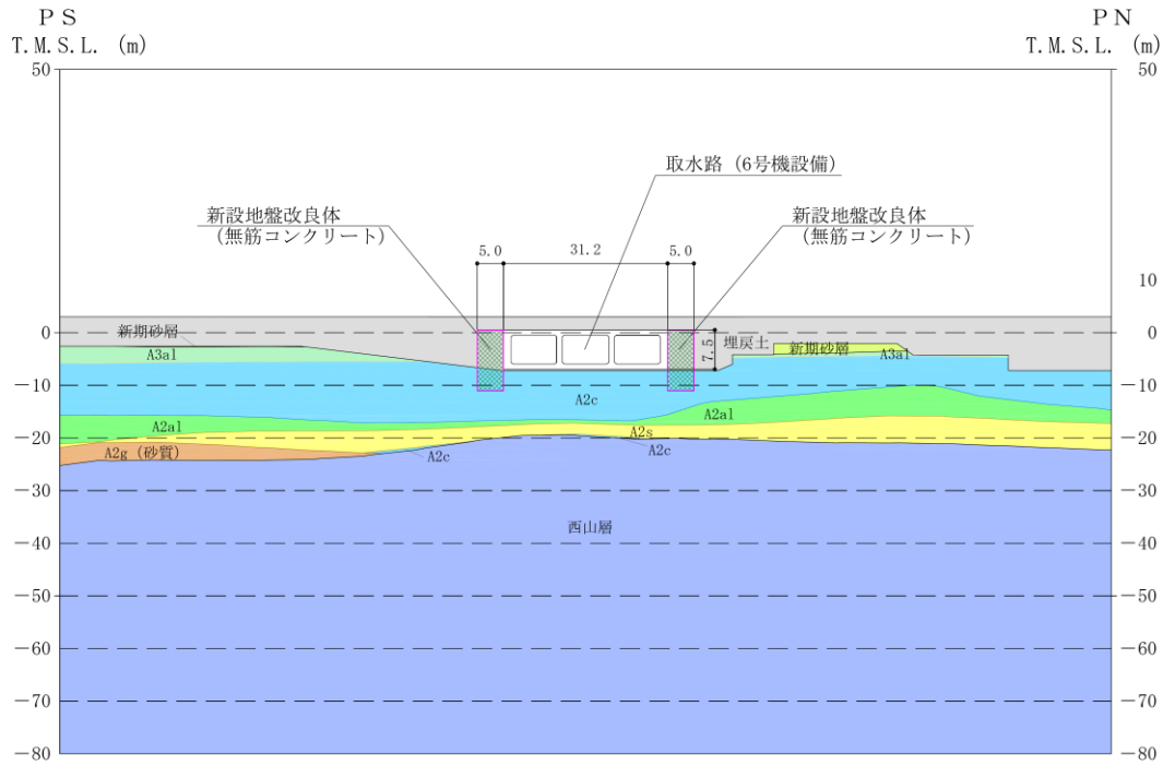
図 3-2 (1) 取水路 (6号機設備) の評価対象断面図 (A-A断面)
