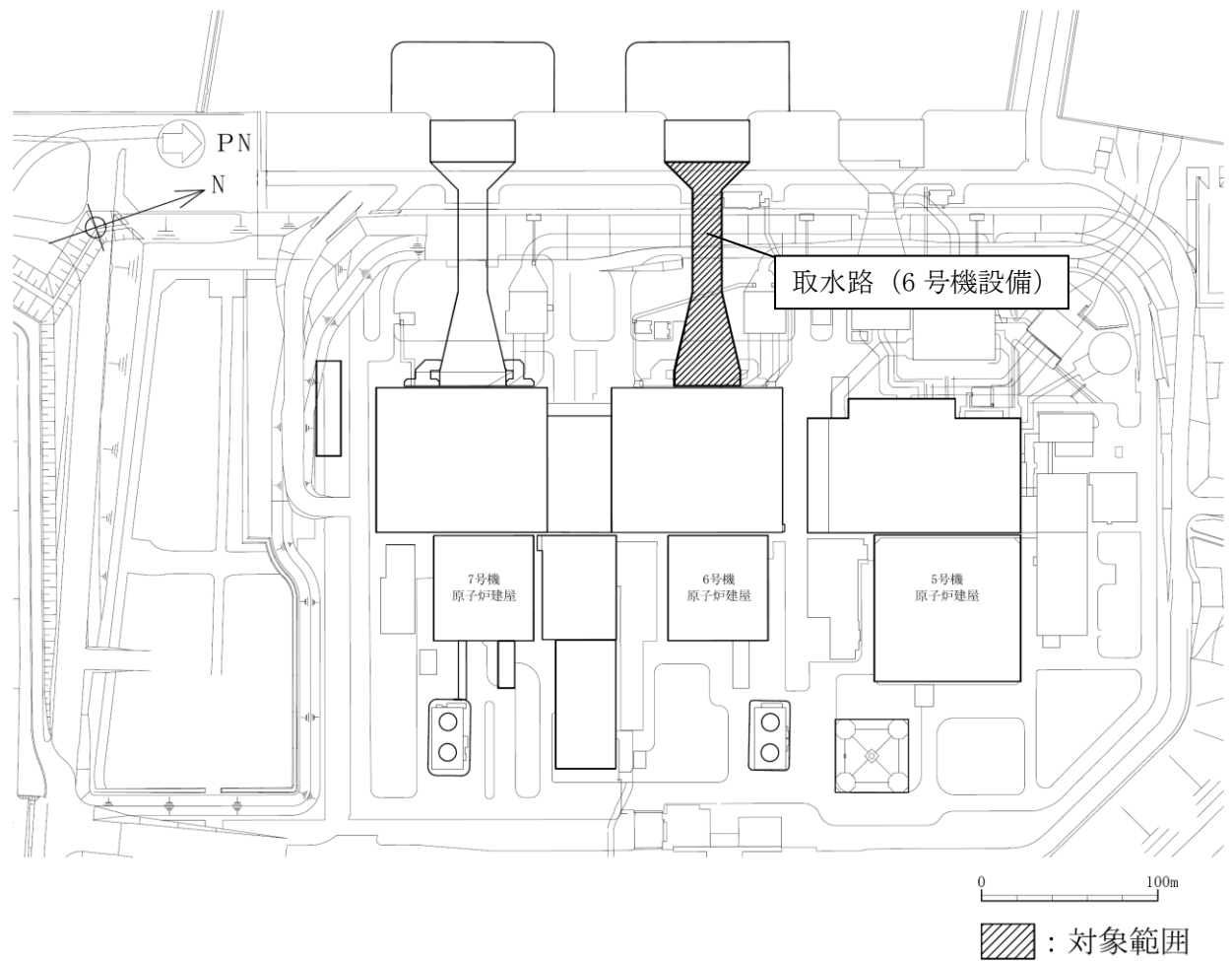
図2-1 取水路（6号機設備）の位置図（全体平面図）
