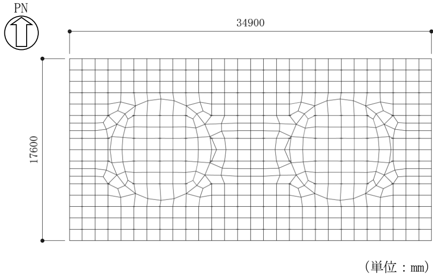
図 3-4 要素分割図
