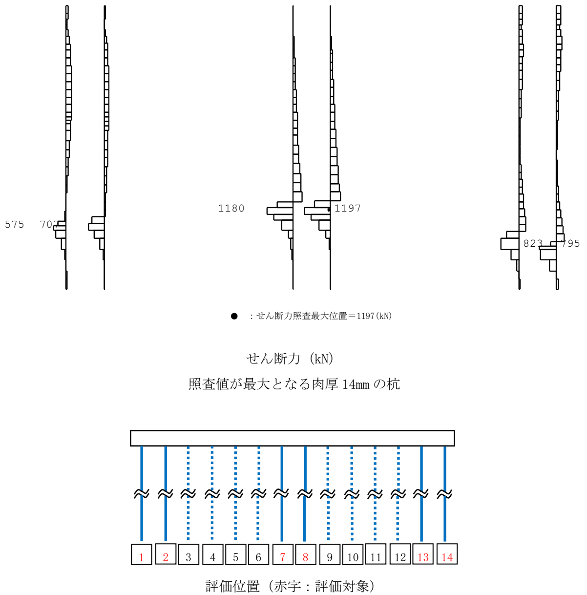
図 4-4 (2) 鋼管杭のせん断力照査値最大時の断面力 (B-B断面, 解析ケース③, Ss-7EW, t=58.33s)
