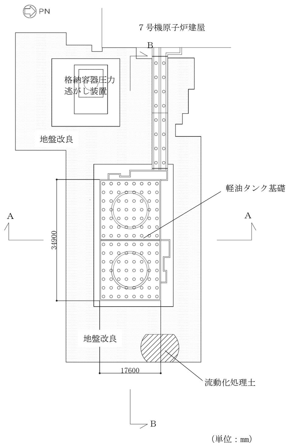
図 2-2 軽油タンク基礎の平面図
