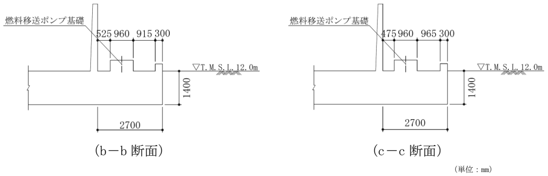
図 2-3 張出し基礎断面図
