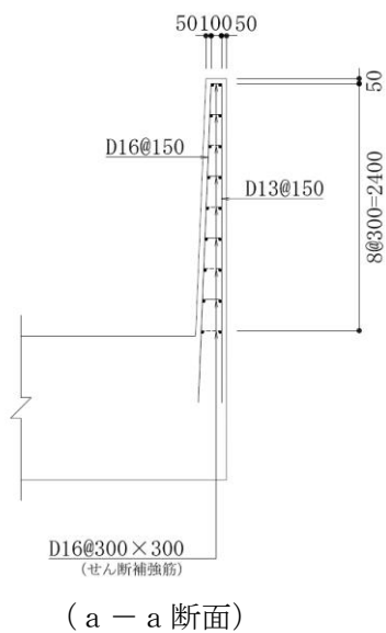
図 3-14 防油堤の評価対象断面
