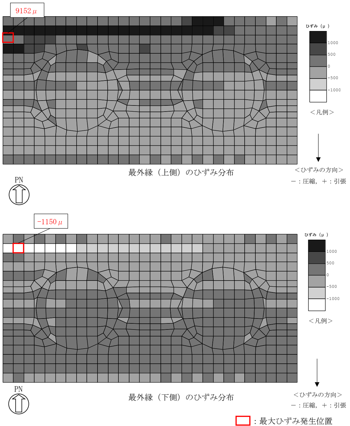
図 4-1 鉄筋コンクリート部材の曲げ軸力照査値最大時のひずみ分布図 (解析ケース①, Ss-1-+, t=5.83s)
