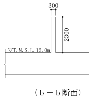
図 3-14 防油堤の評価対象断面
