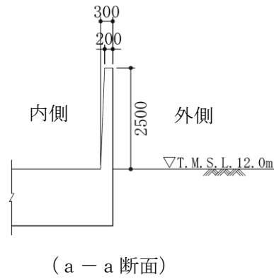
図 3-14 防油堤の評価対象断面
