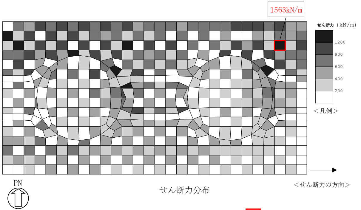
図 4-2 (2) 鉄筋コンクリート部材のせん断力照査値最大時の断面力分布図 (解析ケース③, Ss-8++, t=8.12s)
