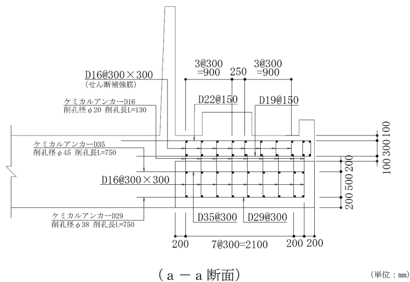
図 3-9 張出し基礎の概略配筋図*
