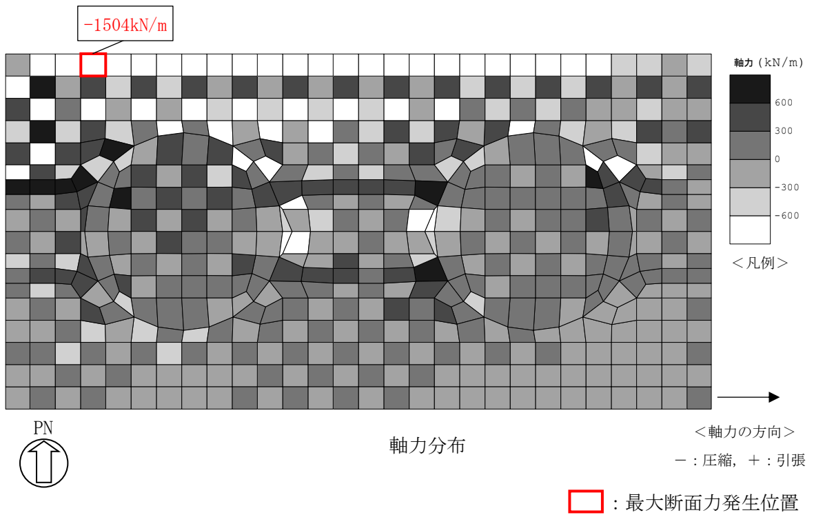
図 4-2 (1) 鉄筋コンクリート部材のせん断力照査値最大時の断面力分布図 (解析ケース③, Ss-8++, t=8.12s)
