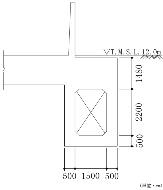
図 2-2 張出しダクト断面図 (a-a 断面)
