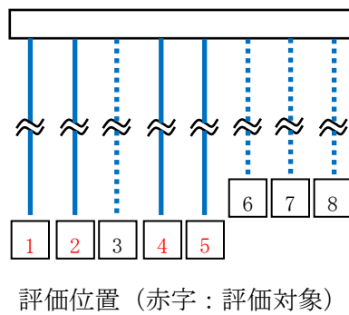
図 4-4 (1) 鋼管杭のせん断力照査値最大時の断面力分布図 (A-A断面, 解析ケース①, Ss-3-+, t=36.62s)
