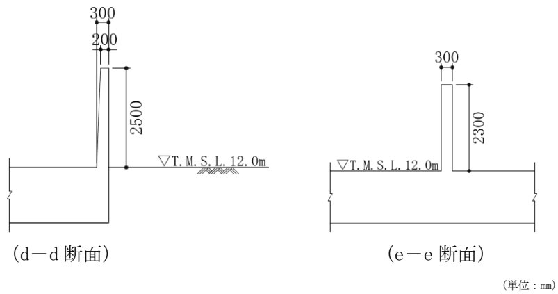
図 2-4 防油堤断面図
