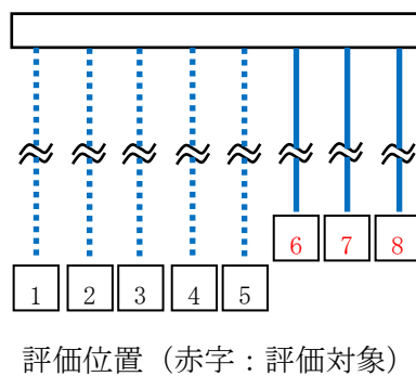
図 4-3 (1) 鋼管杭の曲げ軸力照査値最大時の曲率分布図 (A-A断面, 解析ケース①, Ss-3+-, t=36.64s)
