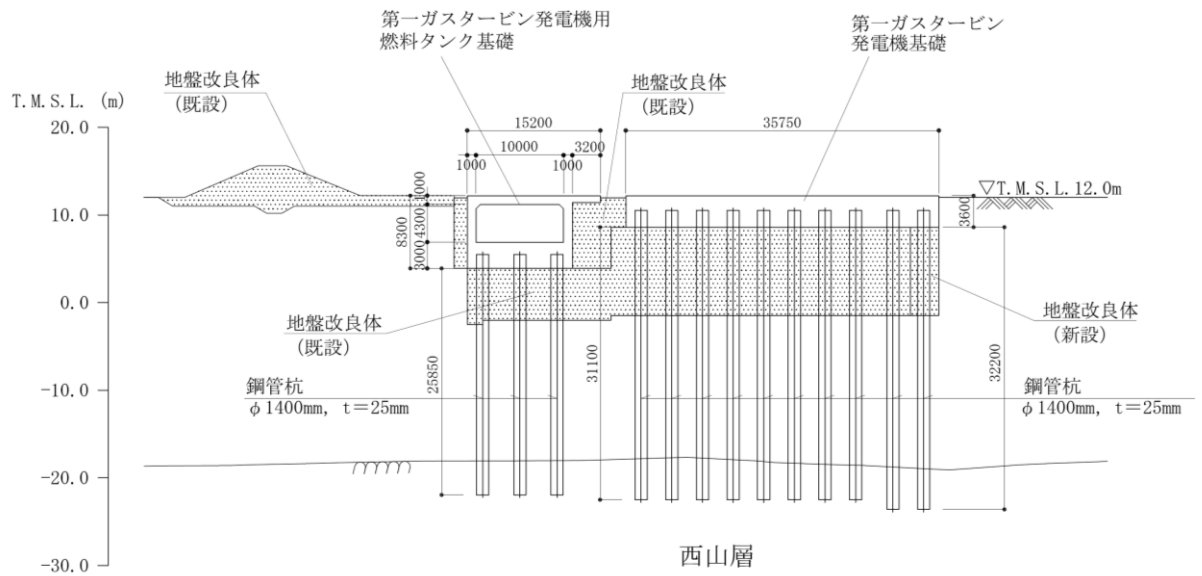
図 2-3 (3) 常設代替交流電源設備基礎の断面図 (C-C 断面)
