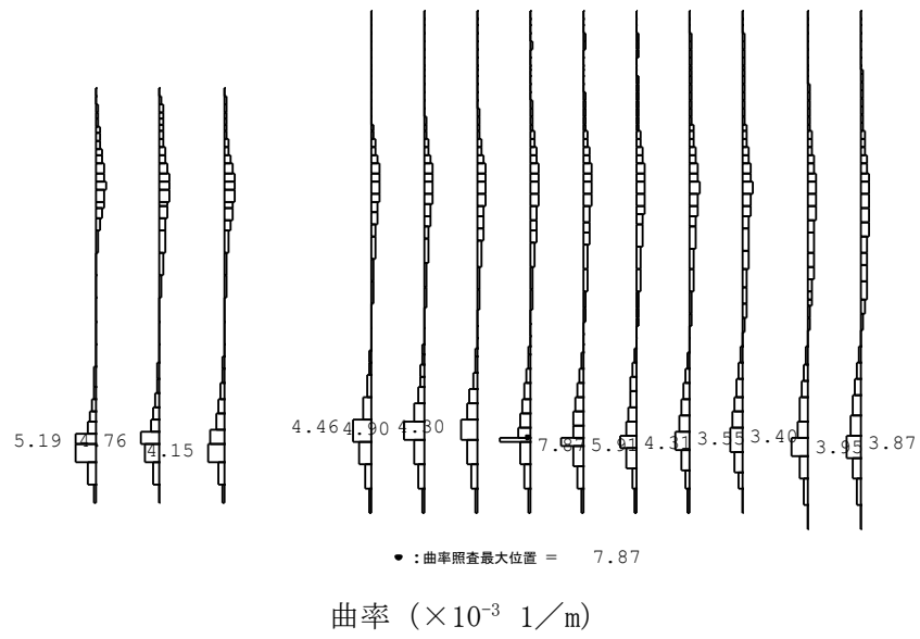
図 4-5 (3) 鋼管杭の曲げ軸力照査値最大時の曲率分布図 (C-C断面, 解析ケース③, Ss-3--, t=37.56s)
