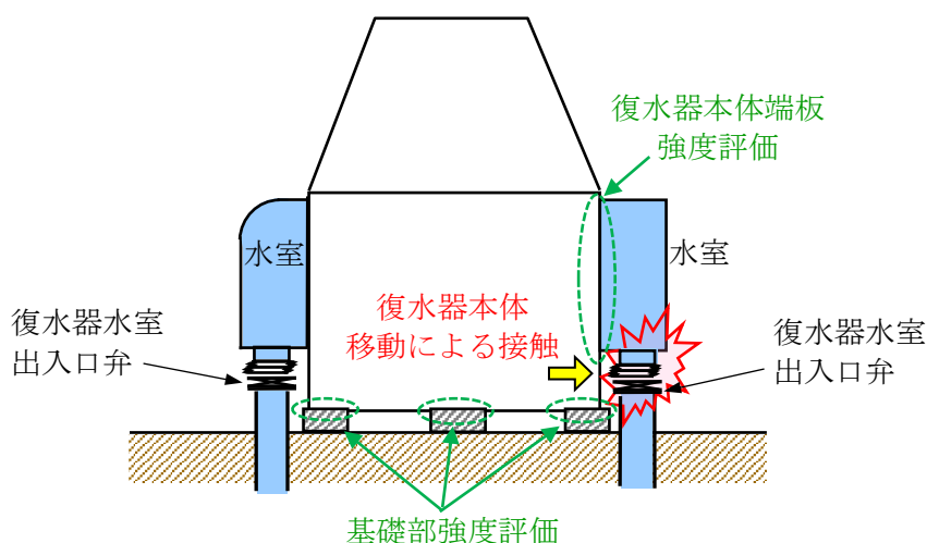
第9.17-2図 地震時の復水器水室出入口弁へ (B. 復水器本体移動による接触影
