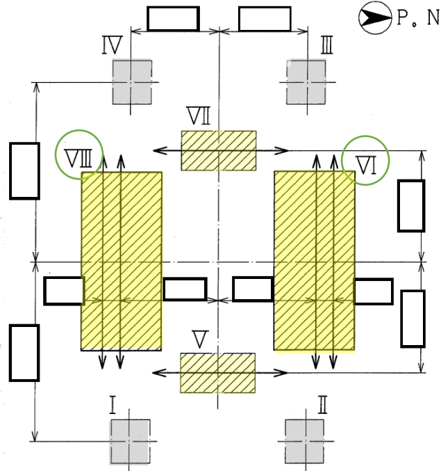
第 9.17-29 図 細管軸方向を拘束する復水器ずれ止め基礎台
