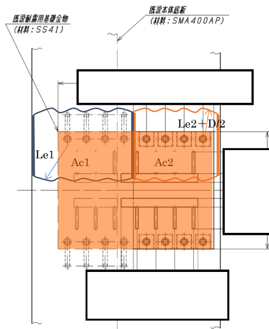
第 9.17-30 図 溝形金物形状と基礎ボルト配置寸法
