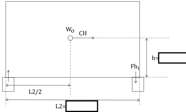
第 9.17-27 図 復水器の細管軸方向への転倒
