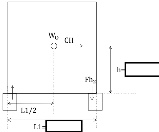
第 9.17-28 図 復水器の細管軸直角方向への転倒
