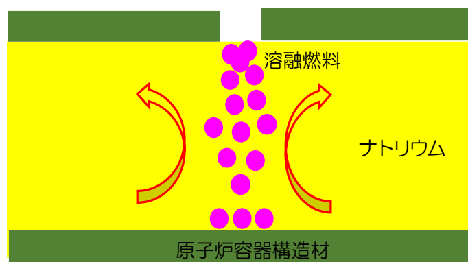
図4 溶融燃料のナトリウムプレナム内流入時モデル概念図
