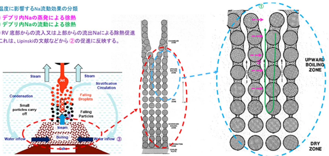
図1 デブリベッド内冷却のメカニズム
