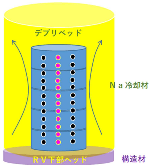
図2 1次元デブリベッド冷却モデルと3次元ナトリウム流動の連成解析モデル
