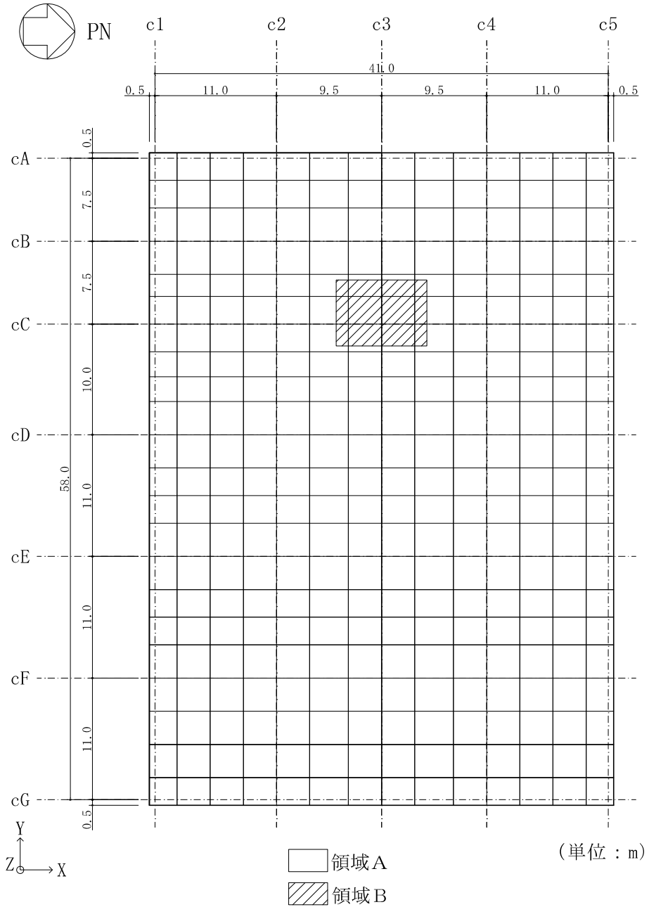
図 6-4 基礎スラブの配筋領域図 (EW 方向, 下ば筋)
