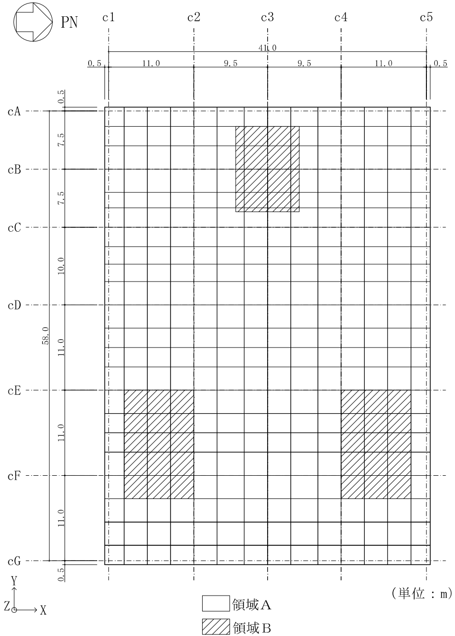
図 6-1 基礎スラブの配筋領域図 (NS 方向, 上ば筋)
