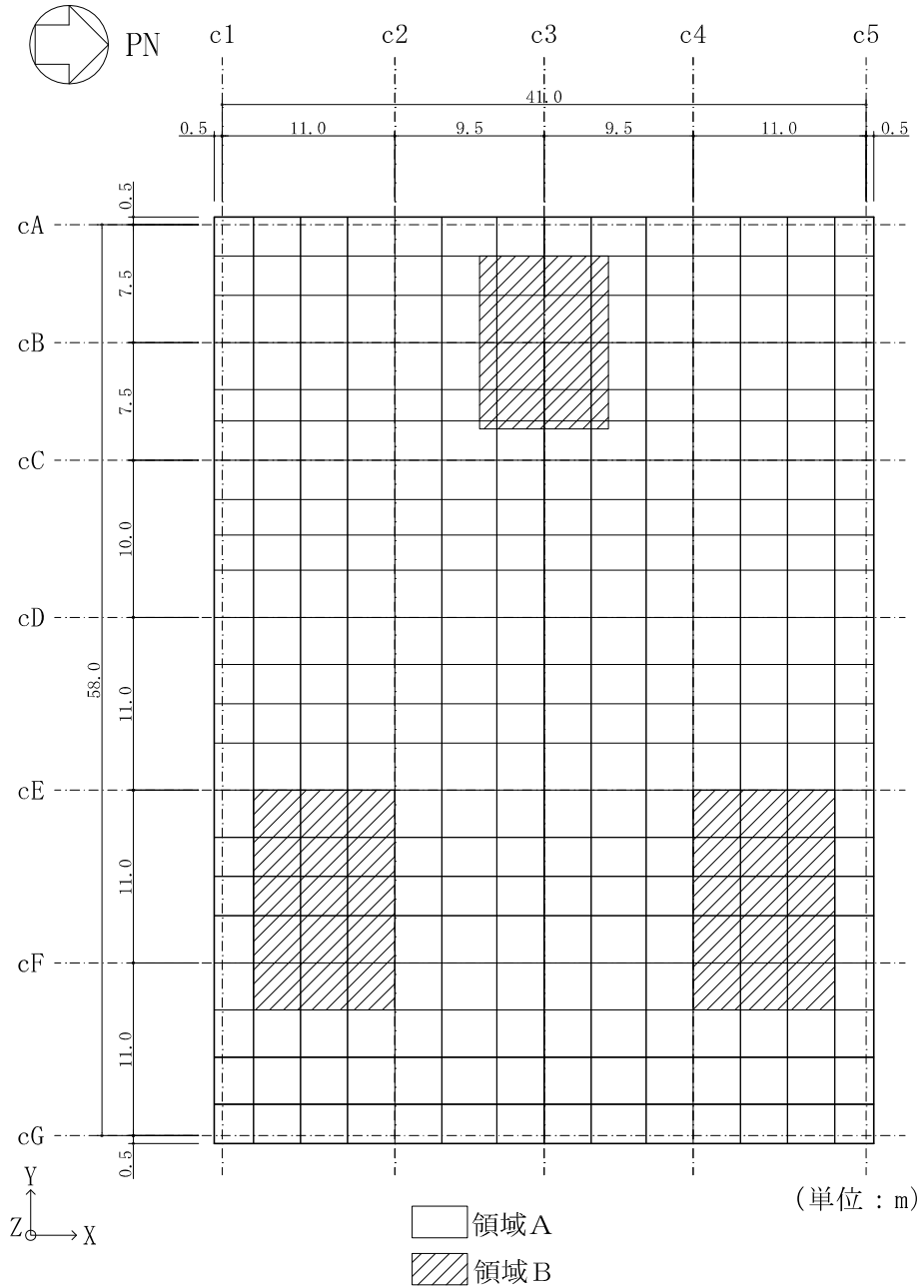
図 6-3 基礎スラブの配筋領域図 (EW 方向, 上ば筋)
