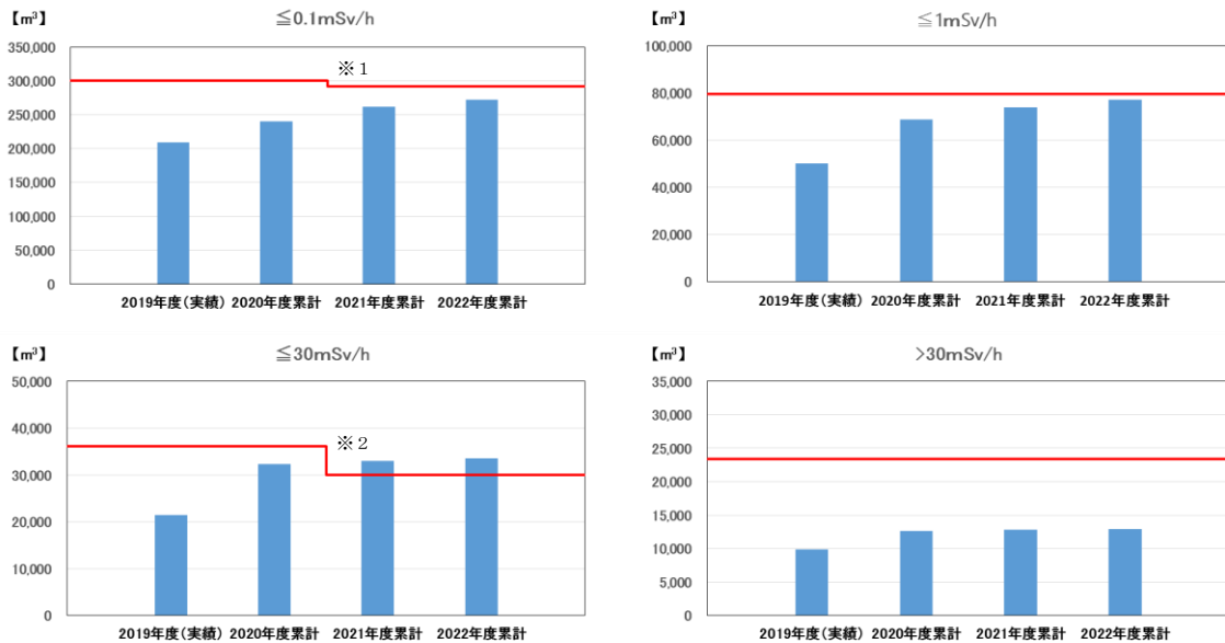
図 2. 1. 1 - 2 - 1 瓦礫等の想定保管量
