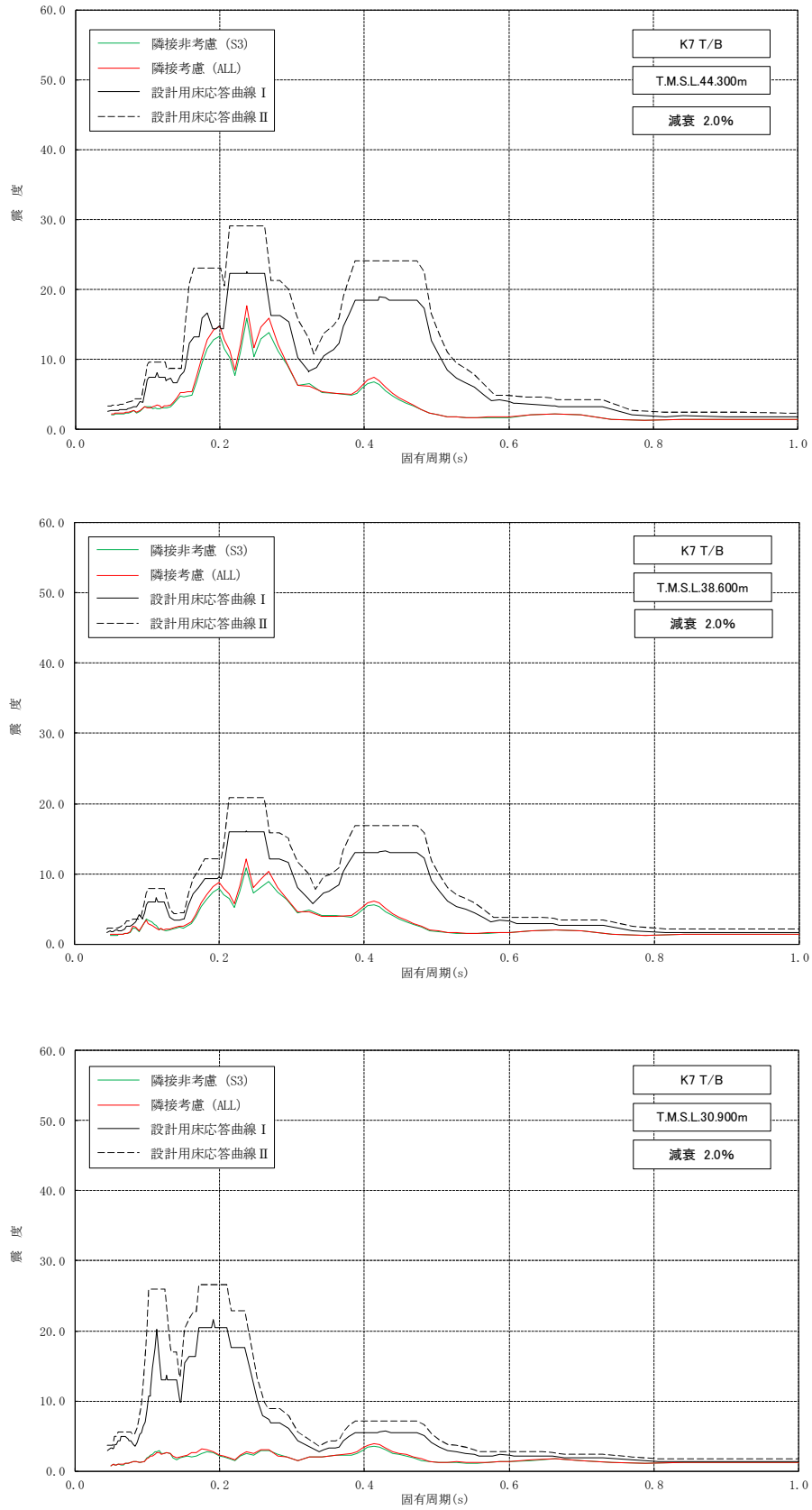
図 2-25 床応答スペクトルの比較 (7号機タービン建屋, 水平方向, 減衰 2.0%) (1/3)
