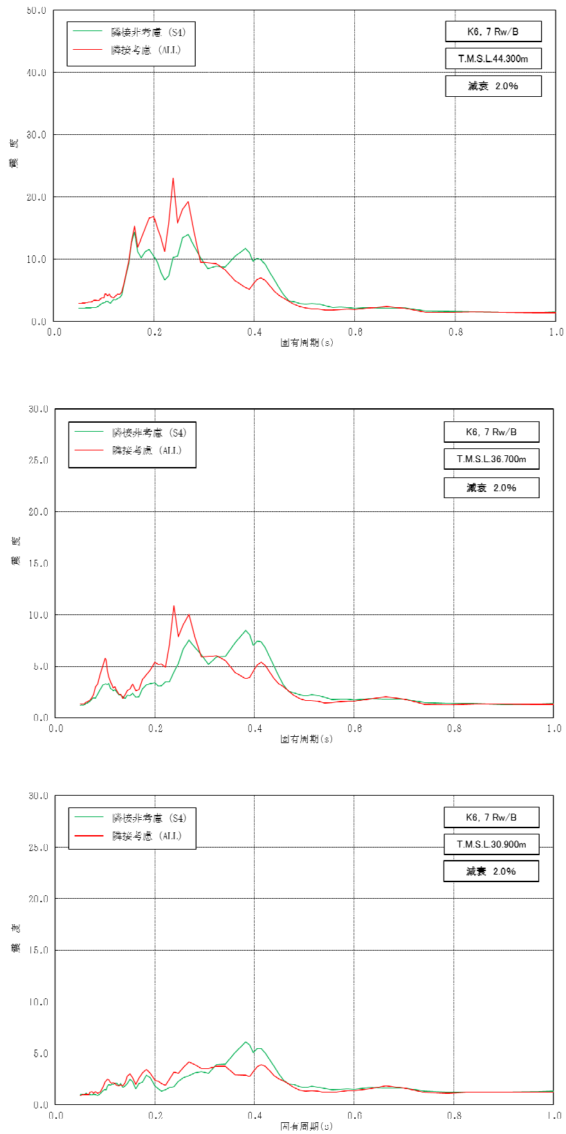
図 2-26 床応答スペクトルの比較（廃棄物処理建屋，水平方向，減衰 2.0%）（1/3）
