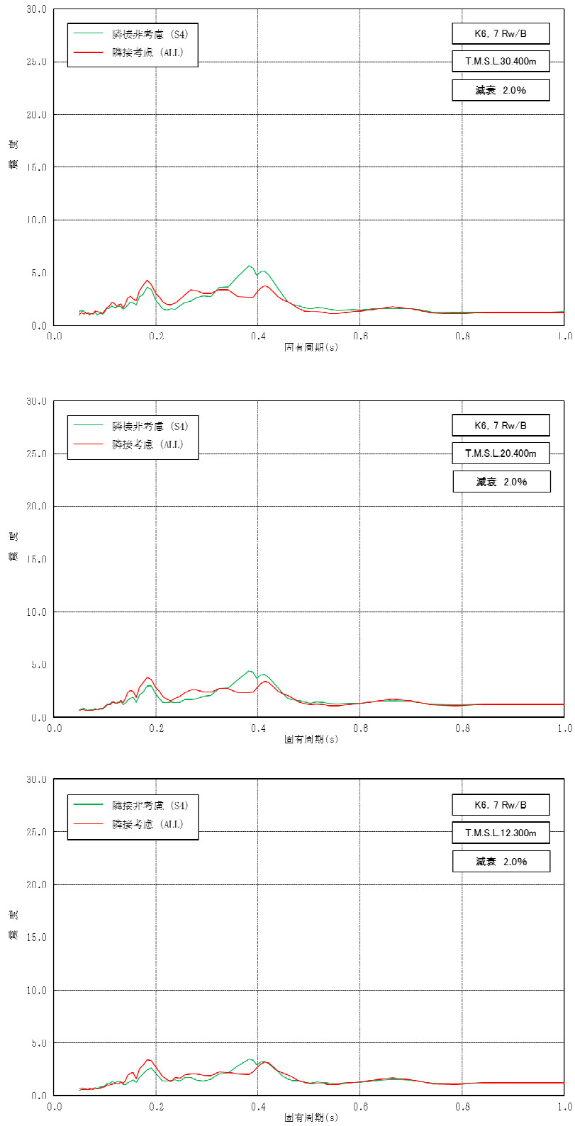
図 2-26 床応答スペクトルの比較（廃棄物処理建屋，水平方向，減衰 2.0%）(2/3)
