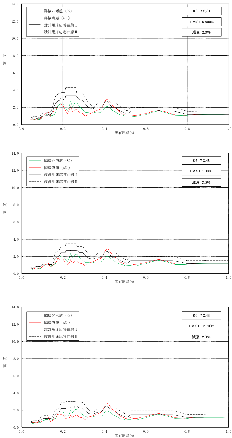
図 2-24 床応答スペクトルの比較 (コントロール建屋, 水平方向, 減衰 2.0%) (2/2)
