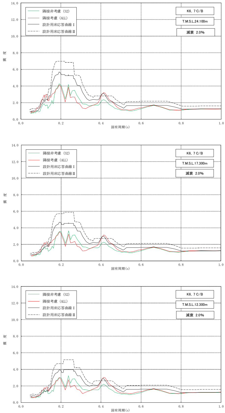
図 2-24 床応答スペクトルの比較 (コントロール建屋, 水平方向, 減衰 2.0%) (1/2)
