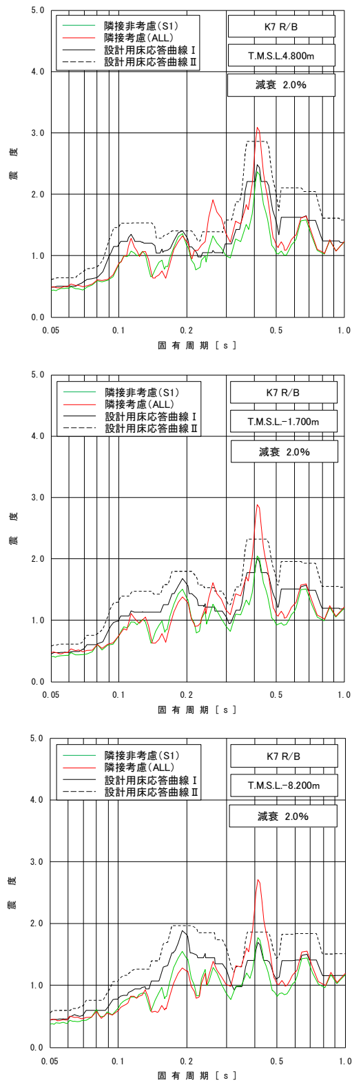
図 2-2 床応答スペクトルの比較 (7号機原子炉建屋, 水平方向, 減衰 2.0%) (3/3)
