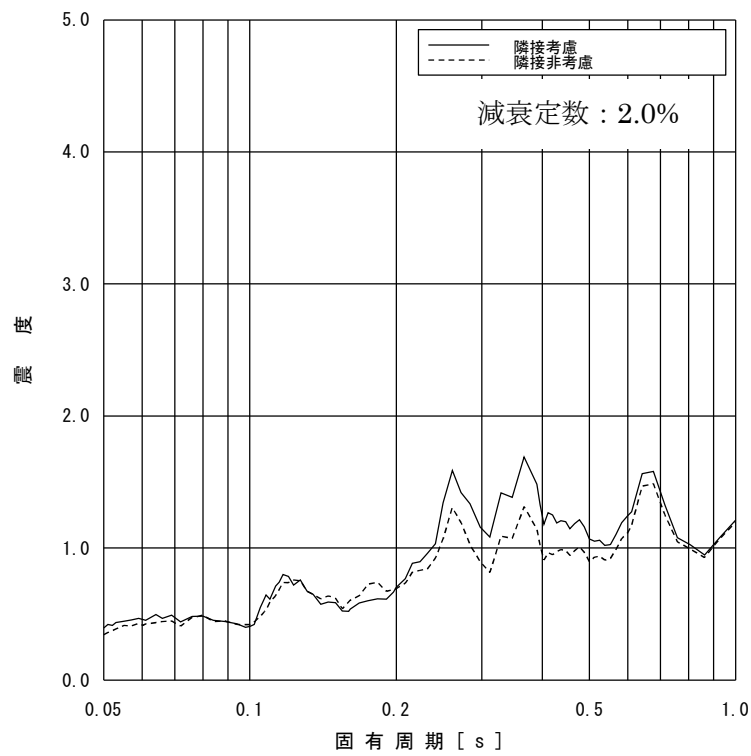
図 2-14 床応答スペクトルの比較 (原子炉本体基礎 T.M.S.L. -2.100, 水平方向, 減衰 2.0%)
