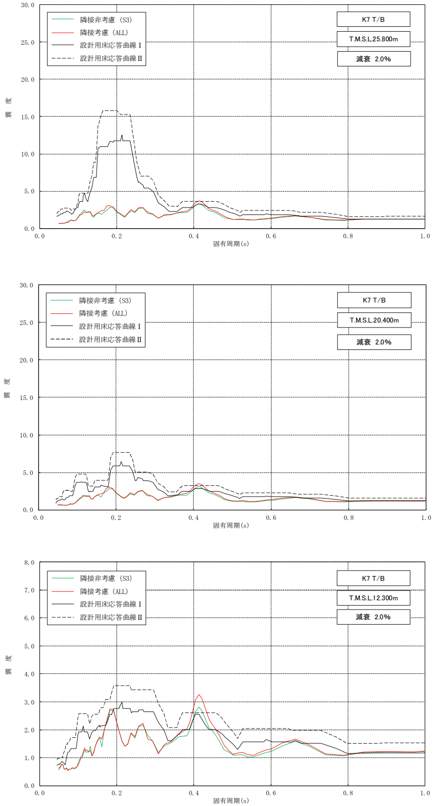
図 2-25 床応答スペクトルの比較 (7号機タービン建屋, 水平方向, 減衰 2.0%) (2/3)
