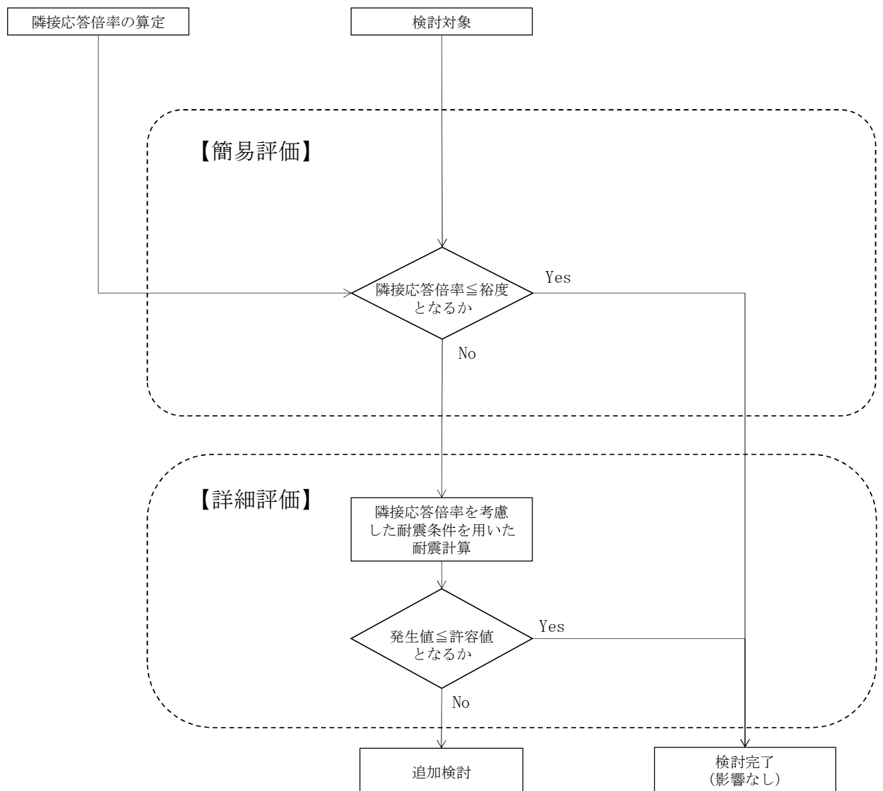
図1-1 影響検討フロー
