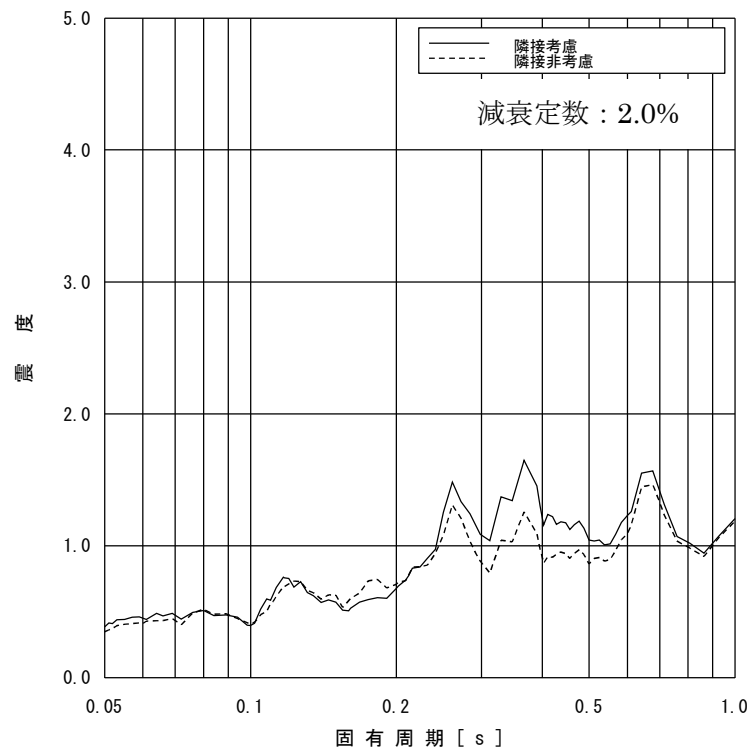
図 2-15 床応答スペクトルの比較 (原子炉本体基礎 T. M. S. L. -4.700, 水平方向, 減衰 2.0%)
