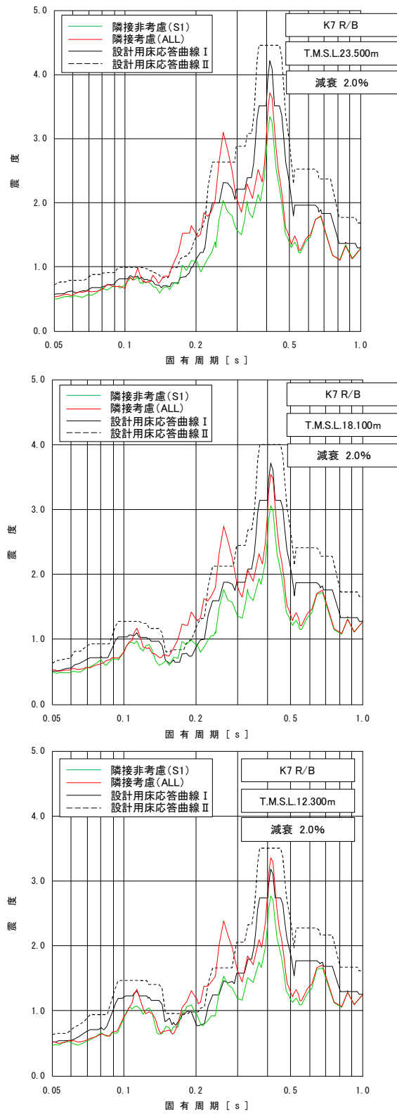
図 2-2 床応答スペクトルの比較 (7号機原子炉建屋, 水平方向, 減衰 2.0%) (2/3)
