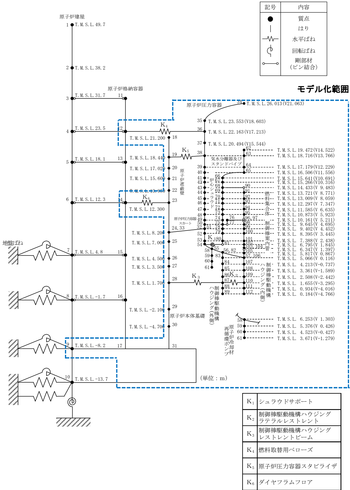
図 2-1 大型機器・炉内応答解析モデル
