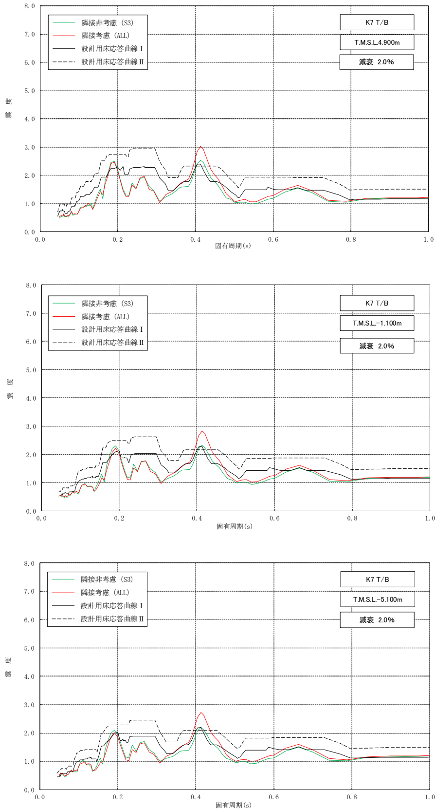
図 2-25 床応答スペクトルの比較 (7号機タービン建屋, 水平方向, 減衰 2.0%) (3/3)
