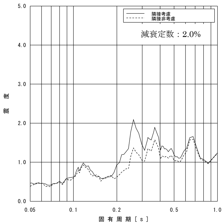
図 2-10 床応答スペクトルの比較 (原子炉本体基礎 T.M.S.L. 7.000, 水平方向, 減衰 2.0%)
