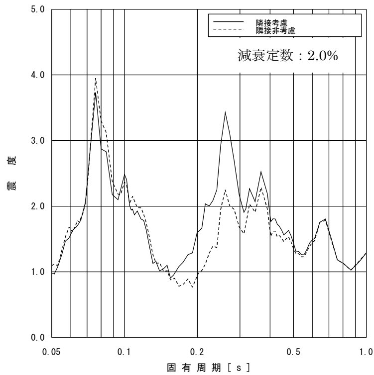
図 2-16 床応答スペクトルの比較 (原子炉压力容器 T. M. S. L. 26.013, 水平方向, 減衰 2.0%)
