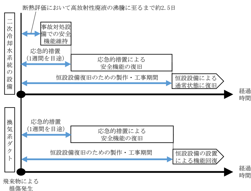
図-1 屋上の二次冷却系統の設備等の段階的な復旧の考え方
