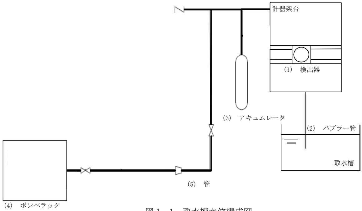
図 1-1 取水槽水位構成図
