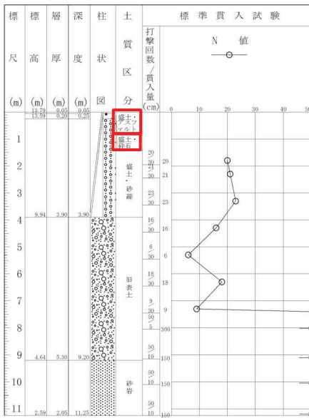
図 1.1-34 ボーリング柱状図・コア写真 (28QB-7)
