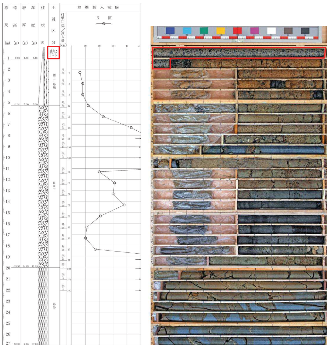
図 1.2-33 ボーリング柱状図・コア写真 (B-7)
