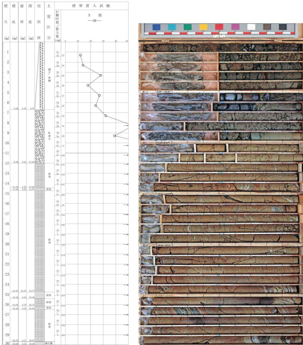
図 1.2-29 ボーリング柱状図・コア写真 (B-1)
