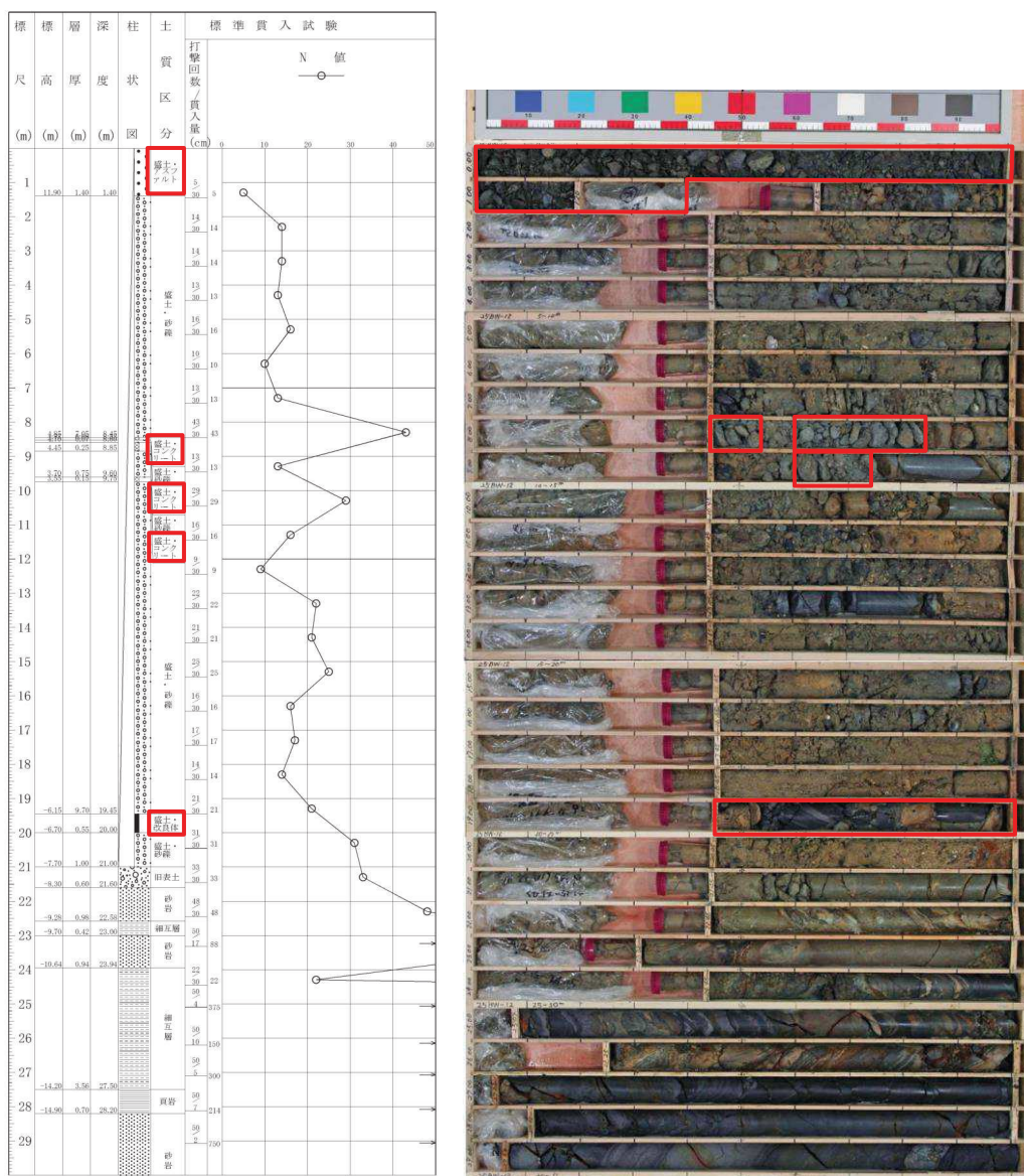
図 1. 1-13 ボーリング柱状図・コア写真 (25BW-12)
