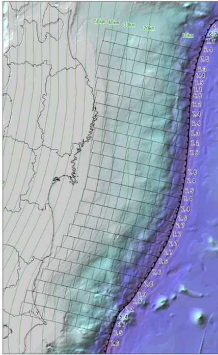
図1 津波波源モデル 25km×25km の小断層が走向方向に24、傾斜方向に8あり、合計192断層である。
