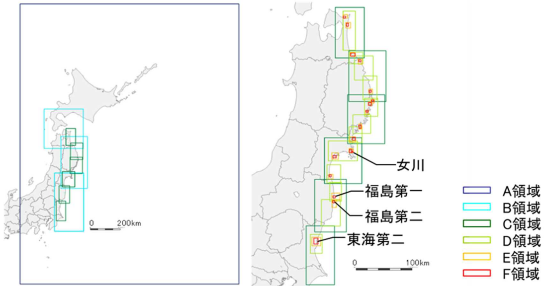
図2 検討対象領域の格子分割概念図(杉野他, 2014)
