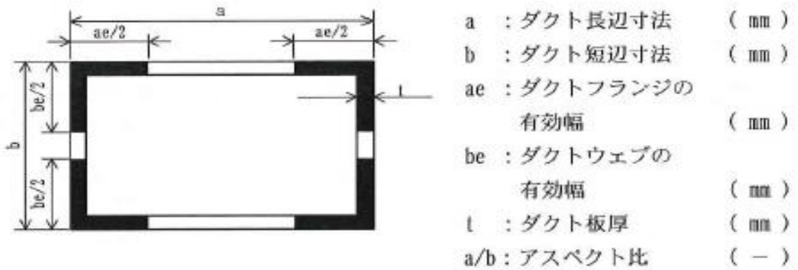
図2 ダクトの断面図
