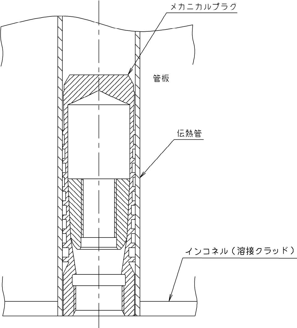
メカニカルプラグ取付図
