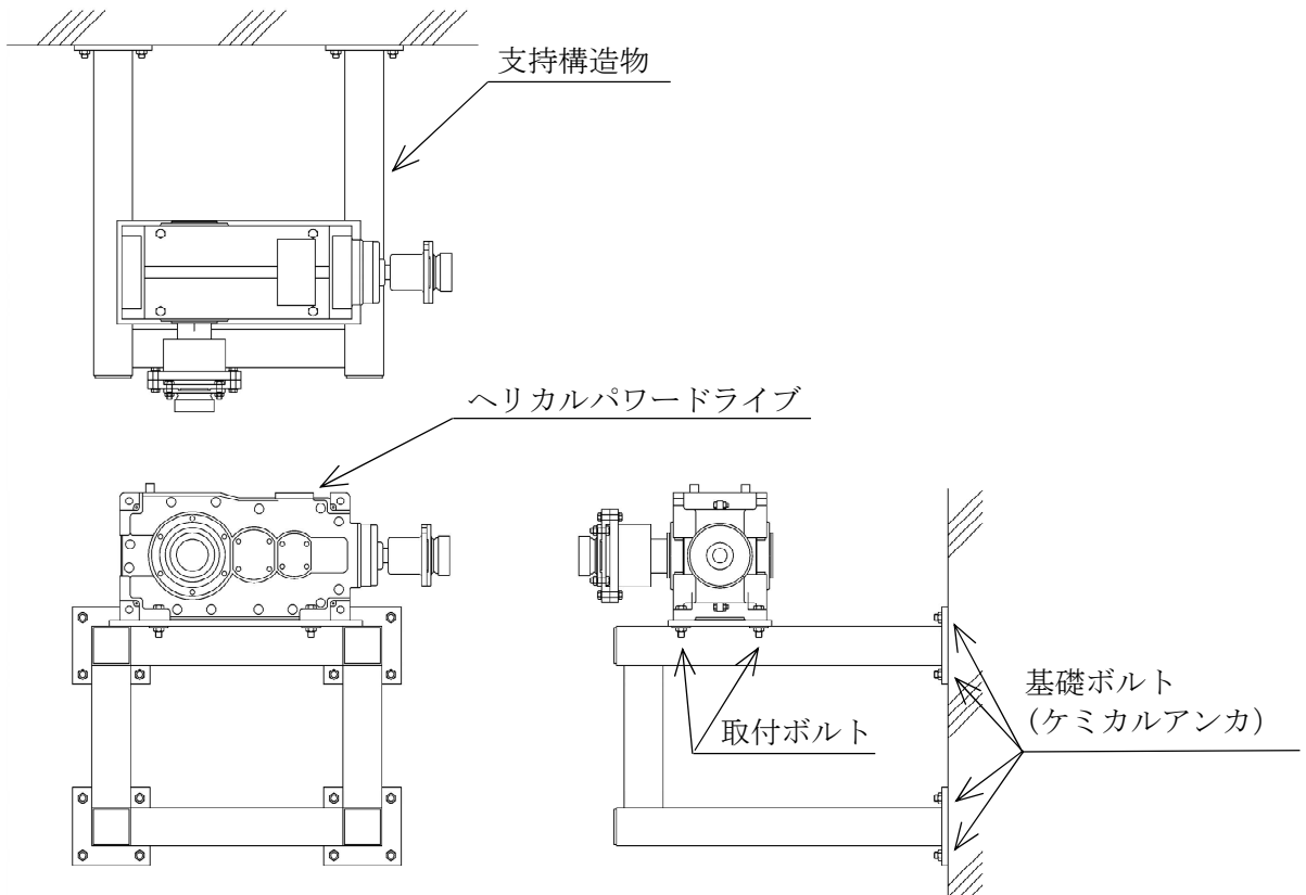
図 3-2 評価部位（遠隔手動弁操作設備（その 5）（支持構造物 A（取付ボルト，基礎ボルト）））
