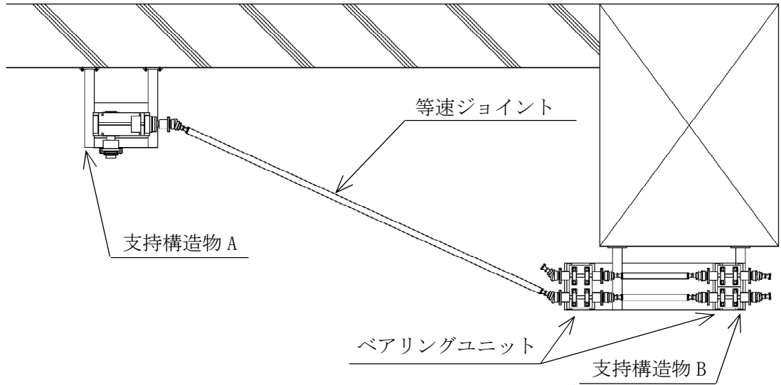
図 3-1 評価部位（遠隔手動弁操作設備（その 5）（等速ジョイント））
