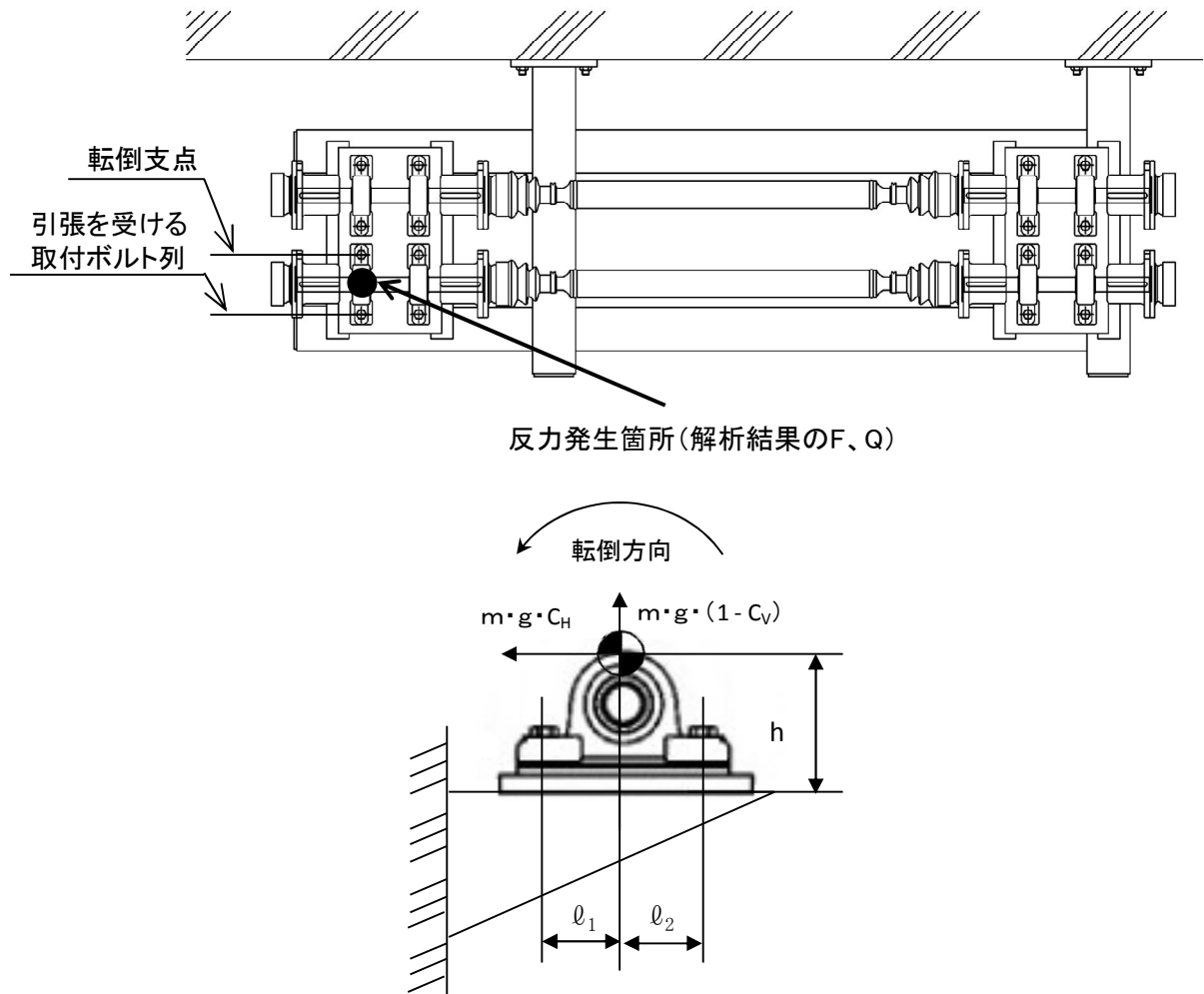
図 4-6 計算モデル
