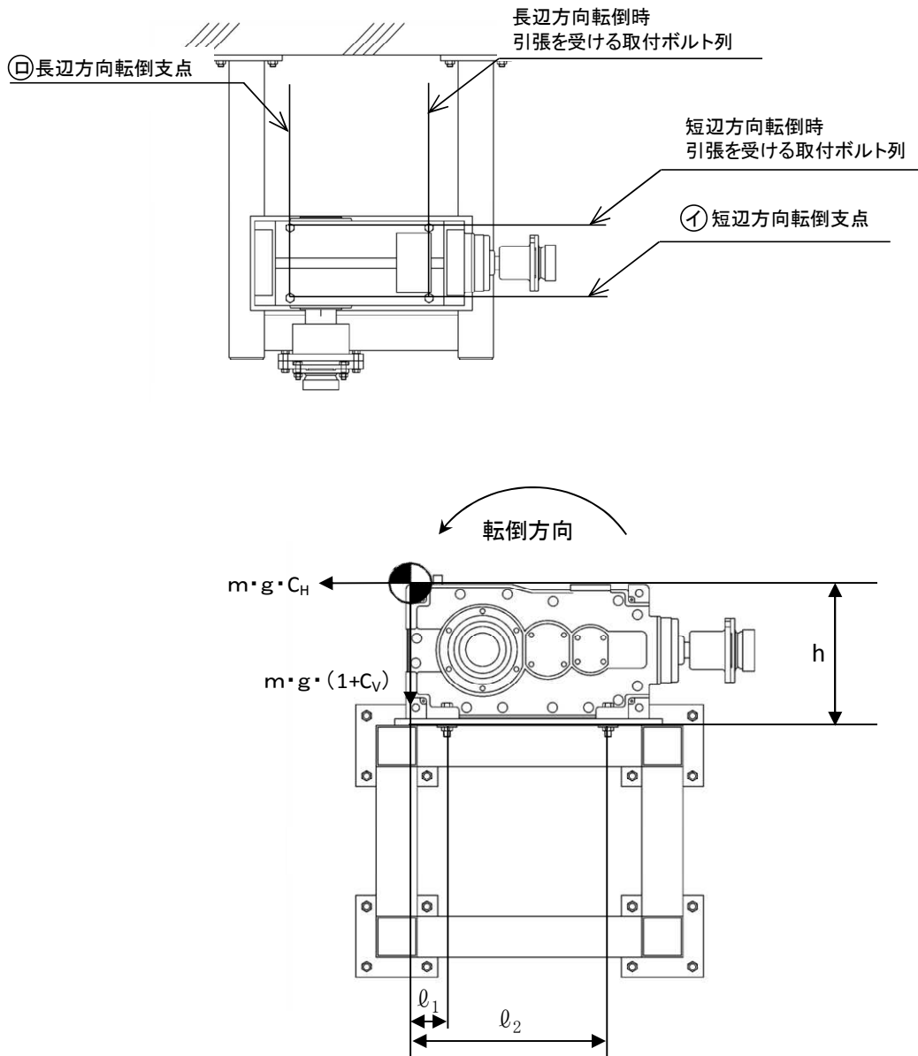
図 4-4 計算モデル（長辺方向転倒の場合）
