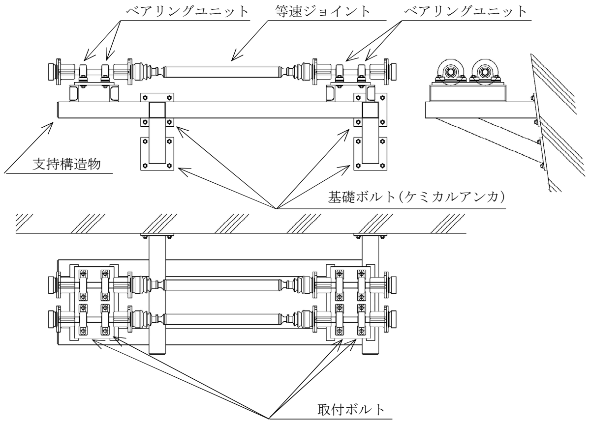
図 3-3 評価部位 (遠隔手動弁操作設備 (その 5) (支持構造物 B (取付ボルト, 基礎ボルト)))
