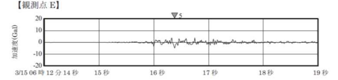
4号機爆発と推定される時刻の加速度波形(南北方向)
