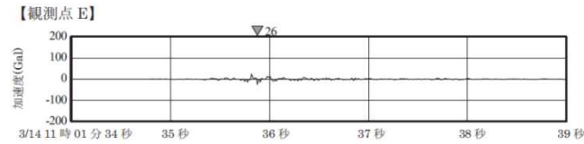
3号機爆発時の加速度波形(南北方向)
