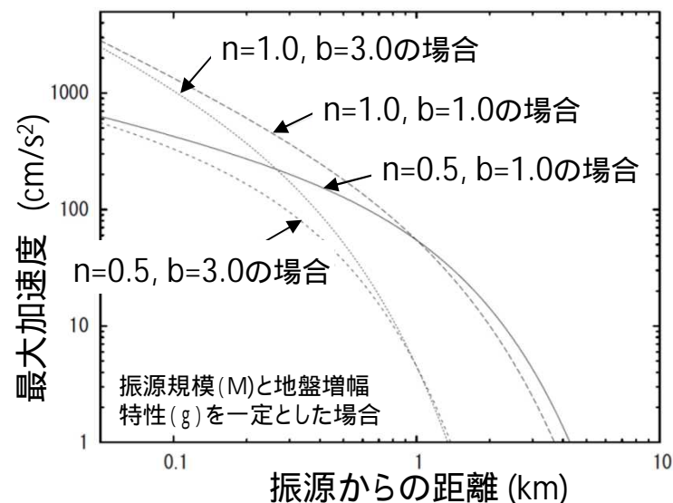
距離減衰特性の例
