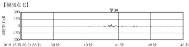
1号機爆発時の加速度波形(南北方向)
