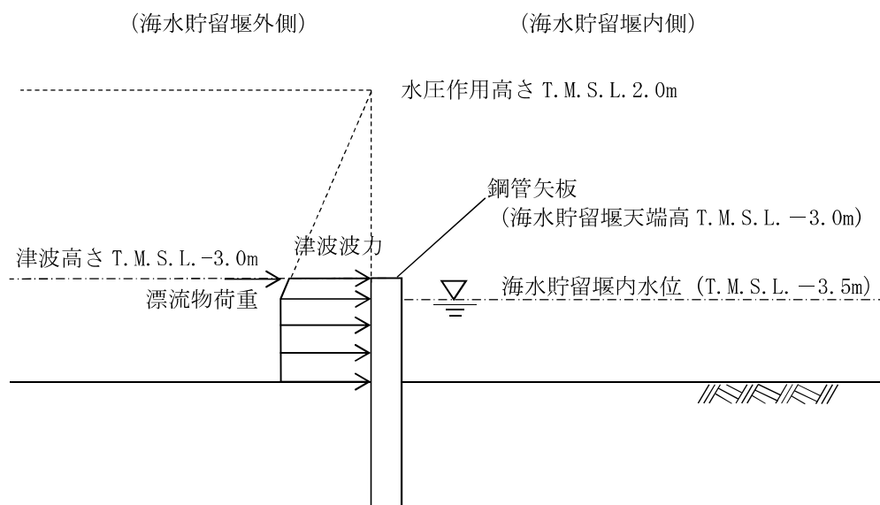
図 2.4-3-4 荷重作用図（鋼管矢板 津波時 北側）
