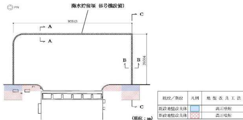
(a) 海水貯留堰の平面図
