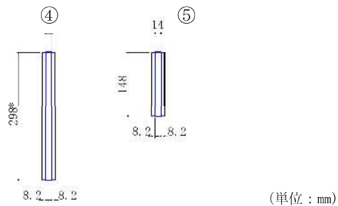
図2.4-3-19 照査モデル図（前面鋼矢板及び鋼管矢板との接合部）
