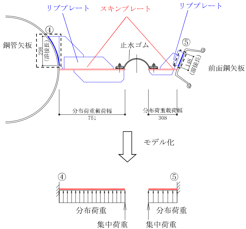
図2.4-3-19 照査モデル図（前面鋼矢板及び鋼管矢板との接合部）
