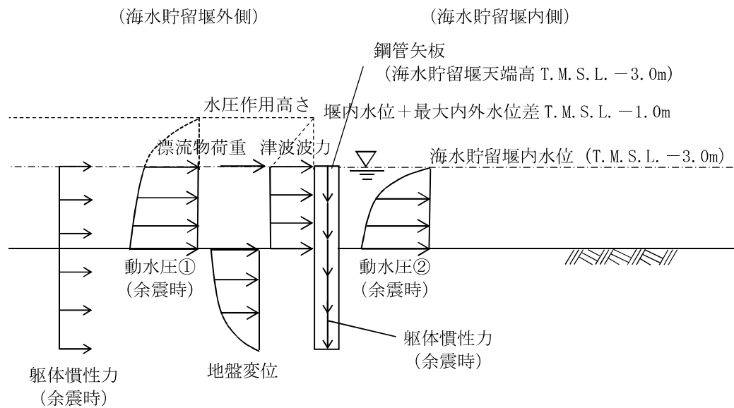
図 2.4-3-6 荷重作用図（鋼管矢板 重畳時 2 北側）
