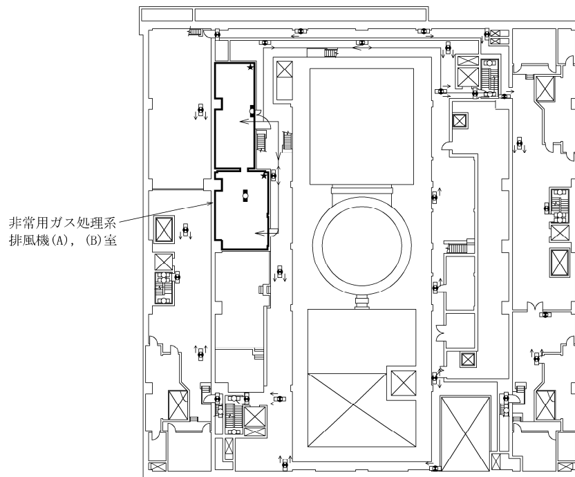
7号機原子炉建屋 T.M.S.L. 23500
