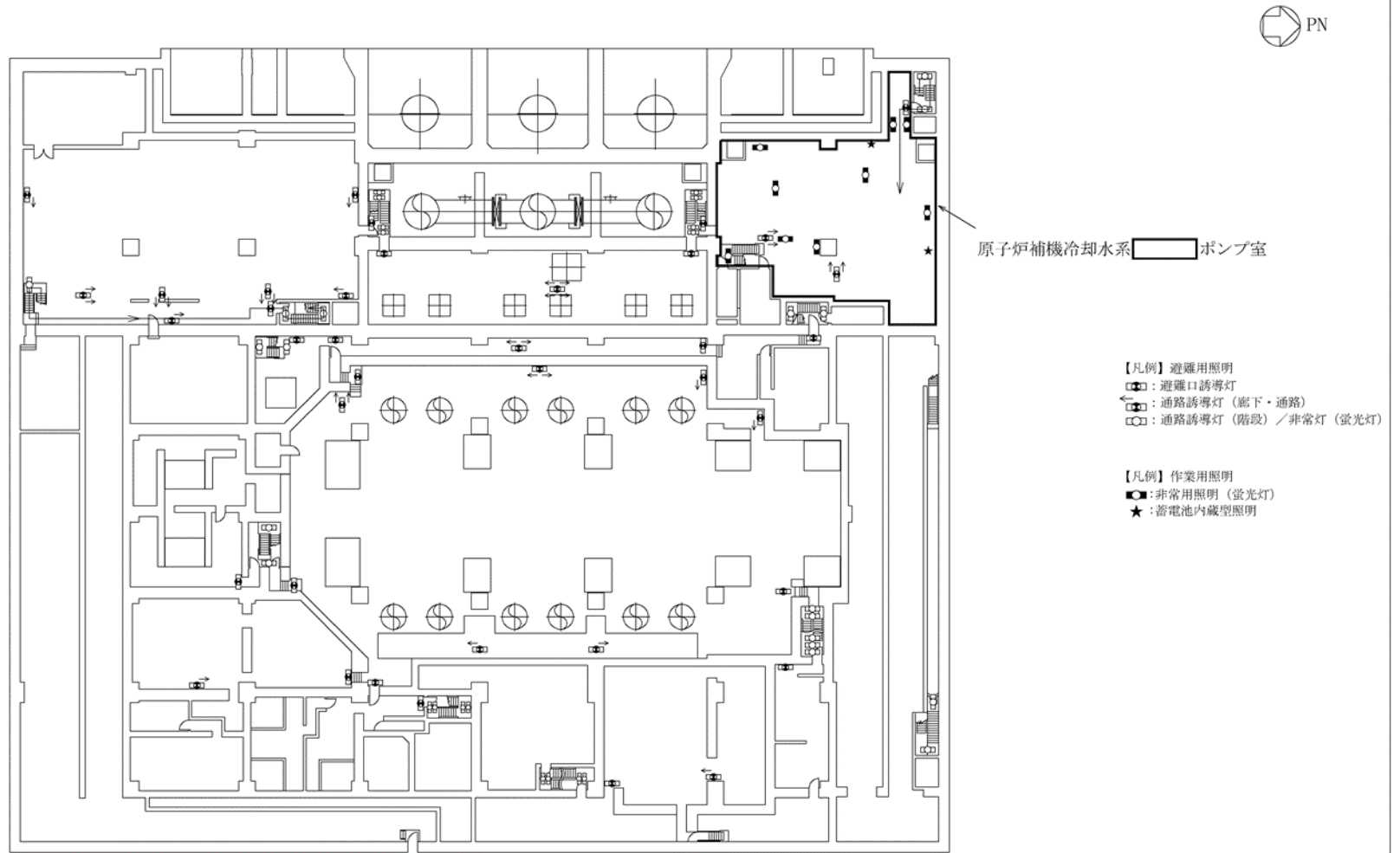
7号機タービン建屋 T.M.S.L. -5100
