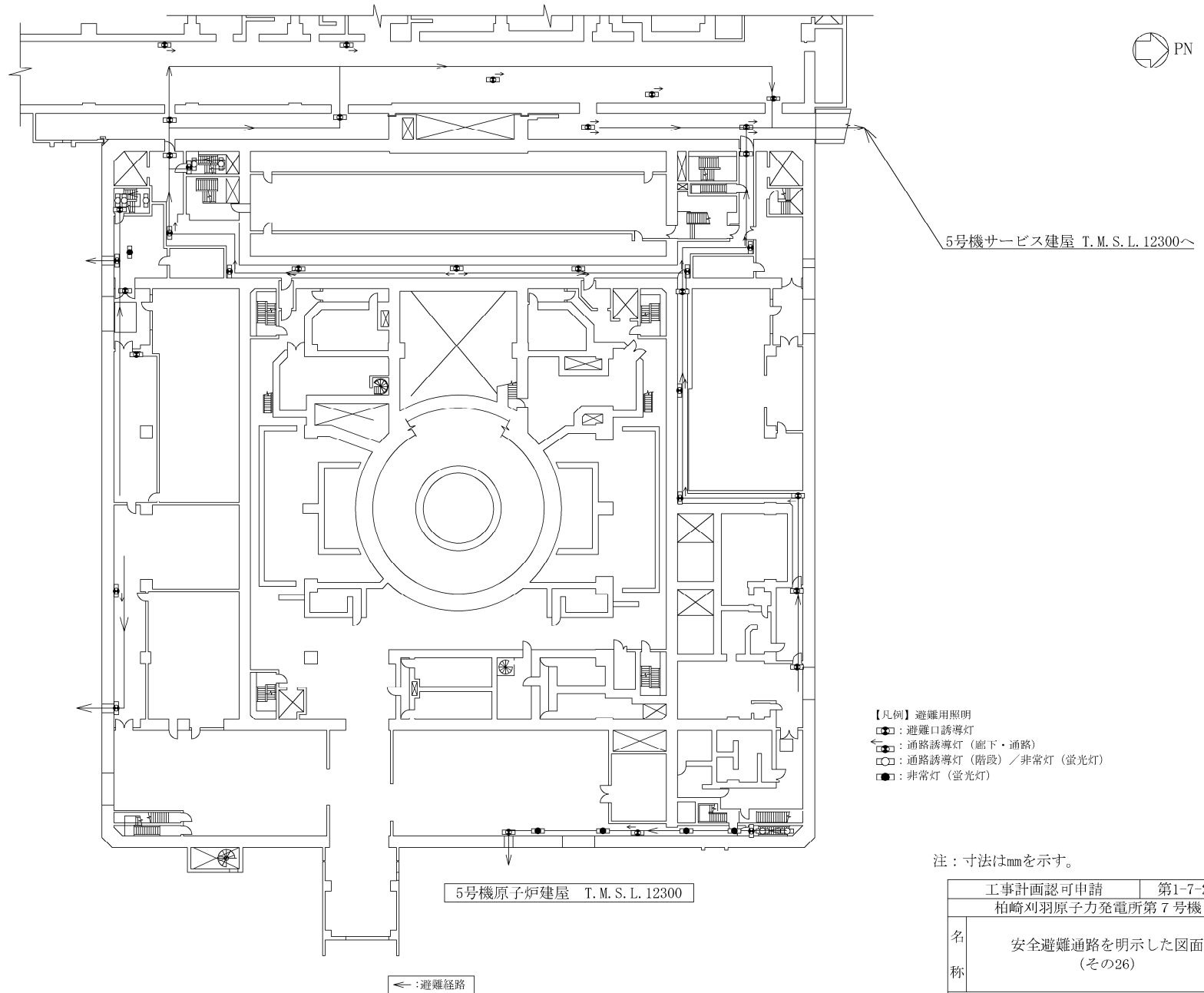
図1 避難経路を明示した図面 26
