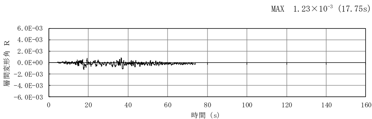
図3-9 層間変形角の時刻歴波形 (A-A断面, Ss-3--) (検討ケース①：基本ケース)
