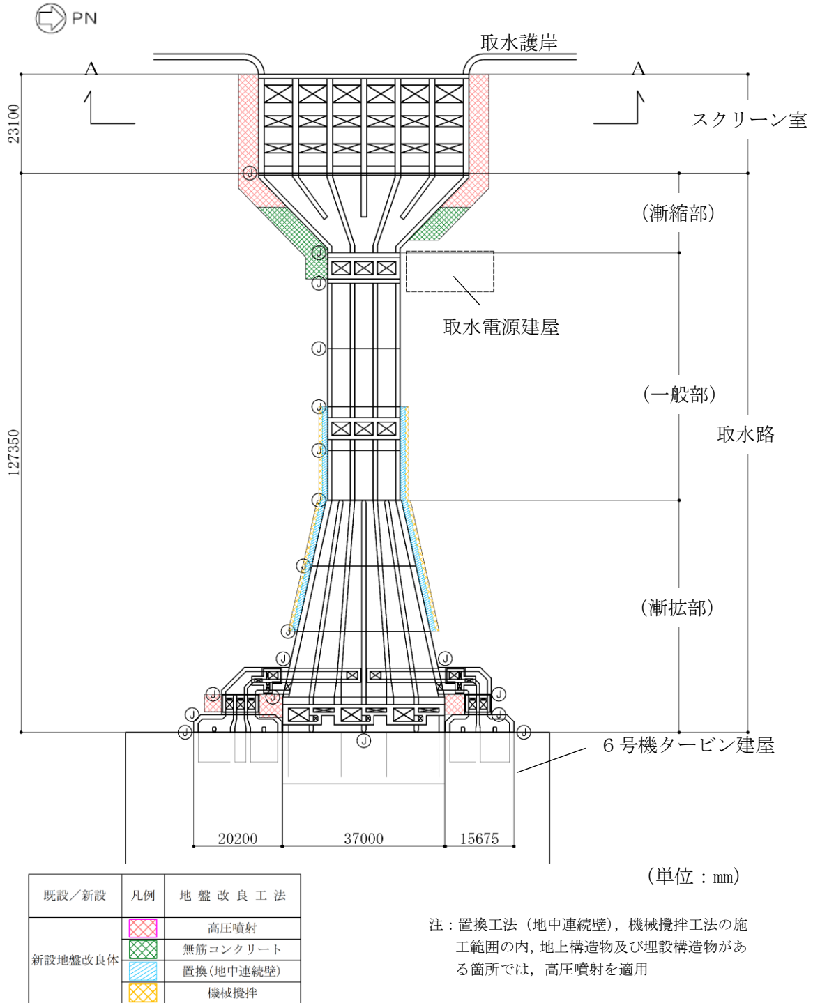
図3-1 スクリーン室（6号機設備）の評価対象断面位置図
