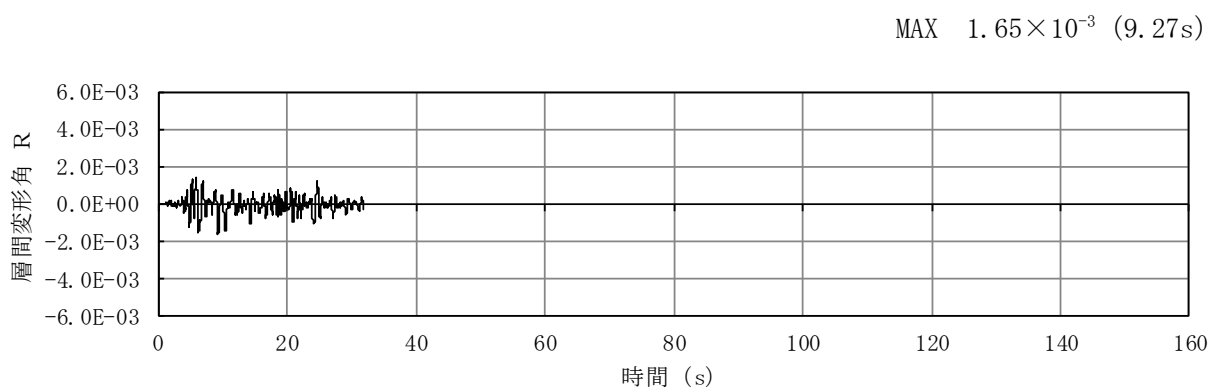
図3-9 層間変形角の時刻歴波形 (A-A断面, Ss-1-+) (検討ケース①: 基本ケース)
