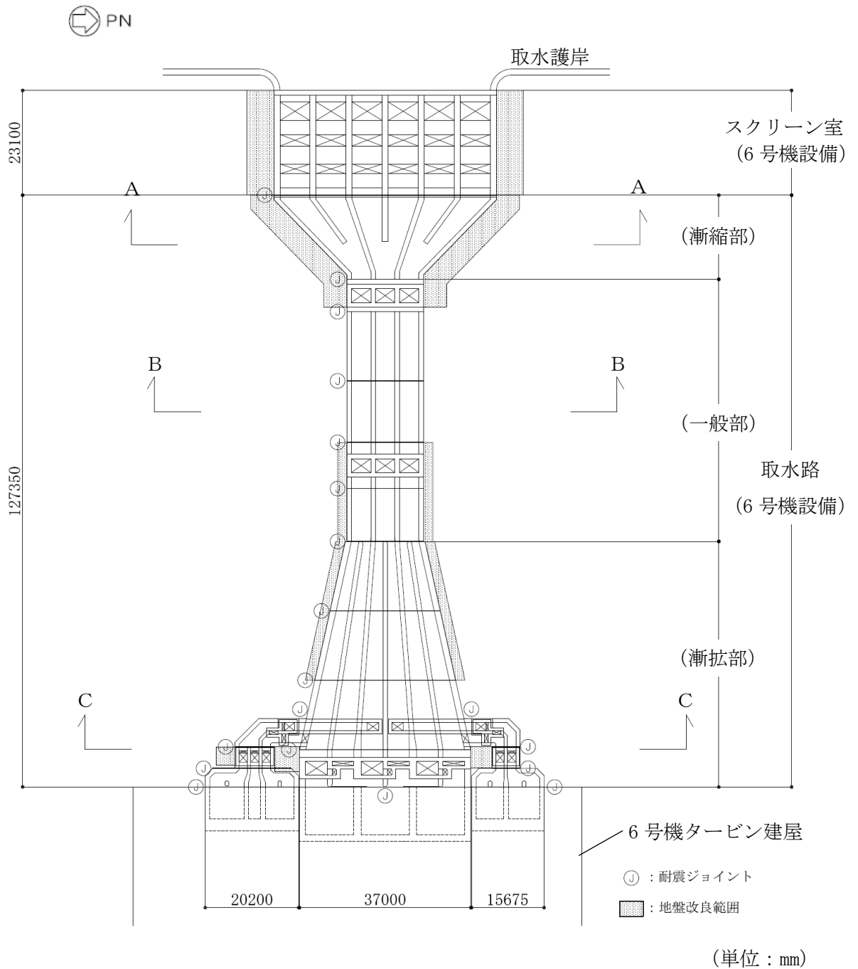
図2-2 取水路（6号機設備）の平面図
