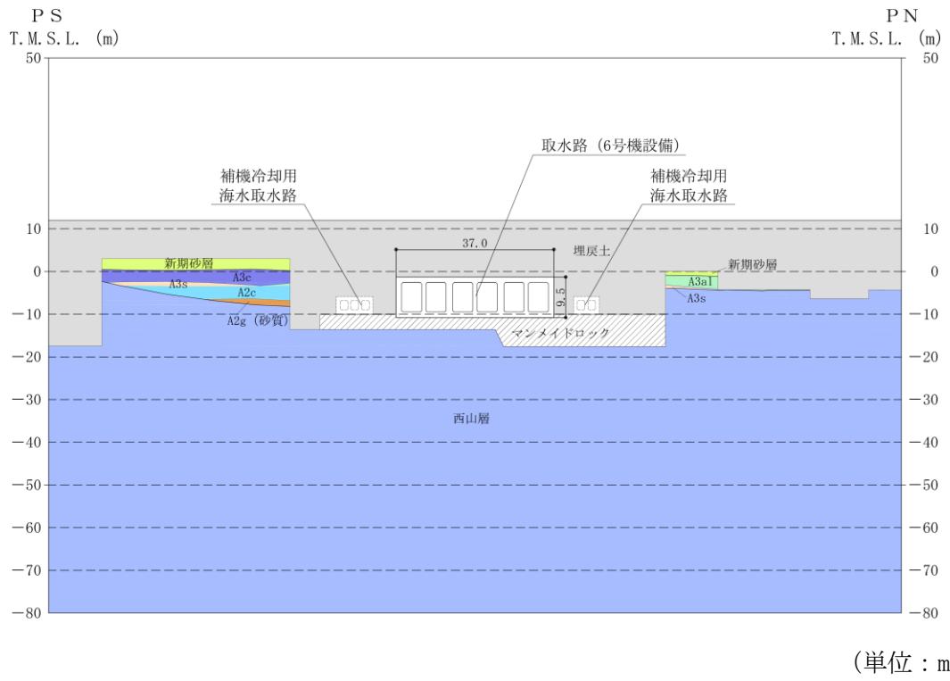
図 3-2 (3) 取水路 (6号機設備) の評価対象断面図 (C-C断面)
