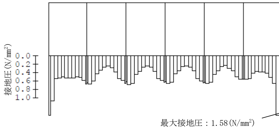
図3-10 C-C断面の最大接地圧分布図 (解析ケース②, 地震動 Ss-1-+)
