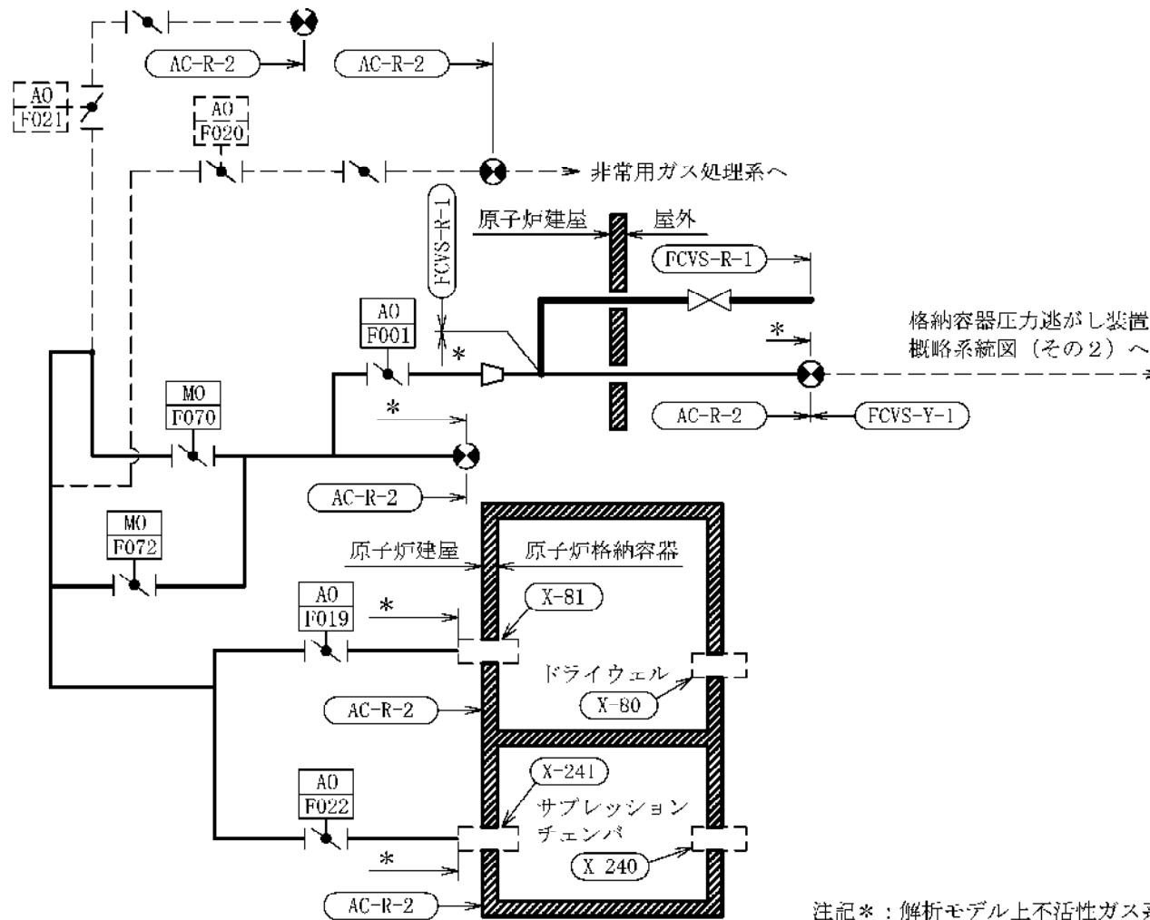
格納容器圧力逃がし装置概略系統図 (その1)
