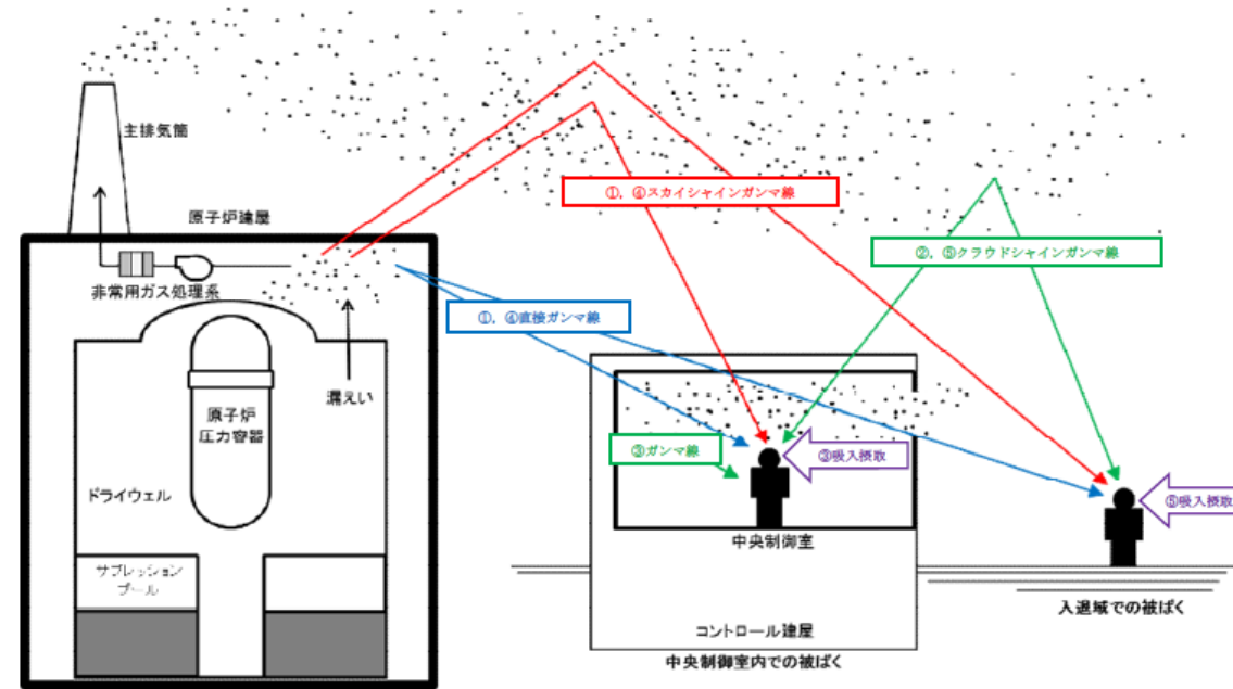
図4-6 中央制御室の居住性に係る被ばく経路イメージ (1/3) (原子炉冷却材喪失)
