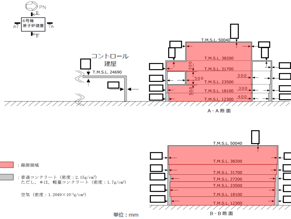
図4-19 建屋内の放射性物質からのガンマ線による被ばく評価モデル (3/5) (原子炉冷却材喪失時の直接ガンマ線評価モデル) (6号機)
