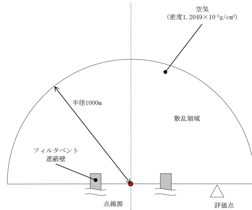
散乱計算モデル (G33-GR2Rコードの計算モデル)
