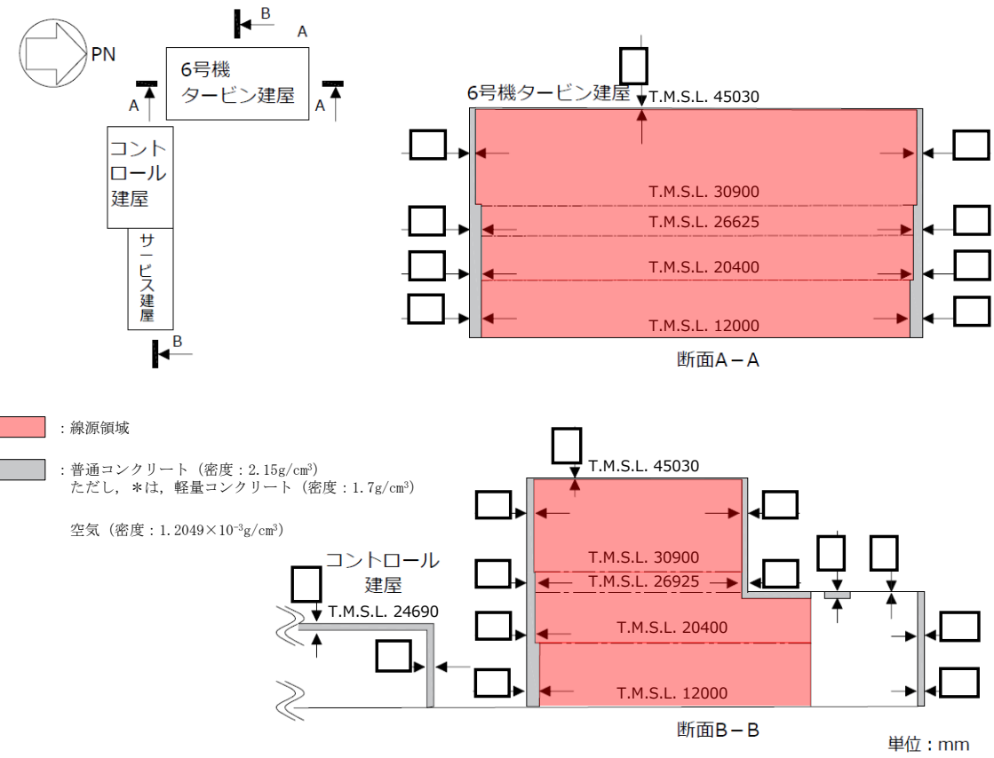
図4-21 主蒸気管破断時の評価モデル (3/5) (直接ガンマ線) (6号機)
