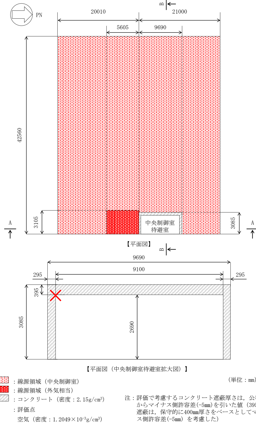
図 4-42 評価モデル (隣接エリア内の放射性物質からのガンマ線) (1/3)
