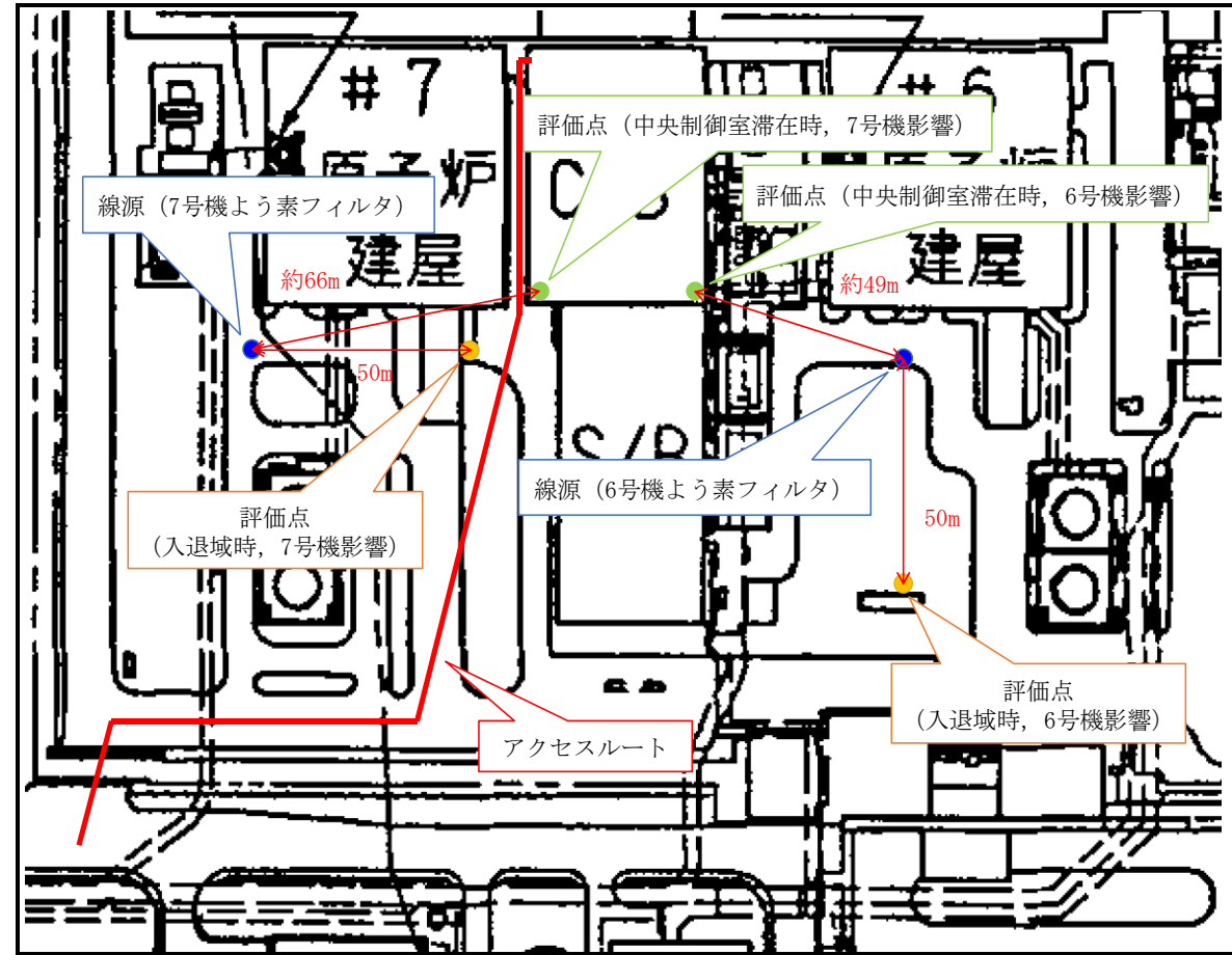
図 4-39 アクセスルート並びに線源及び評価点の位置 (中央制御室滞在時及び入退域時) (距離は、フィルタベント建屋中心から評価点までの距離を示す)
