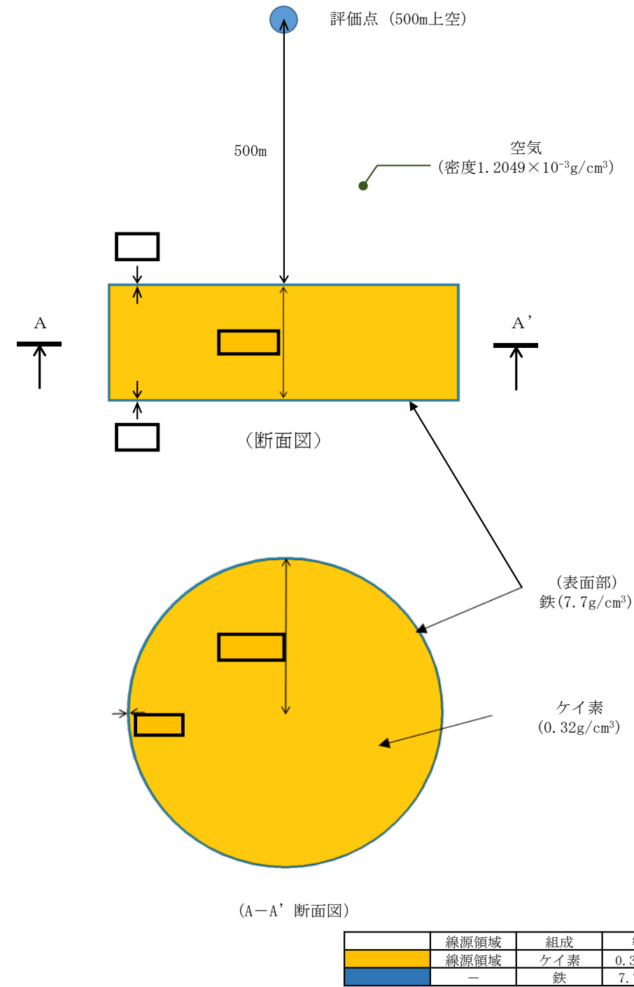
図 4-36 体積線源モデル図 (よう素フィルタ)
