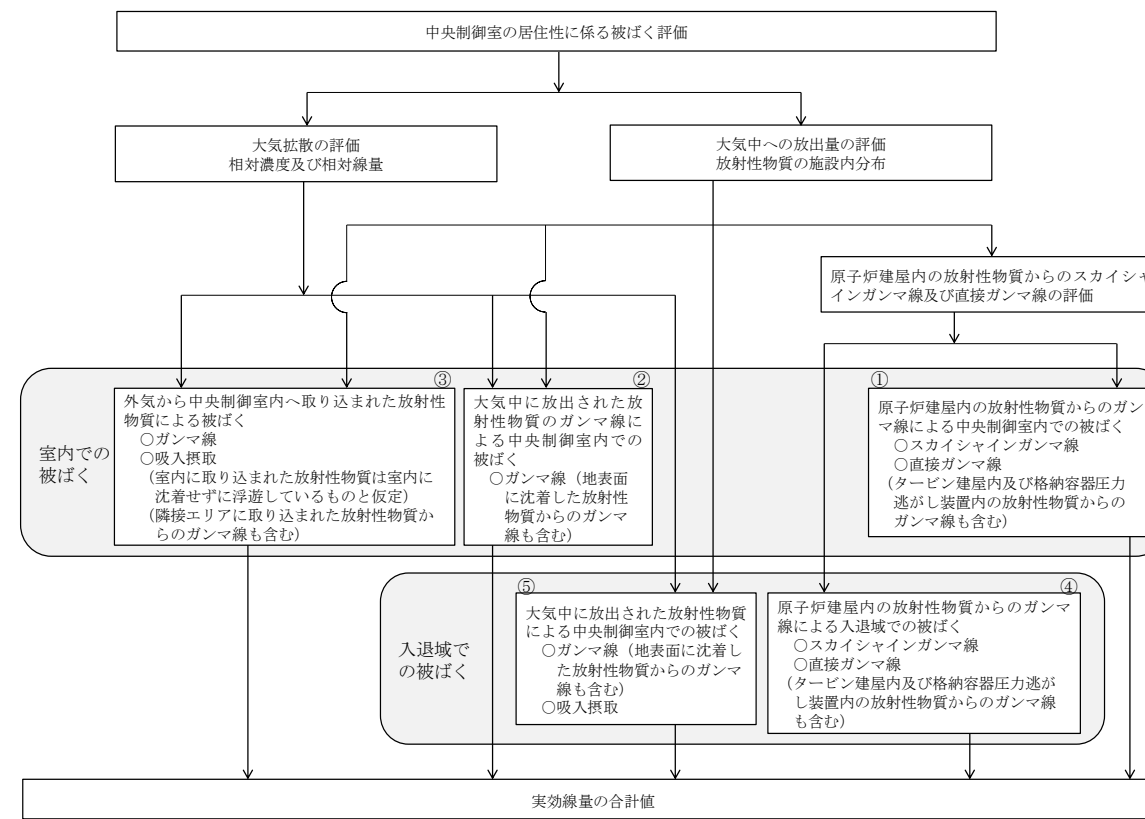
図4-5 中央制御室の運転員の被ばく経路
