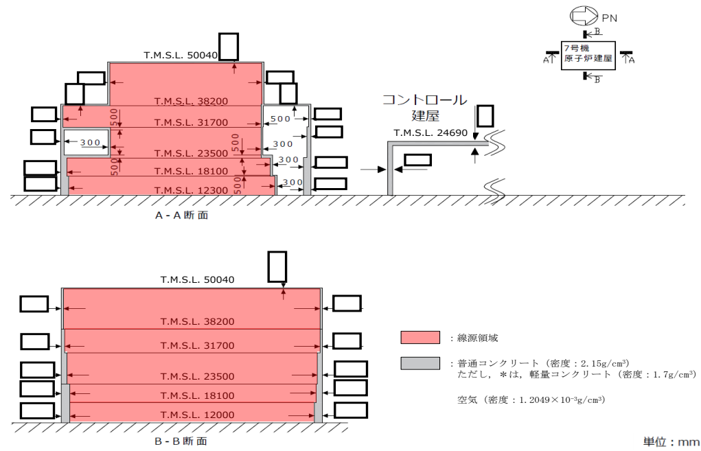
図4-19 建屋内の放射性物質からのガンマ線による被ばく評価モデル (4/5) (原子炉冷却材喪失時の直接ガンマ線評価モデル) (7号機)
