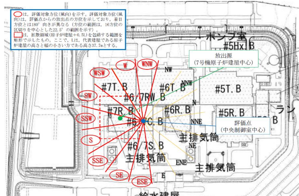
図4-14 原子炉建屋漏えい時の評価風向 (評価点：中央制御室中心) (炉心の著しい損傷が発生した場合) (2/2) (7号機)
