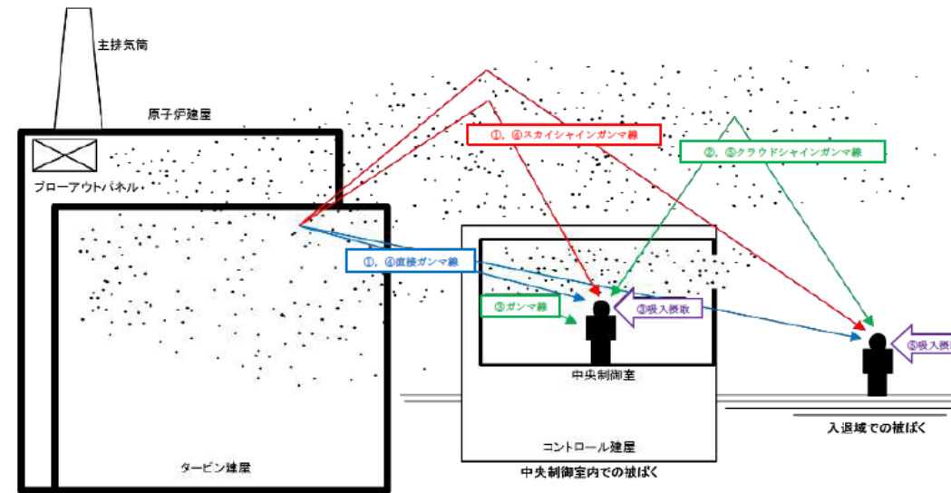
図4-6 中央制御室の居住性に係る被ばく経路イメージ (2/3) (主蒸気管破断)
