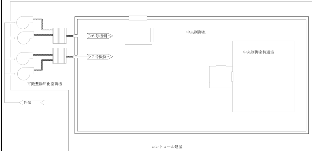
図4-3 換気設備の系統図 (2/2) (中央制御室可搬型陽圧化空調機)
