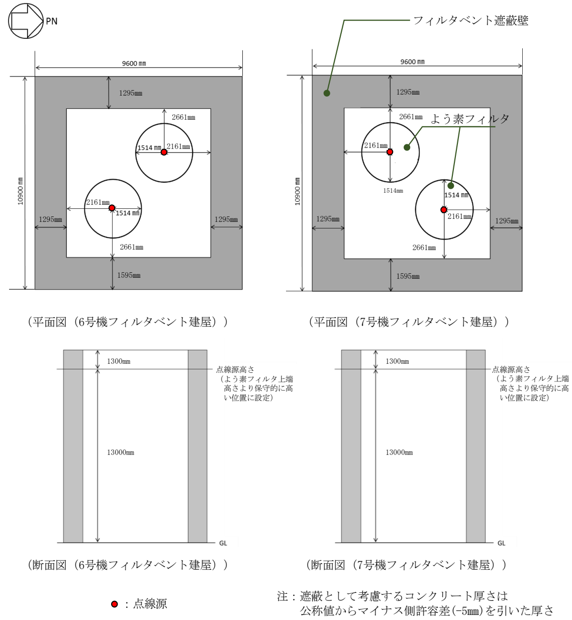
図 4-38 よう素フィルタからのスカイシャインガンマ線の評価モデル (よう素フィルタとフィルタベント遮蔽壁の位置関係)
