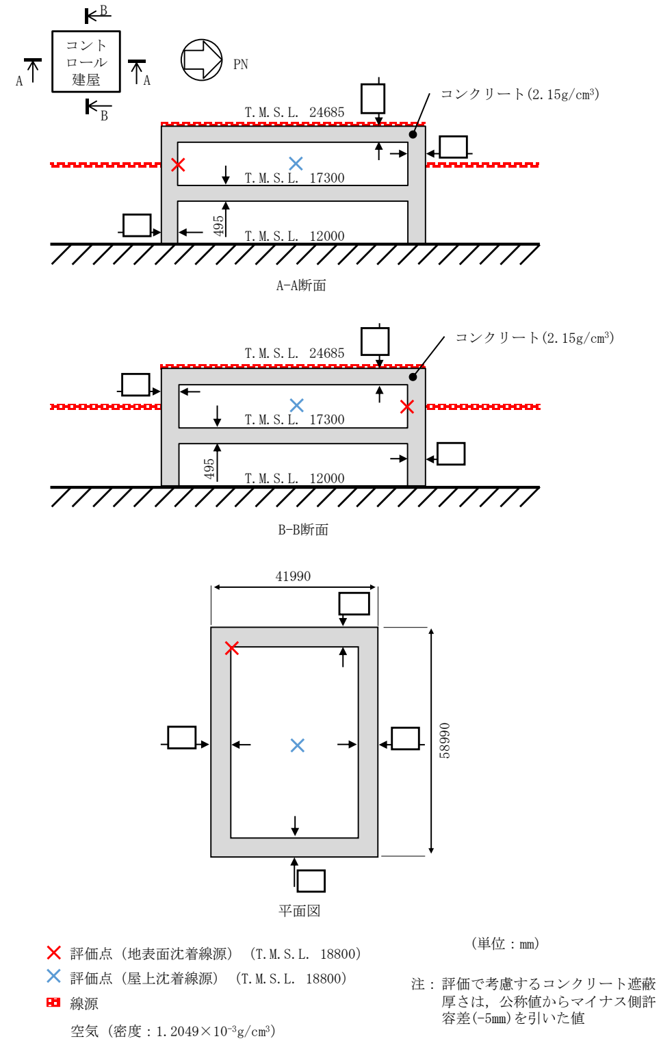
図4-41 中央制御室内被ばく評価時のグラウンドシャイン評価モデル(2/2)
