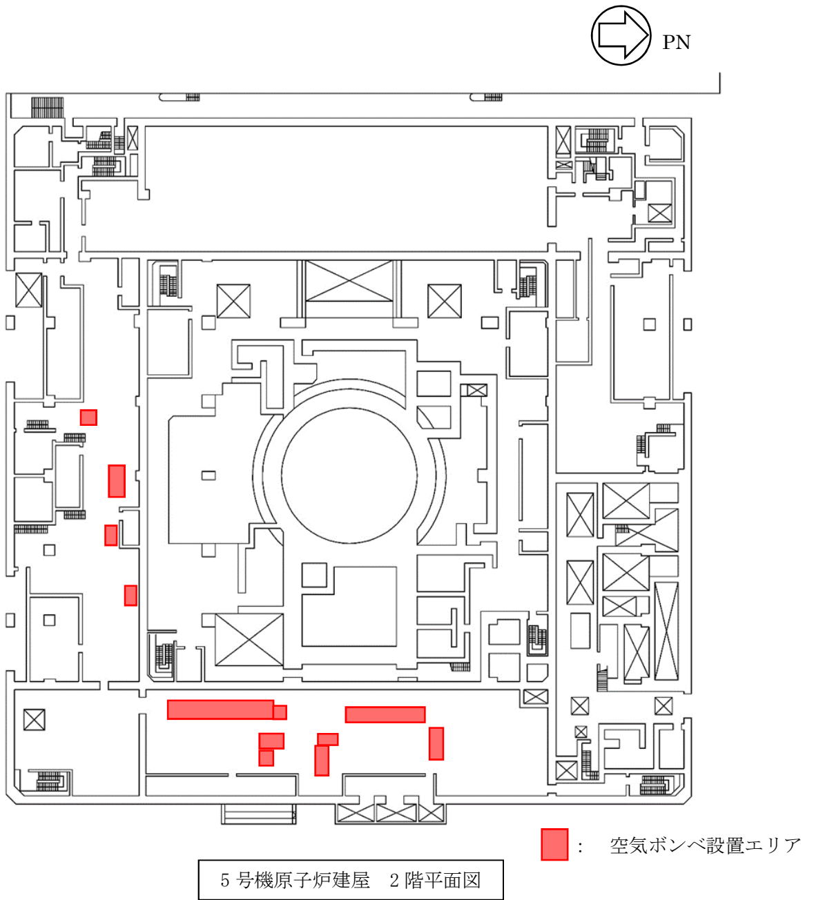
図 3-2 緊急時対策所機器配置図 (2/3)
