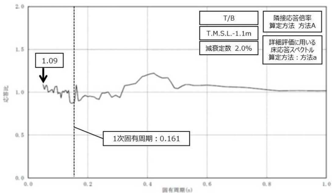
図添2-9 隣接応答倍率の算定 (RCW-T-5)
