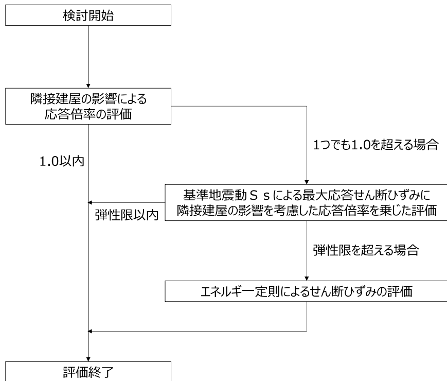
(a) 耐震壁
