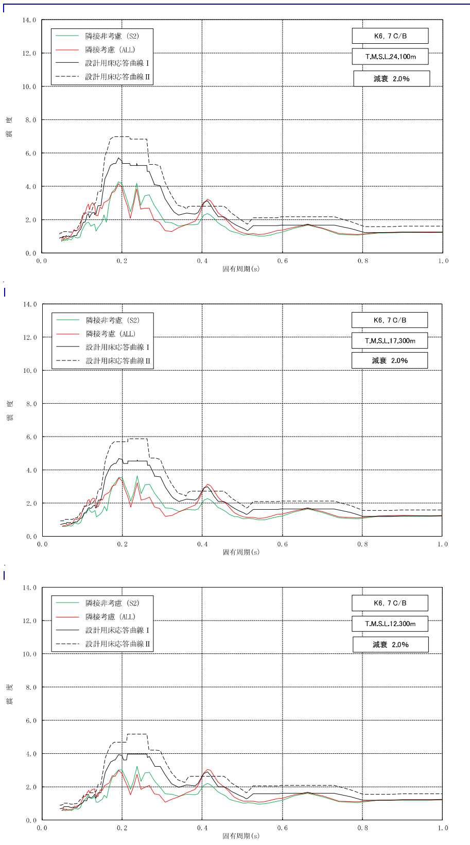
図添 1-2 床応答スペクトルの比較 (コントロール建屋, 水平方向, 減衰 2.0%) (1/2)
