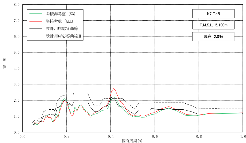
図添 1-3 床応答スペクトルの比較 (7号機タービン建屋, 水平方向, 減衰 2.0%) (3/3) 別紙 4-17
