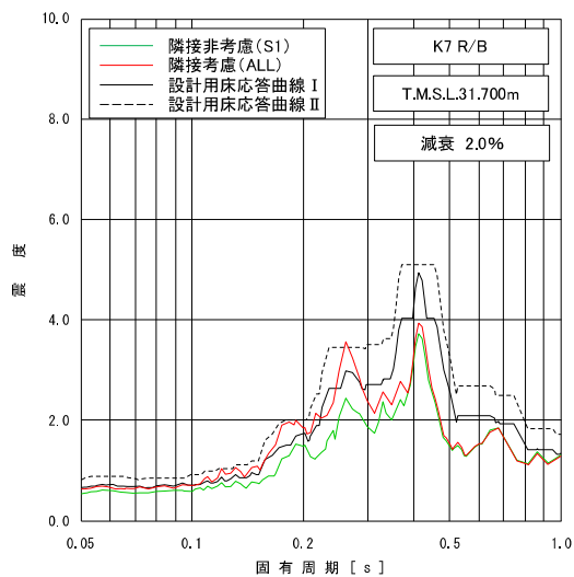
図添 1-1 床応答スペクトルの比較 (7号機原子炉建屋, 水平方向, 減衰 2.0%) (1/3)
