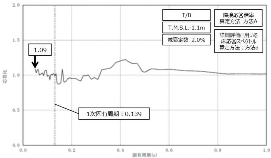
図添2-7 隣接応答倍率の算定 (RCW-T-1)
