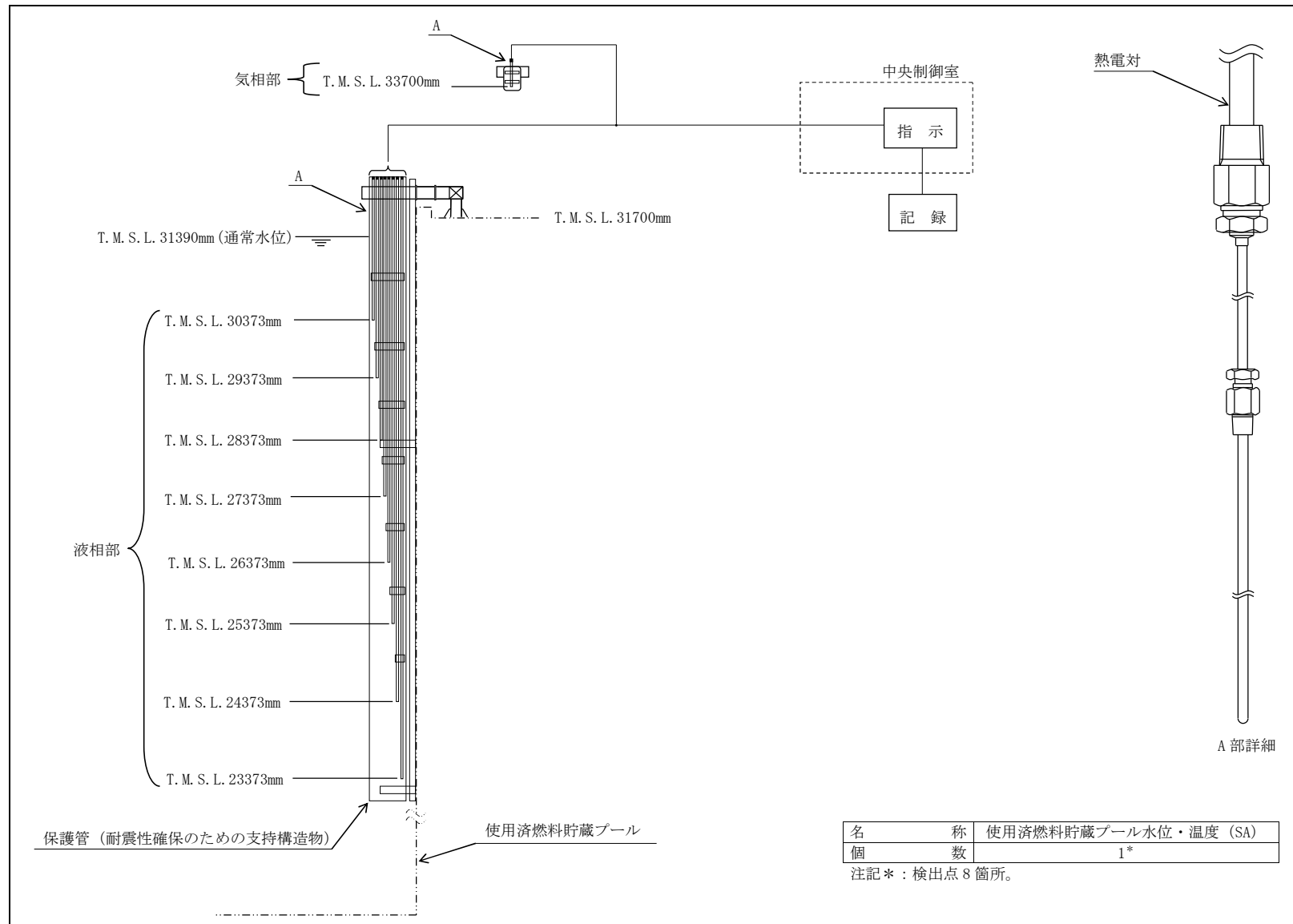
図 3-7 使用済燃料貯蔵プール水位・温度 (SA) の構造図
