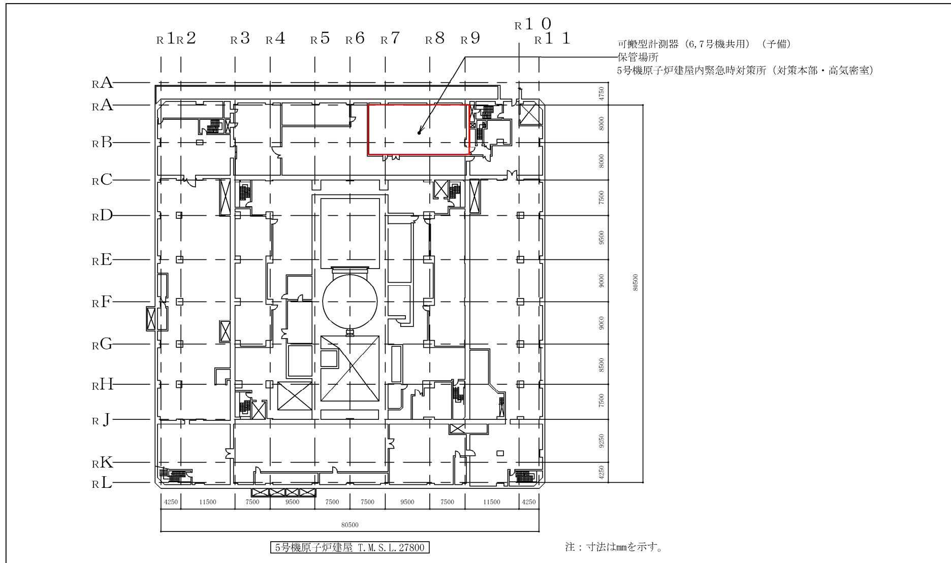
図 3-19 可搬型計測器 (6, 7号機共用) (予備) の保管場所を明示した図面
