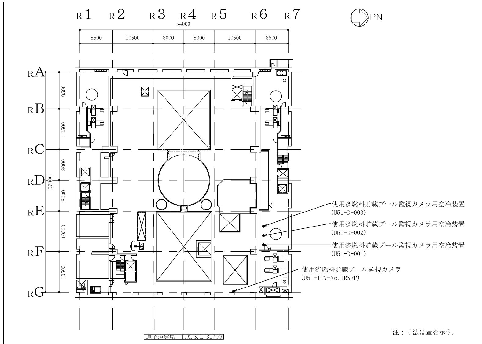
図 3-13 使用済燃料貯蔵プール監視カメラ及び使用済燃料貯蔵プール監視カメラ用空冷装置の取付箇所を明示した図面
