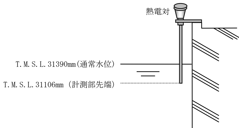
図 4-1 使用済燃料貯蔵プール温度の設置図
