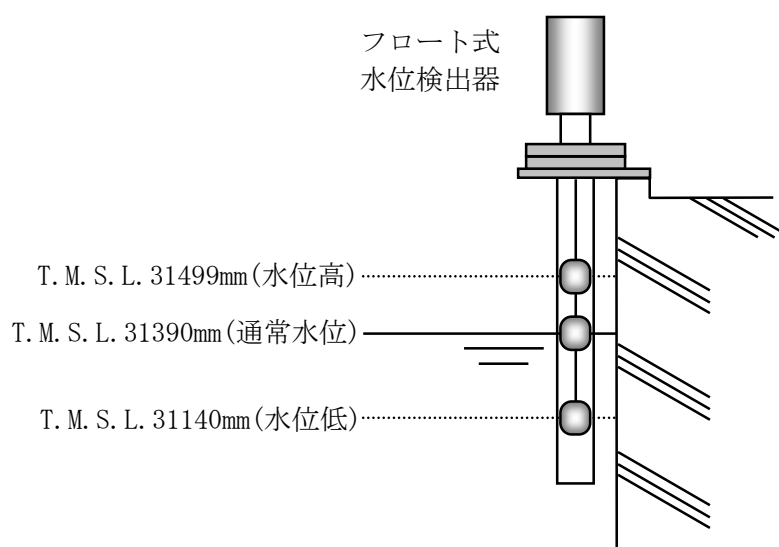
図 4-3 使用済燃料貯蔵プール水位の設置図
