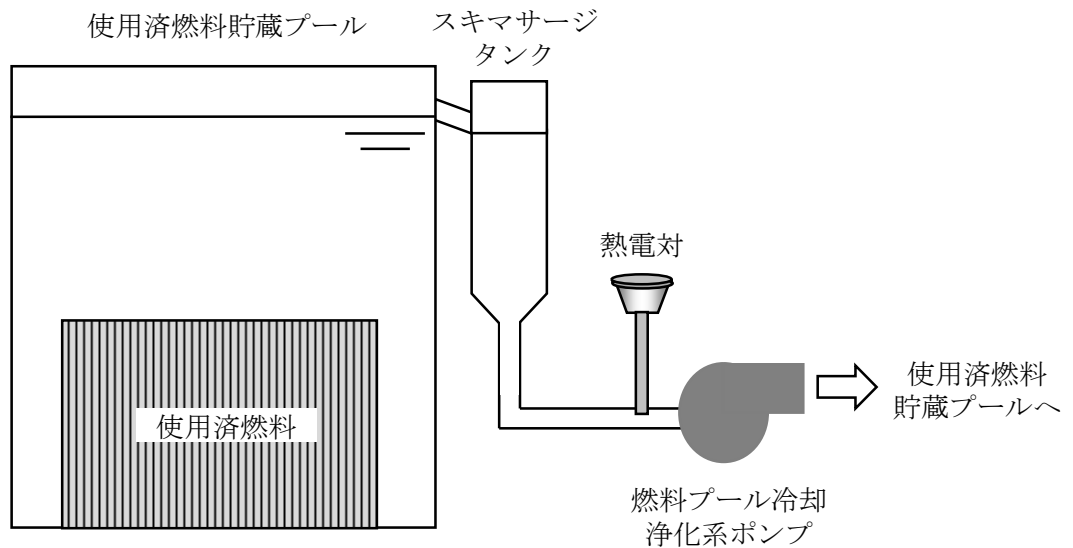
図4-2 燃料プール冷却浄化系ポンプ入口温度の設置図
