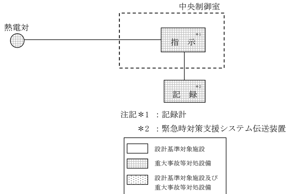
図3-6 使用済燃料貯蔵プール温度（SA）の概略構成図
